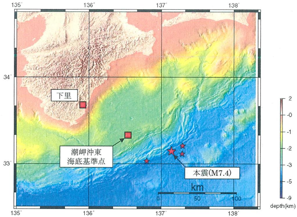
図1：潮岬沖東海底基準点、および紀伊半島南東沖地震の震源（星印はM6.0以上の震央）
