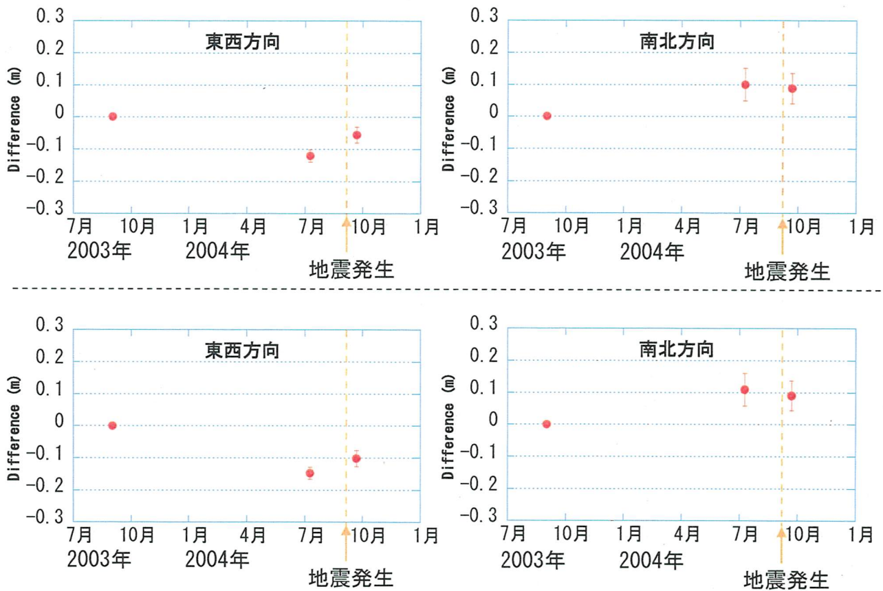
図2：潮岬沖東海底基準点の位置変化（2003年9月～2004年9月）
