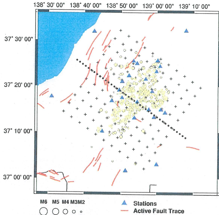
左図. 使用したグリッド配置、観測点分布、求めた震源の震央分布を示す。点線は上図の断面図の位置を示す。
