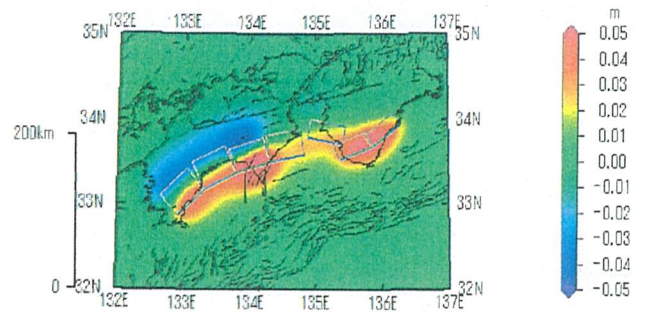
断層モデルによる地表の理論上下変動(橋本)
