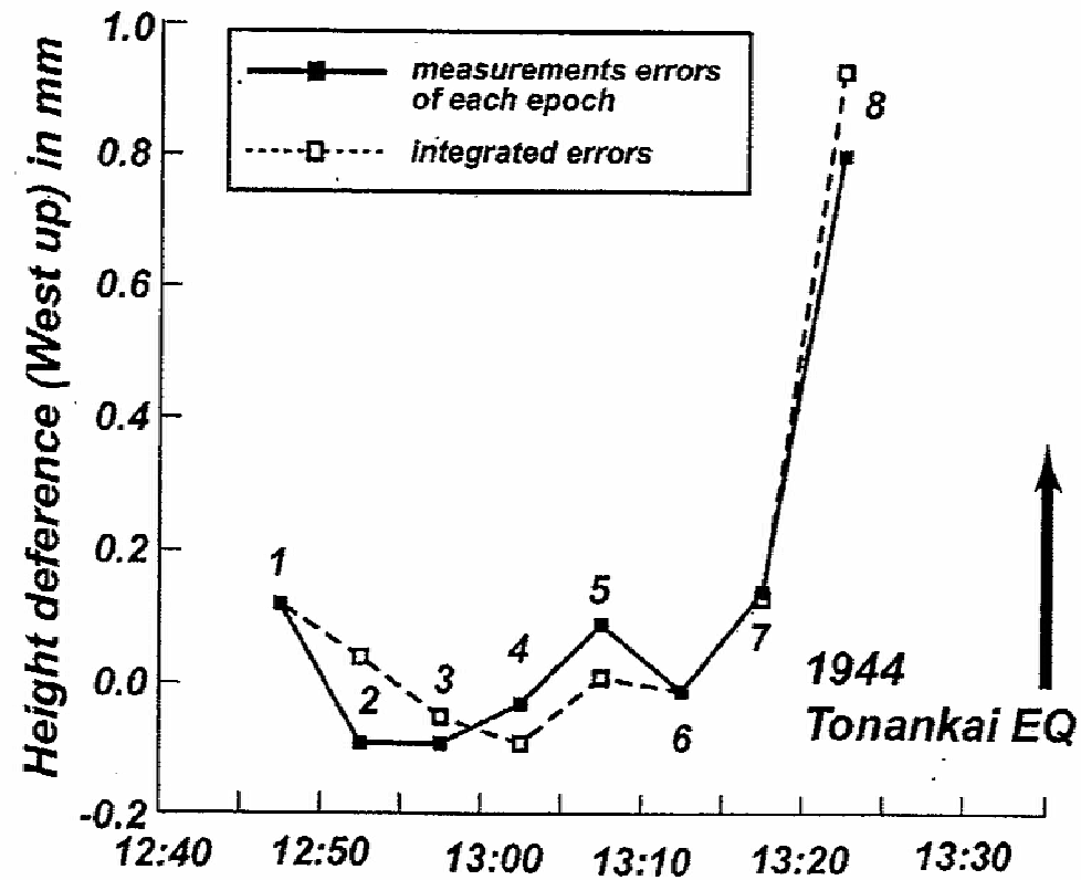
図2 水準作業区間31(D)における測量ごとの誤差と水準儀不安定から推定される上下変動量。 ■が各回ごとの誤差、□が積算した誤差を示す。
