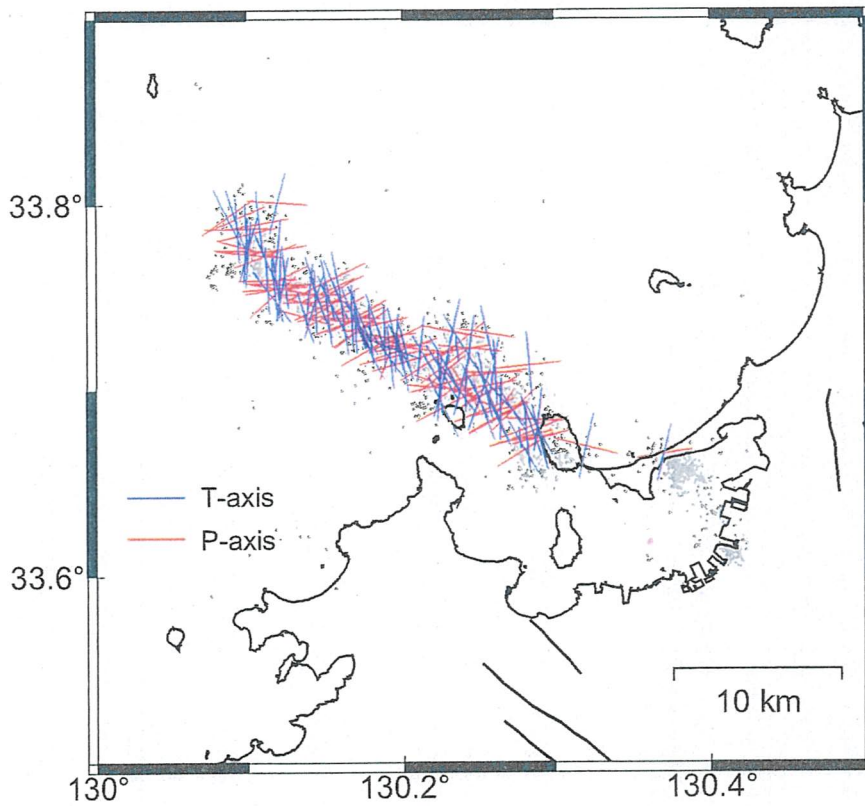
上図) 主な地震のメカニズム解. 橙色: Hi-netによる初動解. 水色: F-netによるMT解. 赤点はHi-netにより求められた震央分布を表す.
