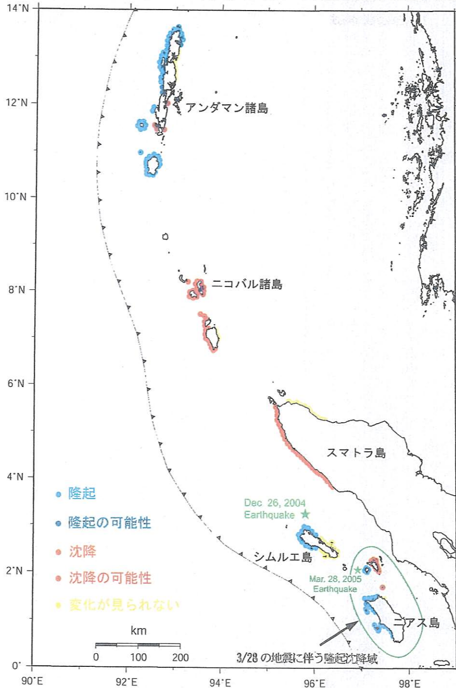
人工衛星画像解析によって判明した2004年(一部2005年)スマトラ島沖地震に伴う隆起・沈降域
