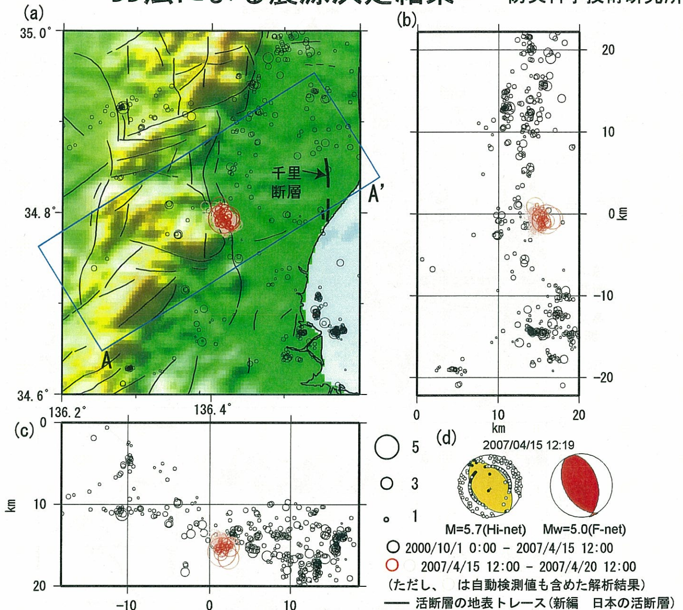
図1 防災科研Hi-netによる三重県北部の震源をDD法により再決定した震源分布を示す。(a)震央分布(深さ0~20km)、(b)南北断面に投影した震源深さ分布、(c)東西断面に投影した震源深さ分布、(d)本震の初動メカニズム解およびMT解。
