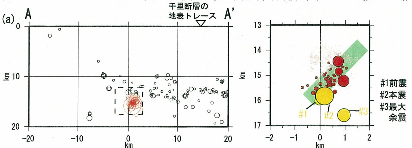
図2 (a)本震MT解節面走向(N148°E)に直交する断面(図1(a)のA-A')に投影した震源深さ分布、(b)余震域の拡大図(図2(a)の点線四角で囲まれた領域)。赤色は手動検測値を用いて決定した余震位置、薄い赤色は自動検測も含めて決定した余震位置を示す。(b)においてオレンジ色は前震、本震および最大余震の震源位置を示す。緑色の線はMT解節面の傾斜方向(45°)を示す。
