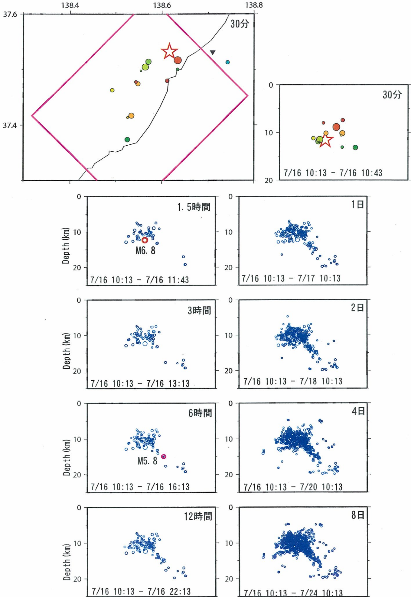
図5 hypoDD法で求めた震源の時間変化を南西方向から見た断面図
