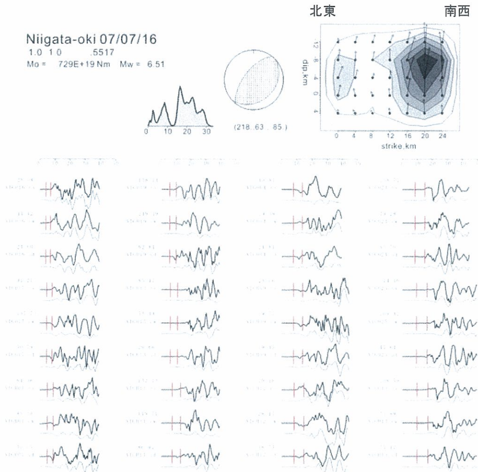
図 5 近地解析結果 波形の比較は上が観測波形，下が理論波形
