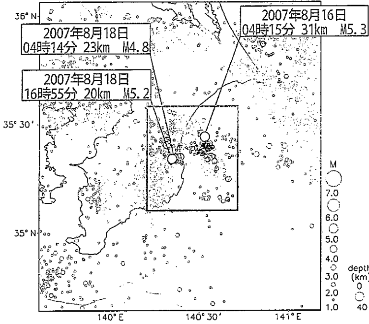
A 震央分布図（2002年1月以降、 M \geq 1.0 、深さ0~40km） 2007年8月1日以降を濃く表示
