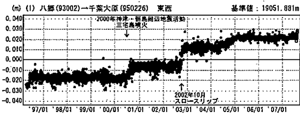
傾斜・半年周・年周補正グラフ (長期)
