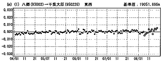
傾斜・半年周・年周補正グラフ (短期)
