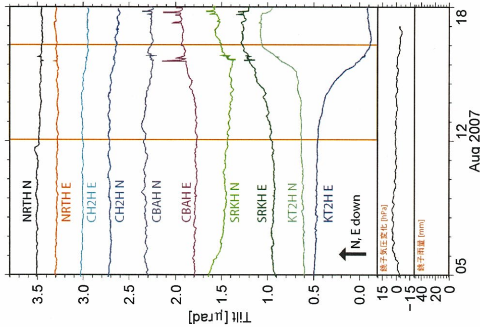
図2：2007年8月5日から19日までの2週間における傾斜時系列。観測点は、図1で示したものに白子（SRKH）を加えた。橙色で示した期間の前後における傾斜変化の差をデータとして断層モデルを推定した。この期間における気象庁銚子観測点の気圧変化および雨量をあわせて示す。
