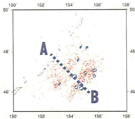
第3図。線分A-Bに投影した震央に対するETASモデルによる変換時間(第2図参照)の時空間図。
