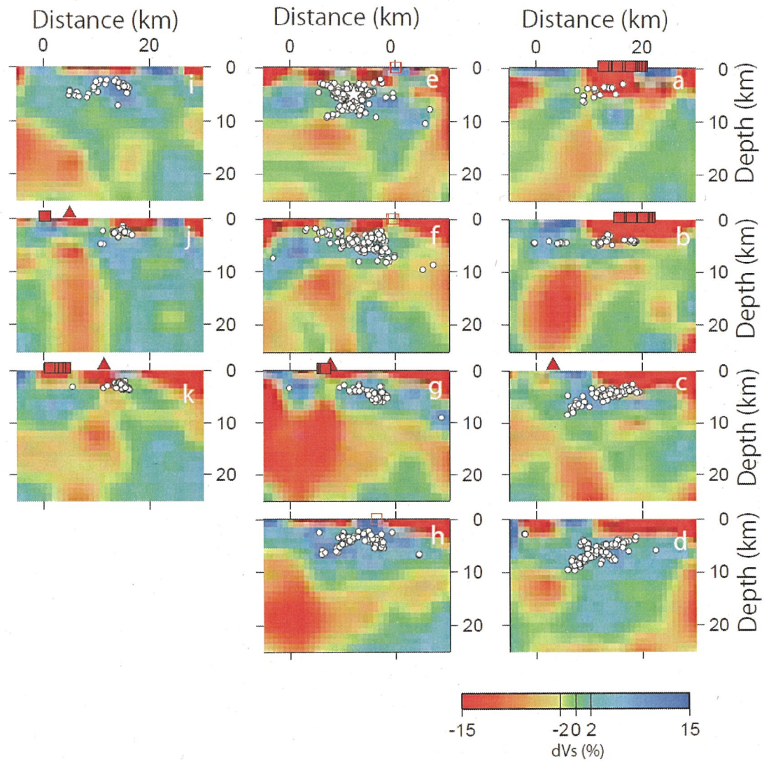
図7. 岩手・宮城内陸地震震源域におけるS波速度偏差分布. 西北西—東南東方向の断面図で示す. 白☆, 白○は, 2008年岩手・宮城内陸地震緊急観測グループによる本震および余震(6/23-6/30, 7/2-7/7)を示す. 赤△は第四紀火山を示す. 赤■および□は活断層および地表地震変状の位置を示す. 本震震源直下(断面図 e)には流体の上昇経路に対応すると考えられる低速度域が分布する. 左下: 深さ3kmにおけるS波速度偏差分布. 赤四角は地震断層の概略を示す.
