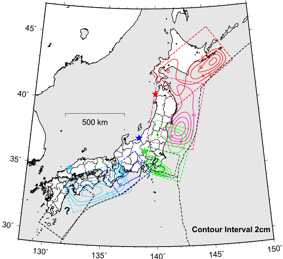
図1-1-3. すべり欠損分布.
