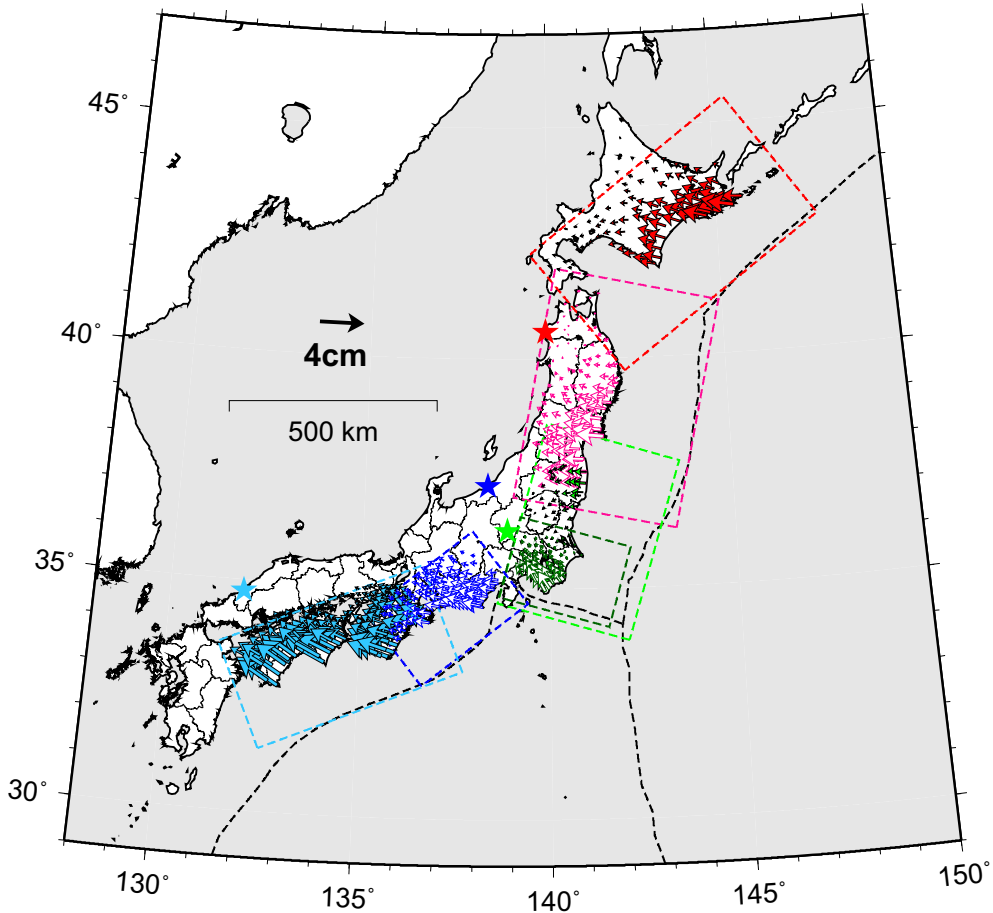
図1-1-4. すべり欠損による変位場.
