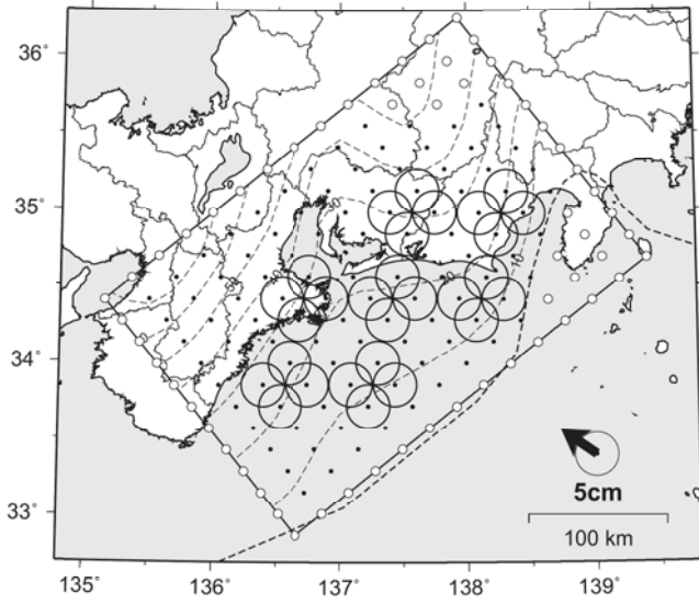
図2-5-3. 与えたすべり分布
