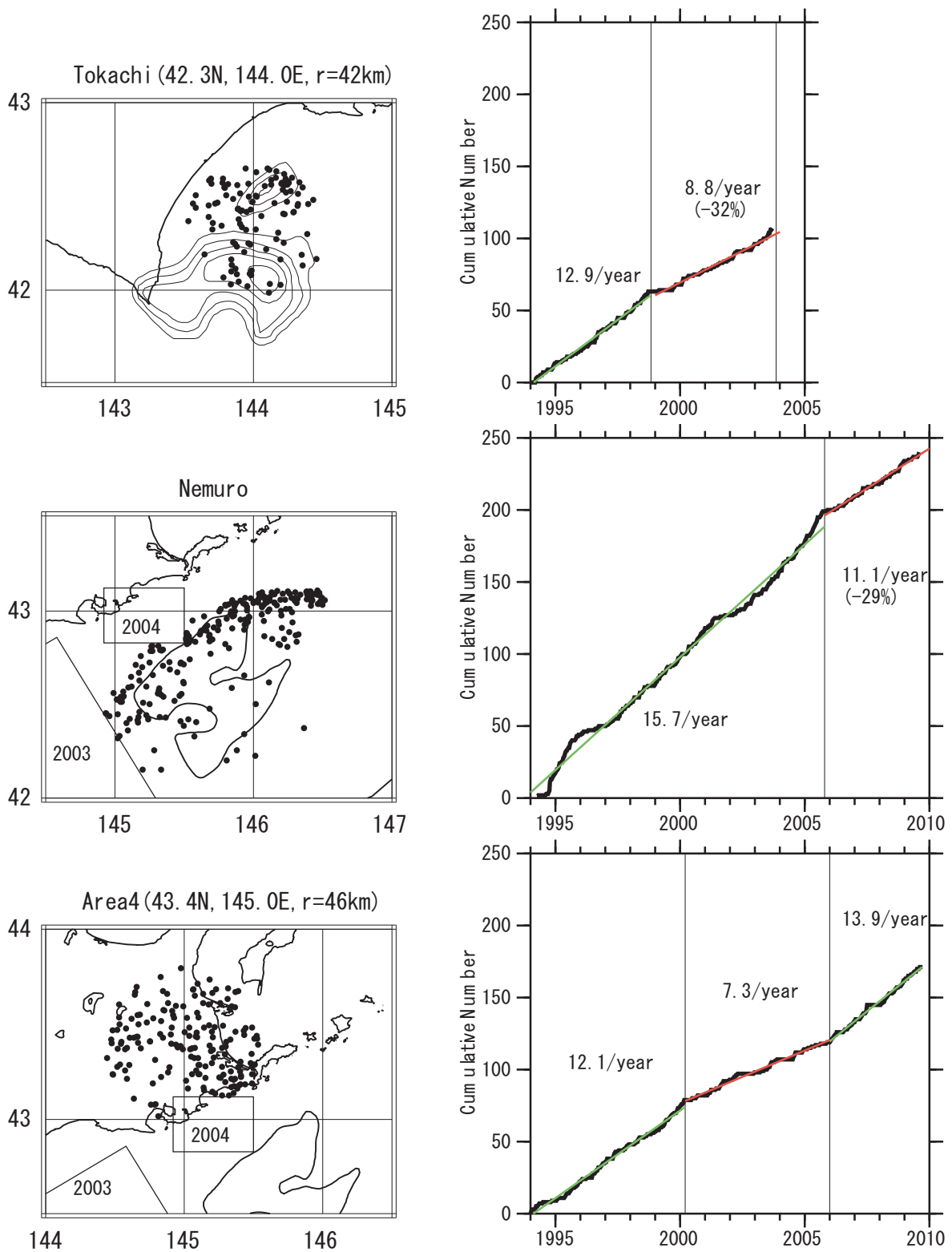
図3. 震央分布と積算度数。2003年十勝沖地震と1973年根室半島沖地震のアスペリティをコンターで示す (Yamanaka and Kikuchi, 2003)。十勝沖では1998年10月頃から静穏化が開始した。根室沖では2005年10月頃から静穏化が開始し、現在も継続中である。Area4では2000年4月頃から静穏化が始まったが、2005年12月頃から以前の発生レートに戻っている。
