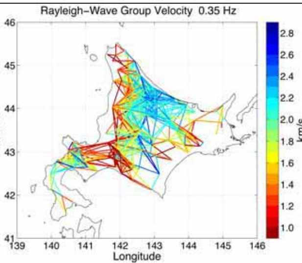
地震ノイズ干渉法によって得られた0.35Hzレリー波の群速度
