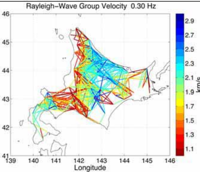
地震ノイズ干渉法によって得られた0.30Hzレリー波の群速度
