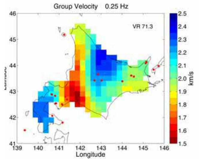
地震ノイズ干渉法によって得られた0.25Hzレリー波の群速度
