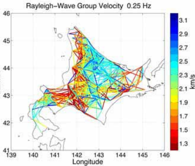
地震ノイズ干渉法によって得られた0.25Hzレリー波の群速度
