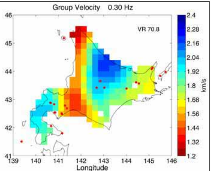
地震ノイズ干渉法によって得られた0.30Hzレリー波の群速度
