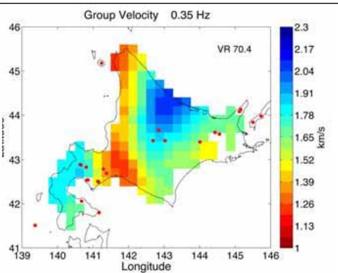
地震ノイズ干渉法によって得られた0.35Hzレリー波の群速度
