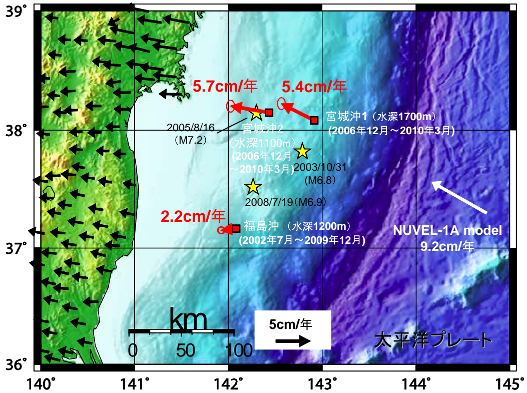
図1 ユーラシアプレート安定域に対する速度ベクトル
