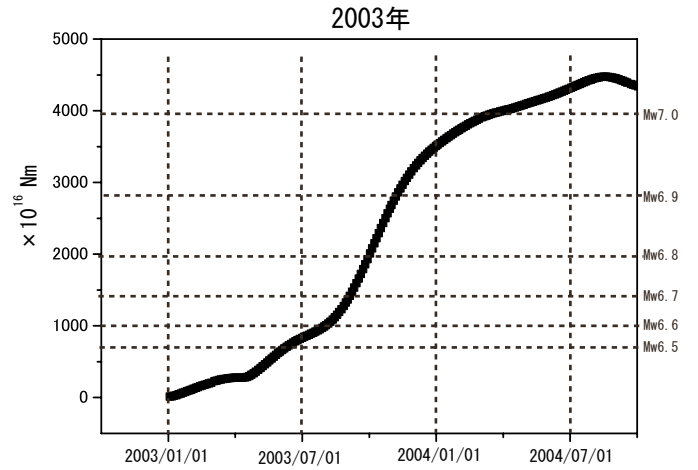
推定すべりの積算モーメント
