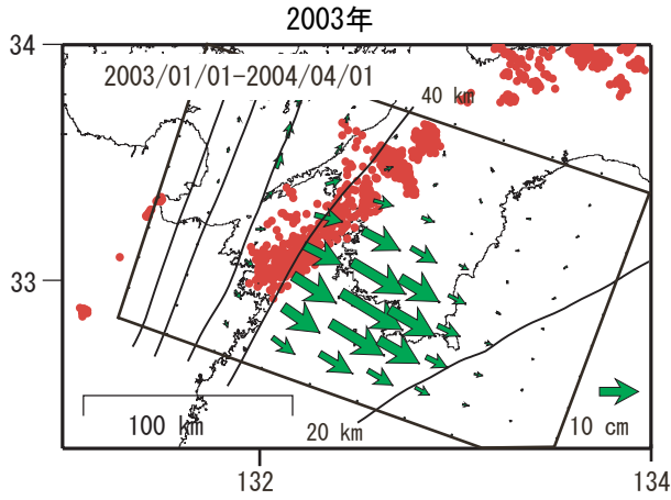
推定プレート間すべり分布
