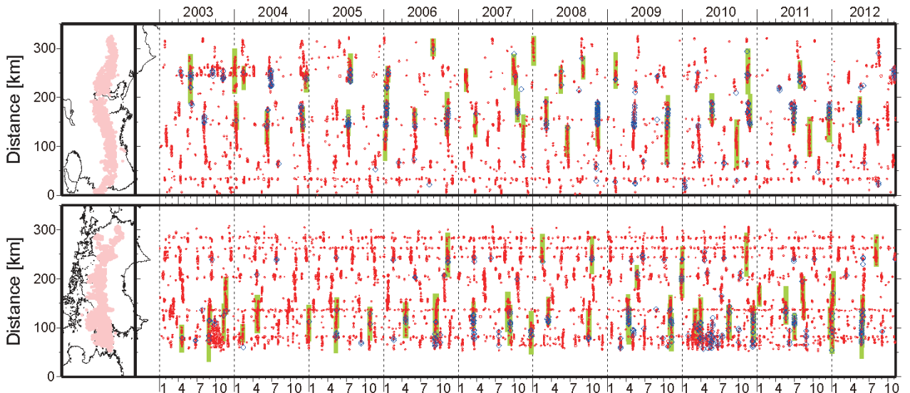
図3. 2003年1月～2012年11月9日までの深部低周波微動 (赤) および，深部超低周波地震 (青菱形) の時空間分布. 緑太線は，傾斜変動から検出された短期的 SSE.
