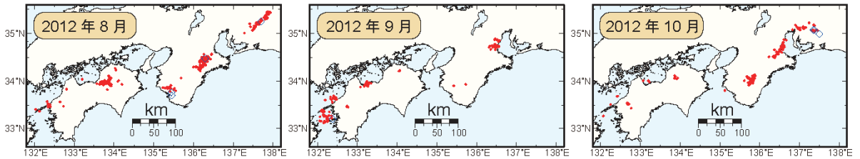
図1. 西南日本における2012年8月～10月の月毎の深部低周波微動活動. 赤丸はエンベロープ相関・振幅ハイブリッド法 (Maeda and Obara, 2009) およびクラスター処理 (Obara et al., 2010) において，1時間毎に自動処理された微動分布の重心である. 青菱形は周期20秒に卓越する深部超低周波地震 (Ito et al., 2007) である.
