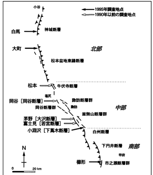
糸魚川－静岡構造線活断層系の概要 (地震調査研究推進本部 HP より引用)
