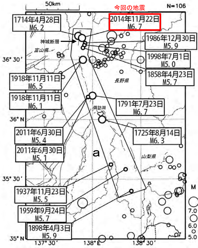
図中の細線は、地震調査研究推進本部による 主要活断層帯を示す。
