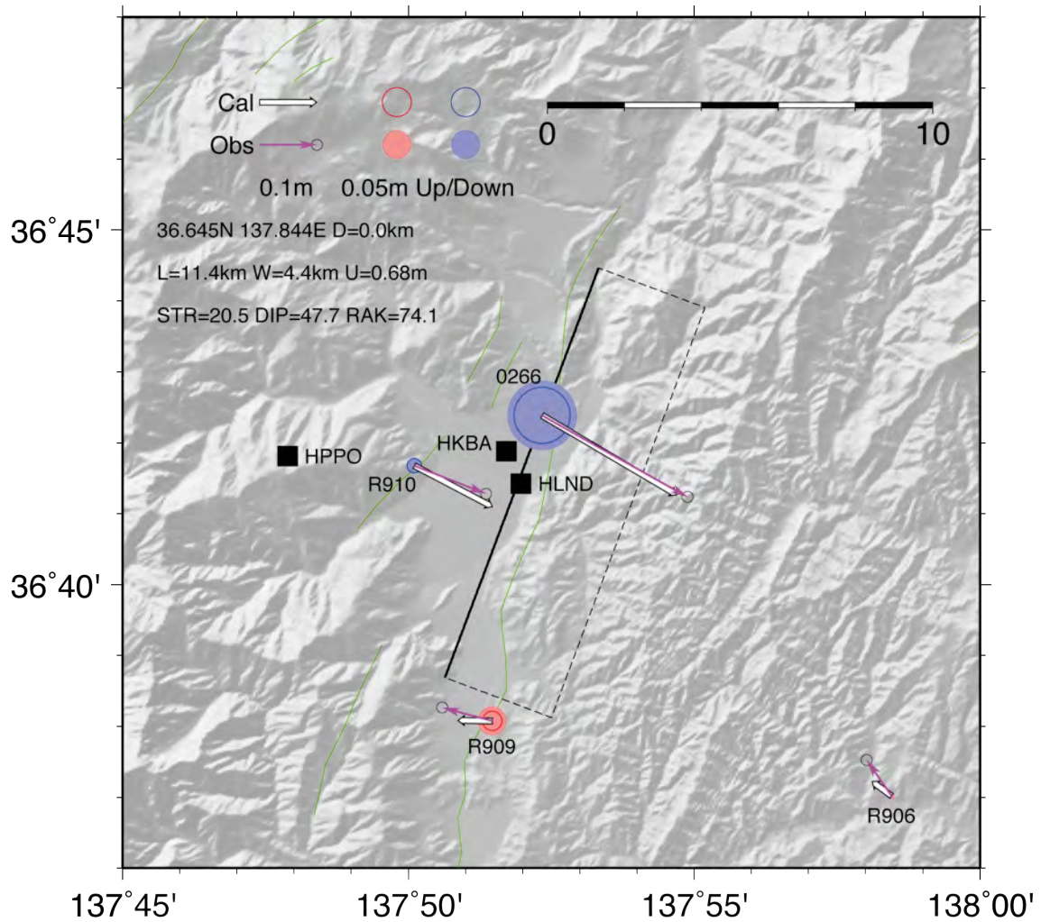
図2 白馬周辺のGPS観測点分布と長野県北部地震に伴う変位、および推定された断層モデル。塗りつぶした丸印は観測された上下変位を、中抜きの丸印は上下変位の計算値を示す。
