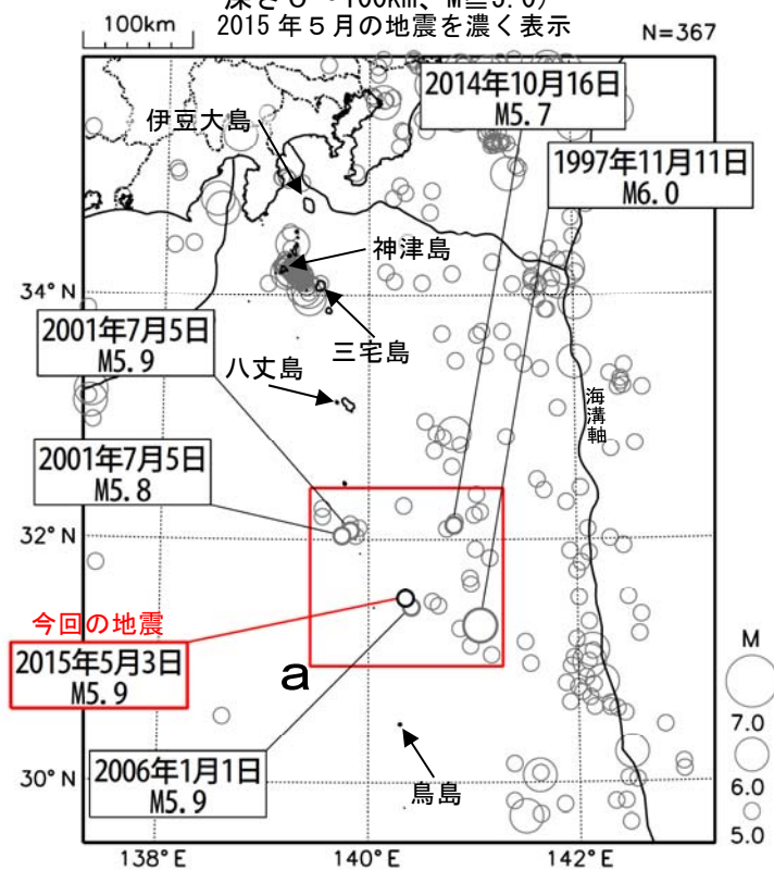
図 2-1 震央分布図
