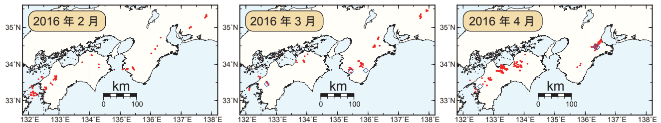
図 1. 西南日本における 2016 年 2 月～4 月の月毎の深部低周波微動活動．赤丸はエンベロープ相関・振幅ハイブリッド法 (Maeda and Obara, 2009) およびクラスタ処理 (Obara et al., 2010) において，1 時間毎に自動処理された微動分布の重心である．青菱形は周期 20 秒に卓越する深部超低周波地震 (Ito et al., 2007) である．
