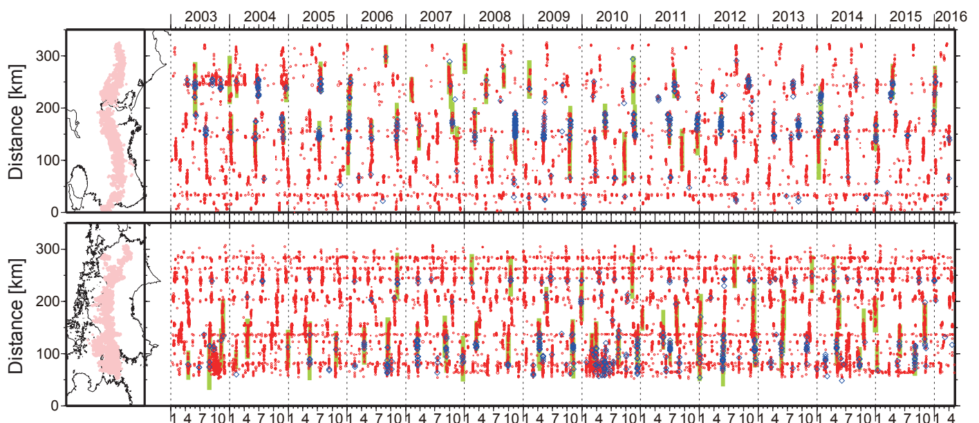
図 3. 2003 年 1 月～2016 年 5 月 8 日までの深部低周波微動（赤）および，深部超低周波地震（青菱形）の時空間分布．緑太線は，傾斜変動から検出された短期的スロースリップイベント．
