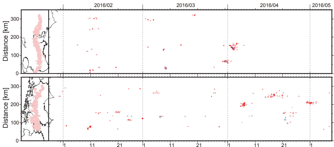
図 2. 2016 年 1 月 30 日～5 月 8 日の深部低周波微動（赤）および，深部超低周波地震（青菱形）の時空間分布．
