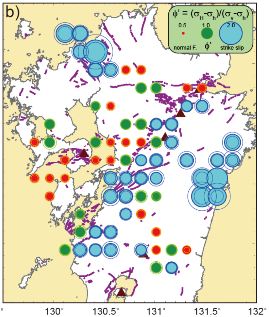
応力比から求めた応力区分 (青、緑、赤: 横ずれ、1軸伸張、正断層応力場)
