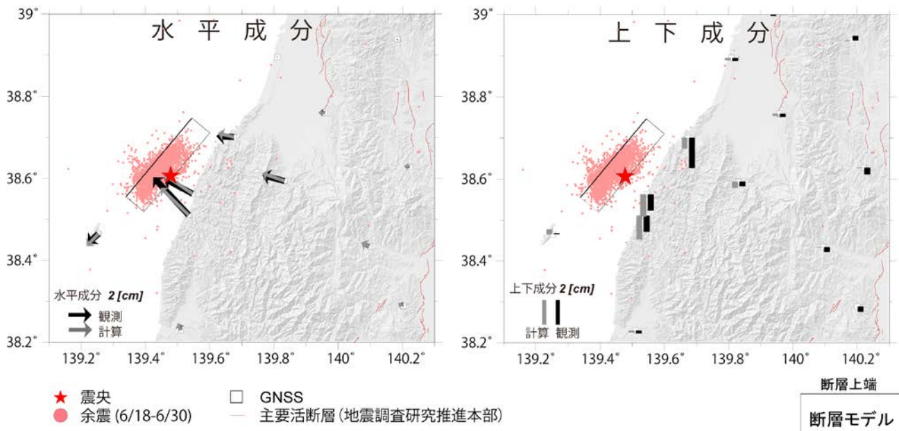
図1 東に傾き下がる断層面を仮定した場合の震源断層モデル。
