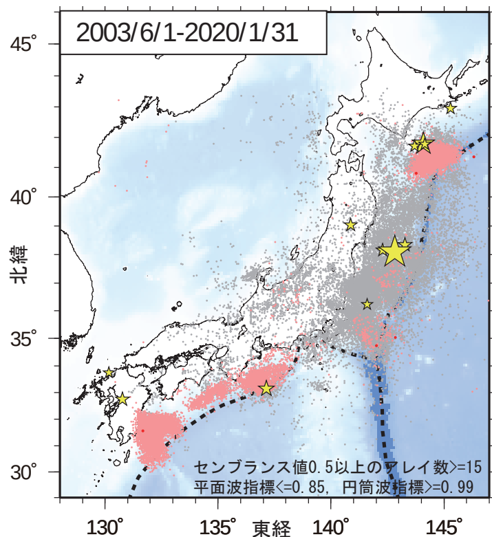
第1図. 2003年6月1日から2020年1月31日までの期間にアレイ解析によって検出されたイベントの震央分布. 検出イベントを防災科研 Hi-net の手動または自動検測震源と照合し, 対応する地震が見出されたイベントを灰色で, それ以外を桃色 (2019年10月31日以前), および赤色 (11月1日以降) の点でそれぞれ示す. これらは主として周期10秒以上に卓越する超低周波地震を表すが, 東北地方太平洋沖地震の発生以降は, 除去しきれない通常地震を含む. 期間内に発生した M7 以上の地震 (ただし, 2011年～2015年の期間は東北地方太平洋沖地震の本震のみ) の震央を黄色星印で示す.
