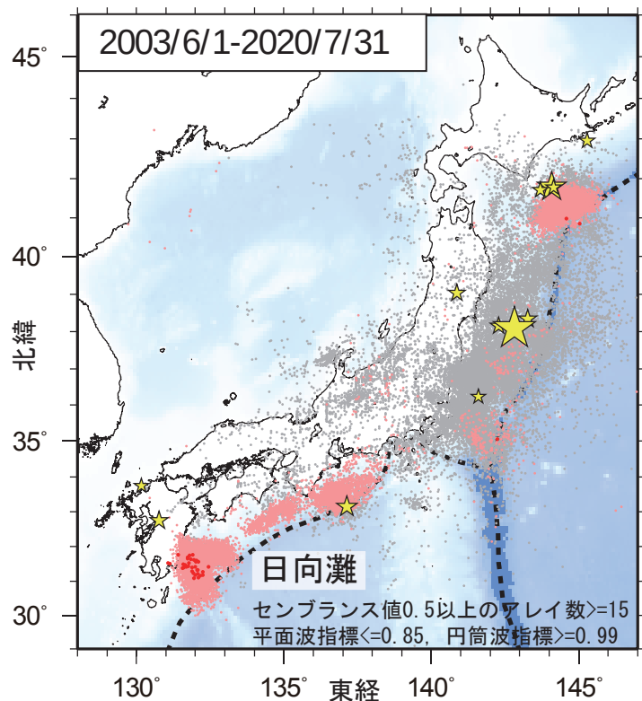
第1図. 2003年6月1日から2020年7月31日までの期間にアレイ解析によって検出されたイベントの震央分布. 検出イベントを防災科研 Hi-net の手動または自動検測震源と照合し, 対応する地震が見出されたイベントを灰色で, それ以外を桃色 (2020年4月30日以前), および赤色 (5月1日以降) の点でそれぞれ示す. これらは主として周期10秒以上に卓越する超低周波地震を表すが, 東北地方太平洋沖地震の発生以降は, 除去しきれない通常の地震を含む. 期間内に発生した M7 以上の地震 (ただし, 2011年～2015年の期間は東北地方太平洋沖地震の本震のみ) の震央を黄色星印で示す.
