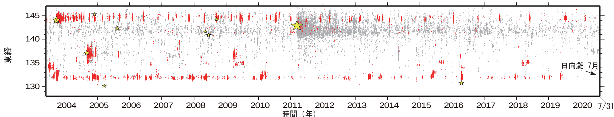
第3図. 2003年6月1日から2020年7月31日までの期間に検出されたイベントの時空間分布. 検出されたイベントを防災科研 Hi-net 手動または自動検測震源と照合し, 対応する地震が見出されたイベントを灰色で, それ以外を赤色の点でそれぞれ示す. その他は第1図に同じ.
