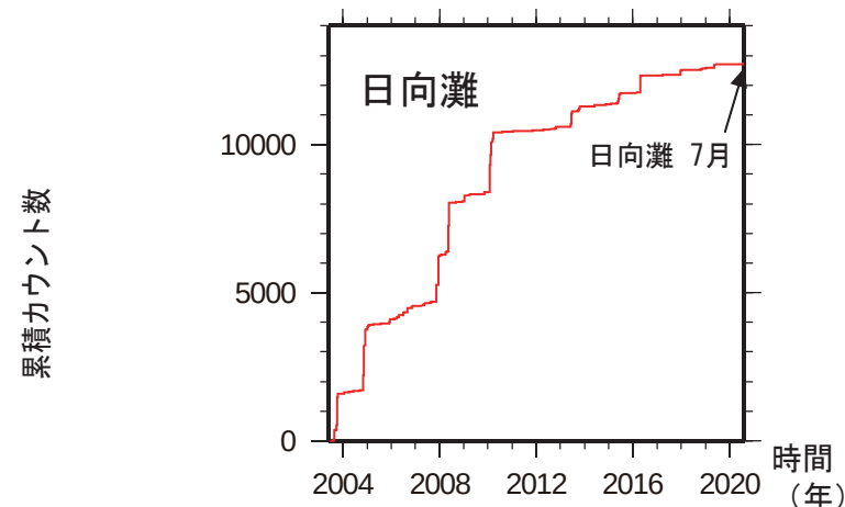
第2図. 日向灘における検出イベントの累積カウント数の時間変化. 幅60秒間の解析時間窓を15秒毎に設定し, それぞれの解析時間窓内にイベントが検出される度に1カウントと数えるよう定義した.
