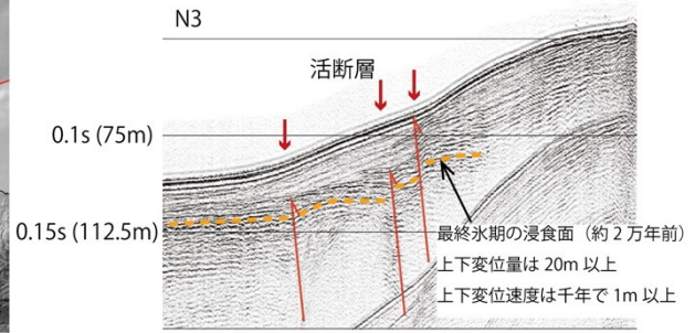
図1 能登半島海域の活断層と2024年地震の余震分布（左）および反射断面の解釈（右）
