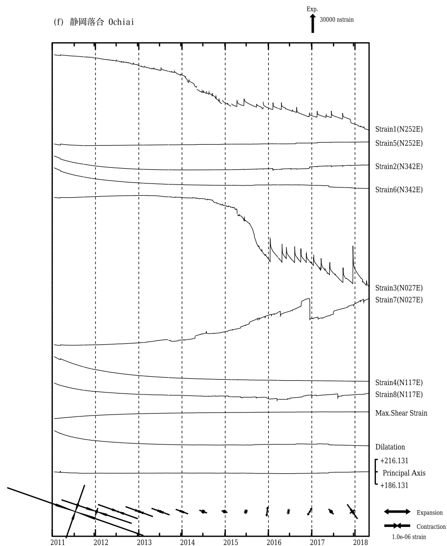
第4図(f)～(k) 左：2011年1月以後の多成分ひずみ計変化（日平均値）。主ひずみ・最大せん断ひずみ・面積ひずみは各方向成分から計算されている。 右：2017年11月～2018年4月の多成分ひずみ計変化（時間値：気圧・潮汐・地磁気補正した値）。各図下部に気圧変化と降水量を示す。
