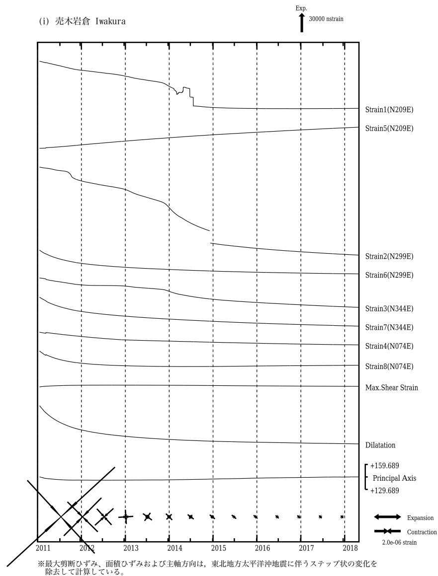
第4図(f)～(k) 左：2011年1月以後の多成分ひずみ計変化（日平均値）。主ひずみ・最大せん断ひずみ・面積ひずみは各方向成分から計算されている。 右：2017年11月～2018年4月の多成分ひずみ計変化（時間値：気圧・潮汐・地磁気補正した値）。各図下部に気圧変化と降水量を示す。
