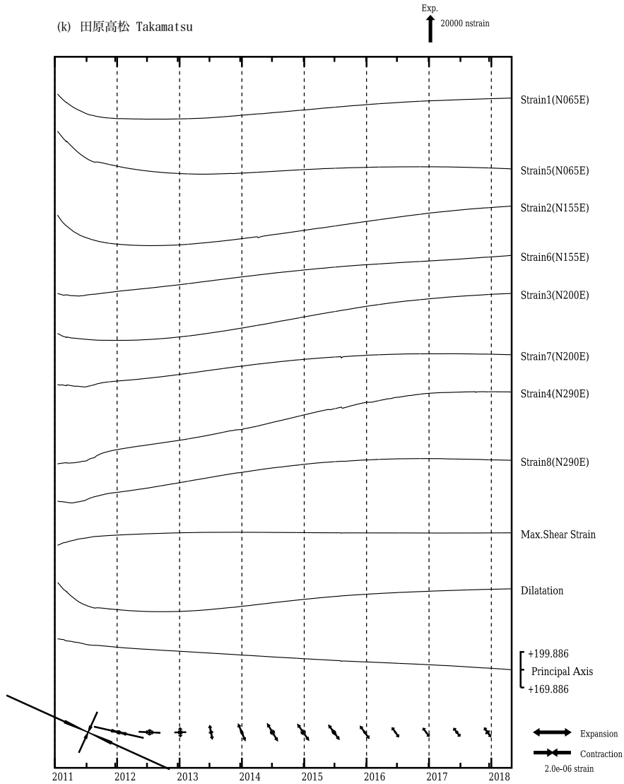
第4図(f)～(k) 左：2011年1月以後の多成分ひずみ計変化（日平均値）。主ひずみ・最大せん断ひずみ・面積ひずみは各方向成分から計算されている。 右：2017年11月～2018年4月の多成分ひずみ計変化（時間値：気圧・潮汐・地磁気補正した値）。各図下部に気圧変化と降水量を示す。
