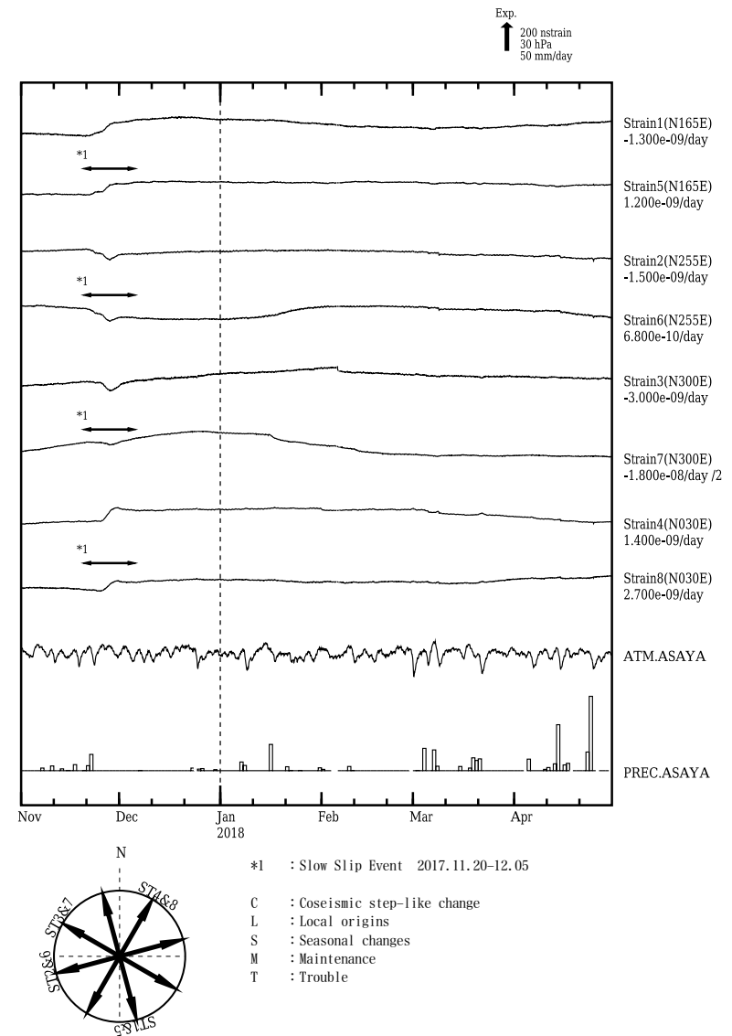
第4図(f)～(k) 左：2011年1月以後の多成分ひずみ計変化（日平均値）。主ひずみ・最大せん断ひずみ・面積ひずみは各方向成分から計算されている。 右：2017年11月～2018年4月の多成分ひずみ計変化（時間値：気圧・潮汐・地磁気補正した値）。各図下部に気圧変化と降水量を示す。
