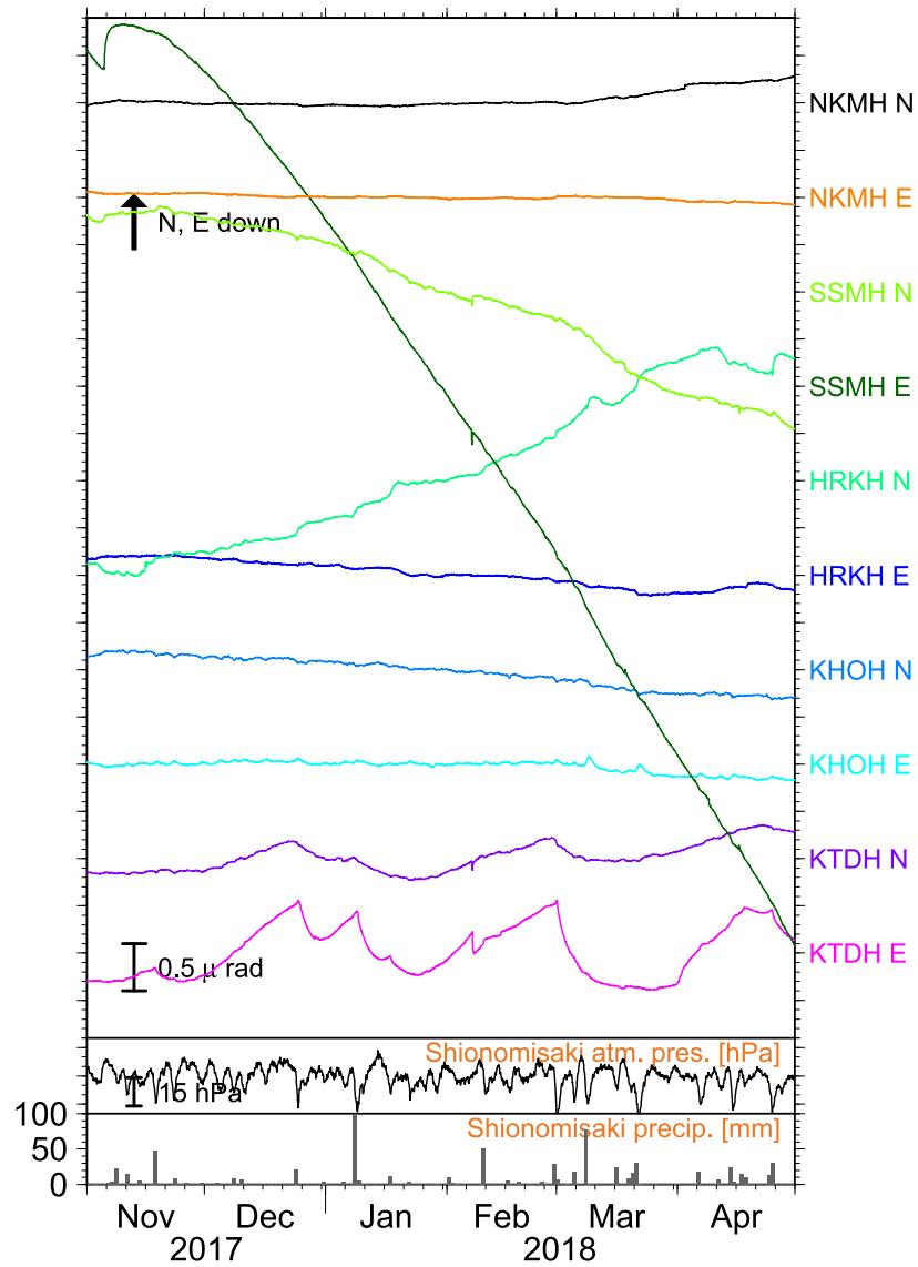
第 2e 図 つづき（紀伊半島南西部，潮岬 気圧・雨量）
