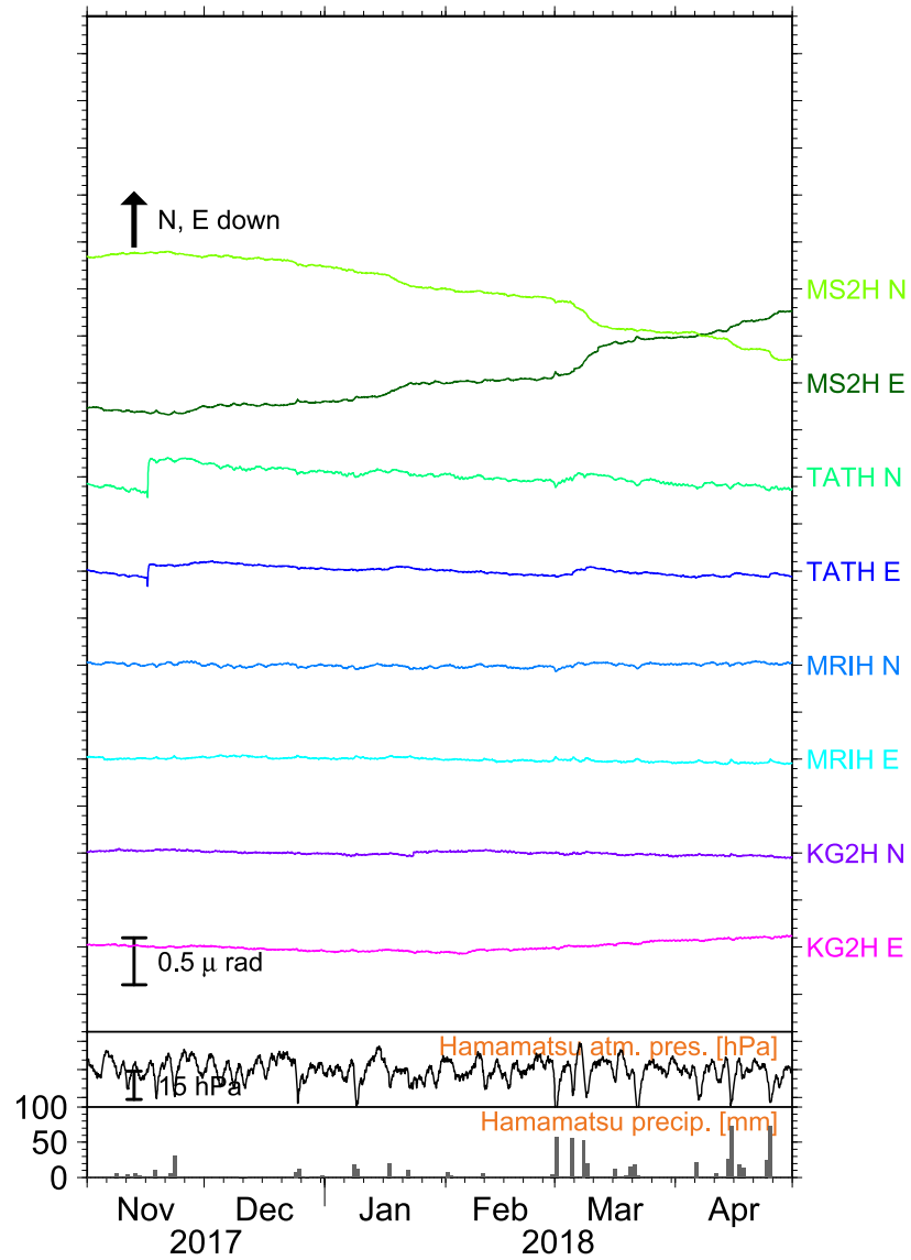
第 2i 図 つづき (静岡西部, 浜松気圧・雨量)
