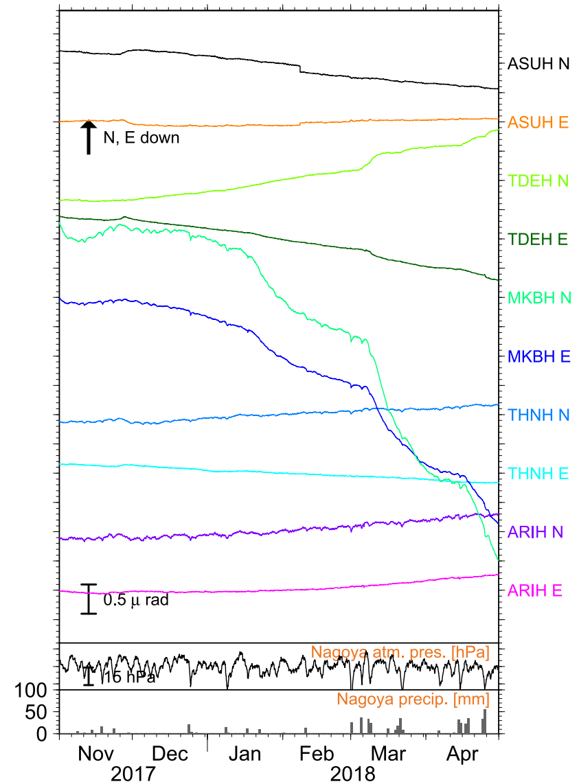
第 2h 図 つづき (愛知東部, 名古屋気圧・雨量)
