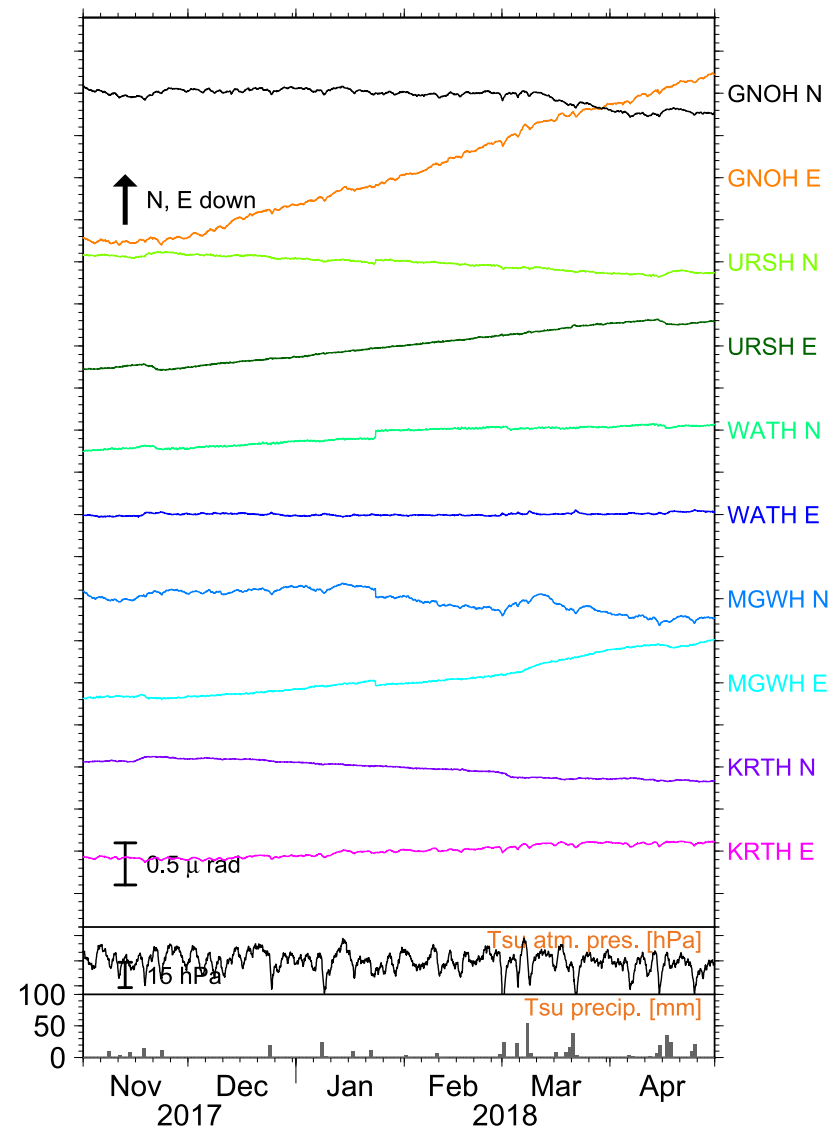
第 2f 図 傾斜の時間値記録及び津での気圧・日雨量（紀伊半島北東部）.
