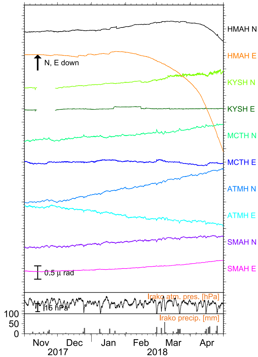
第 2g 図 つづき (愛知西部, 伊良湖気圧・雨量)
