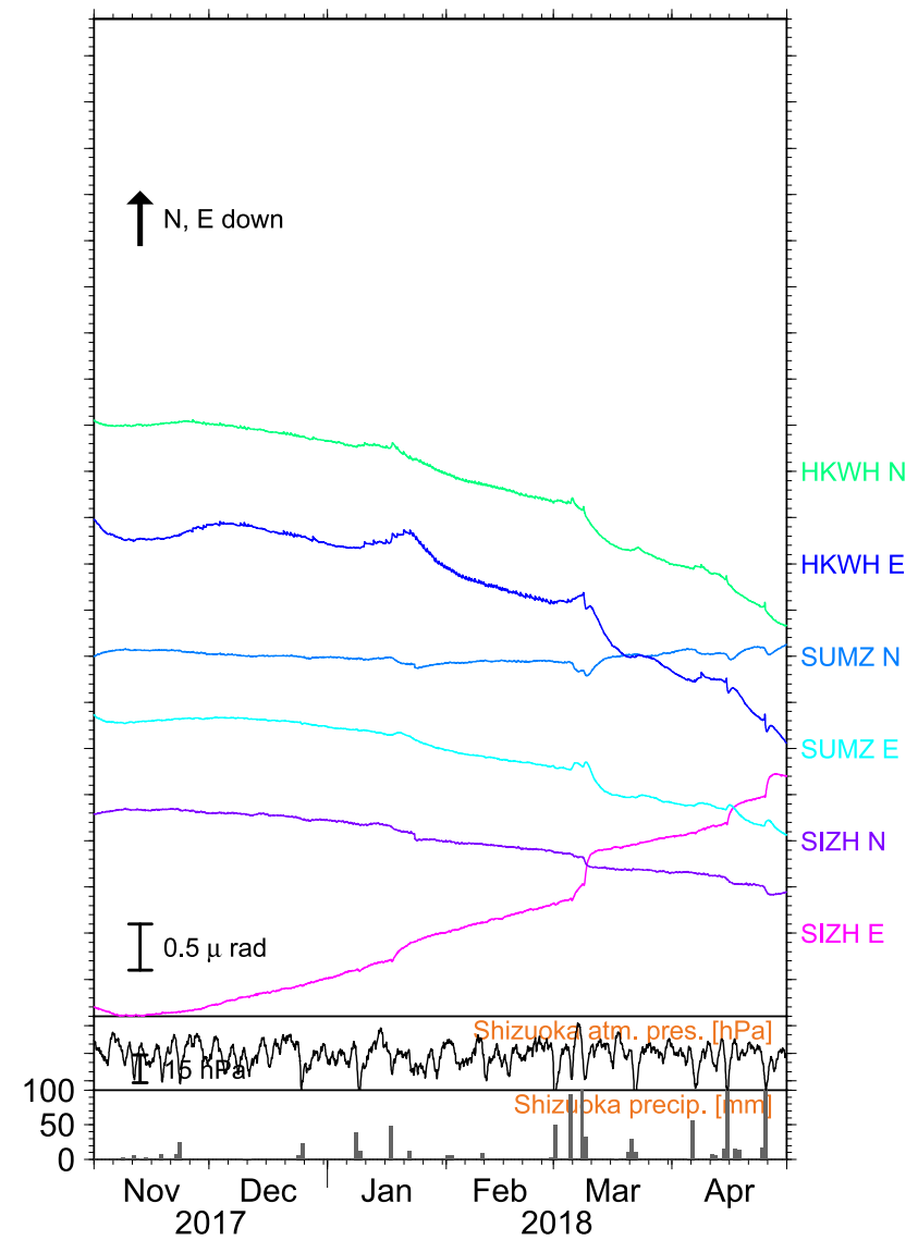
第 2j 図 つづき (静岡中北部, 静岡気圧・雨量)
