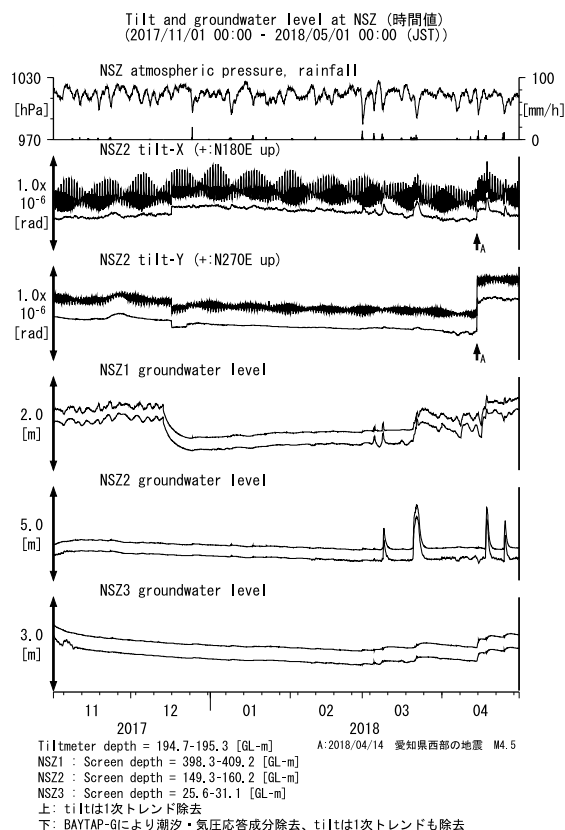
第5図 NSZにおける傾斜・地下水位観測結果 (2017年11月～2018年4月) Fig. 5 Observed tilts and groundwater levels at the NSZ observation site from November 2017 to April 2018.
