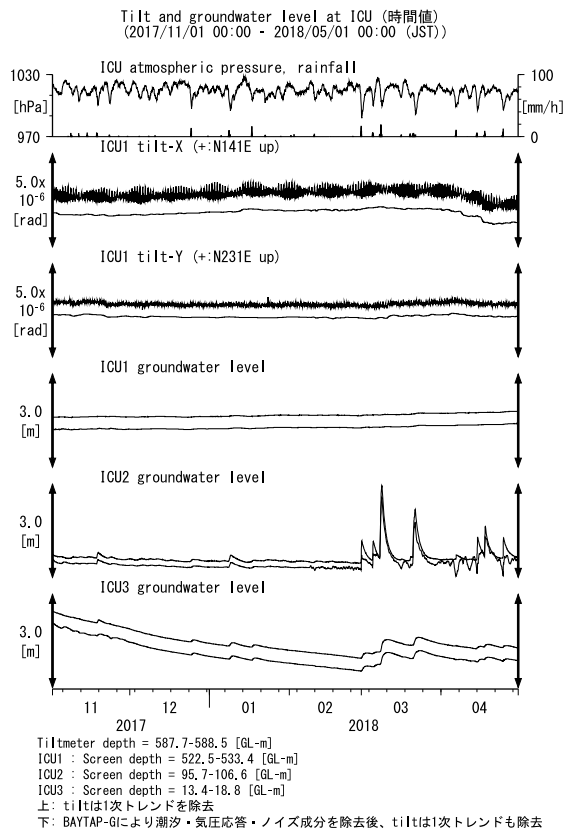
第16図 ICUにおける傾斜・地下水位観測結果 (2017年11月～2018年4月) Fig. 16 Observed tilts and groundwater levels at the ICU observation site from November 2017 to April 2018.
