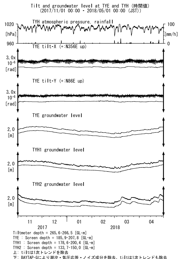
第 7 図 TYE および TYH における傾斜・地下水位観測結果 (2017 年 11 月～2018 年 4 月) Fig. 7 Observed tilts and groundwater levels at the TYE and the TYH observation site from November 2017 to April 2018.
