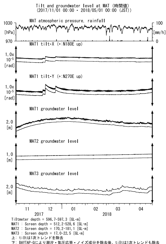
第36図 MATにおける傾斜・地下水位観測結果 (2017年11月～2018年4月) Fig. 36 Observed tilts and groundwater levels at the MAT observation site from November 2017 to April 2018.
