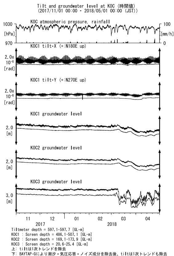
第 28 図 KOC における傾斜・地下水位観測結果 (2017 年 11 月～2018 年 4 月) Fig. 28 Observed tilts and groundwater levels at the KOC observation site from November 2017 to April 2018.
