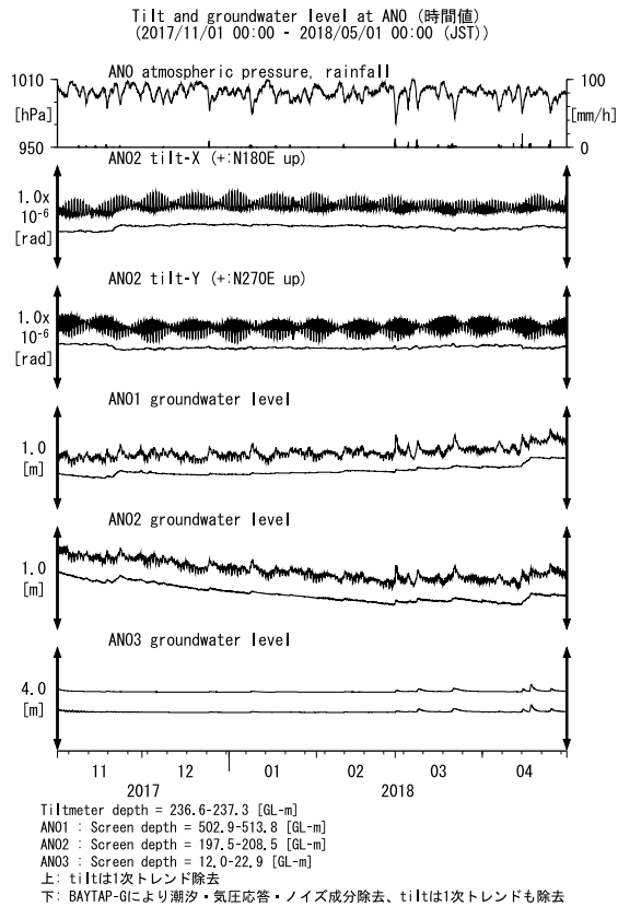
第10図 ANOにおける傾斜・地下水位観測結果 (2017年11月～2018年4月) Fig. 10 Observed tilts and groundwater levels at the ANO observation site from November 2017 to April 2018.
