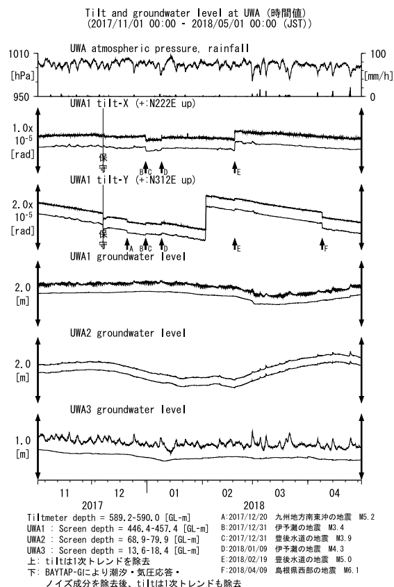
第34図 UWAにおける傾斜・地下水位観測結果 (2017年11月～2018年4月) Fig. 34 Observed tilts and groundwater levels at the UWA observation site from November 2017 to April 2018.
