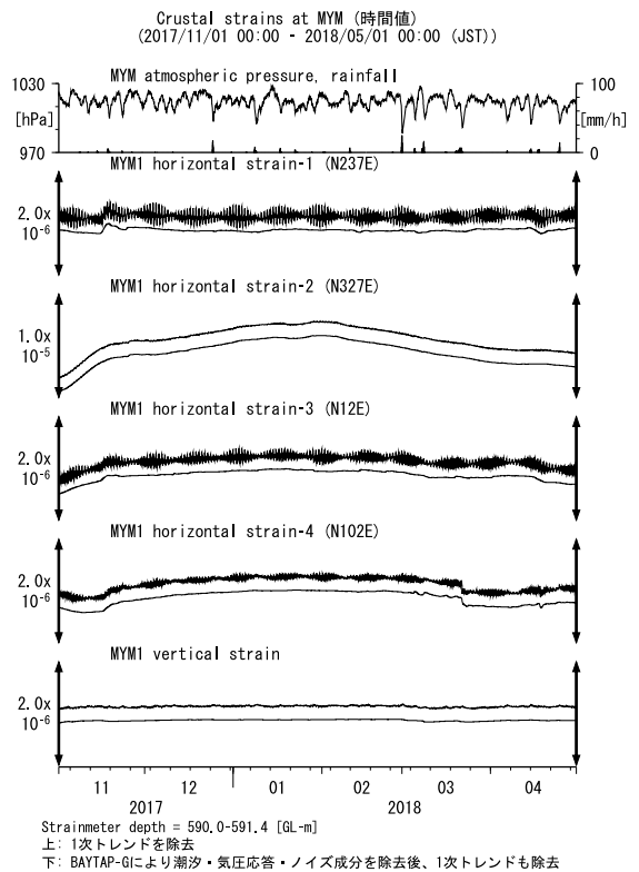
第13図 MYMにおける歪観測結果 (2017年11月～2018年4月) Fig. 13 Observed strains at the MYM observation site from November 2017 to April 2018.
