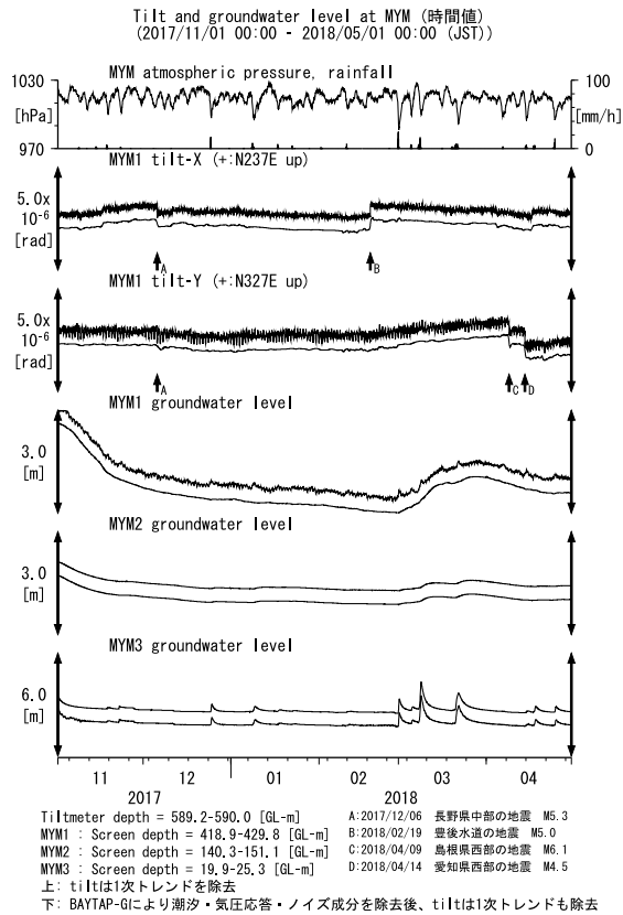
第14図 MYMにおける傾斜・地下水位観測結果 (2017年11月～2018年4月) Fig. 14 Observed tilts and groundwater levels at the MYM observation site from November 2017 to April 2018.
