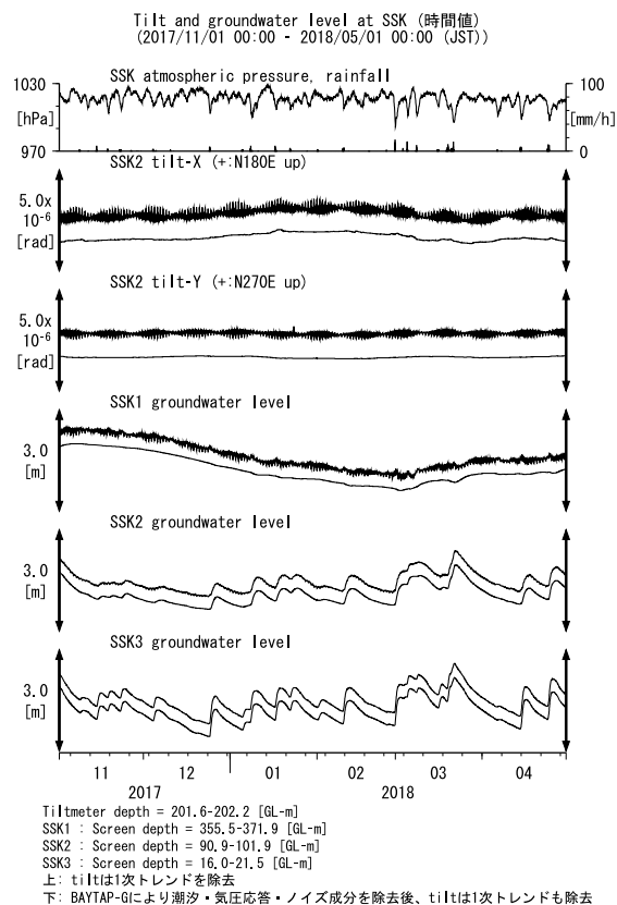
第30図 SSKにおける傾斜・地下水位観測結果 (2017年11月～2018年4月)
