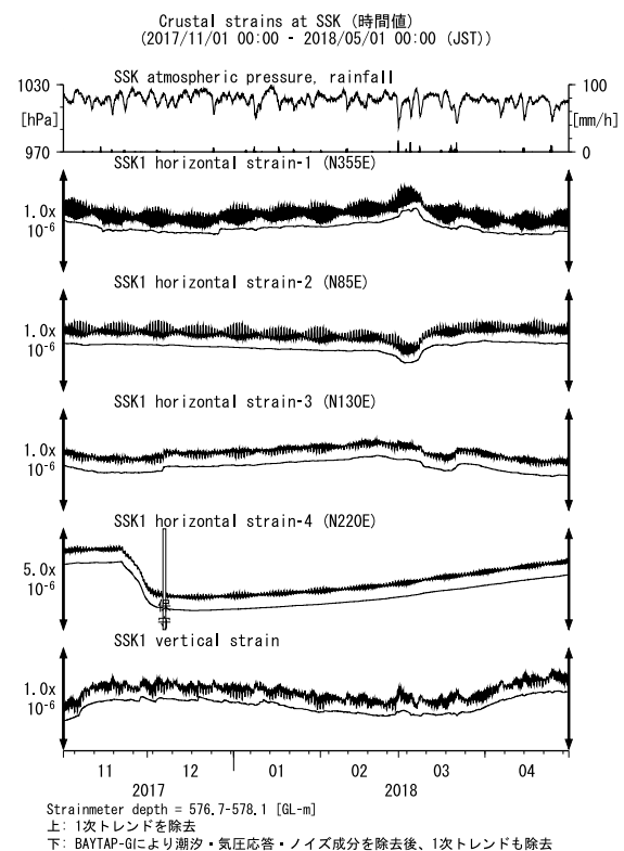
第 29 図 SSK における歪観測結果 (2017 年 11 月～2018 年 4 月) Fig. 29 Observed strains at the SSK observation site from November 2017 to April 2018.
