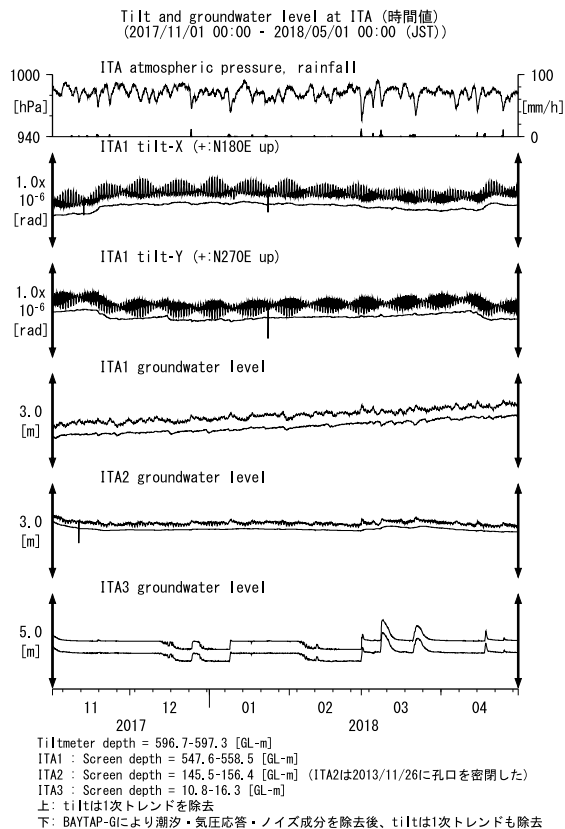
第12図 ITAにおける傾斜・地下水位観測結果 (2017年11月～2018年4月) Fig. 12 Observed tilts and groundwater levels at the ITA observation site from November 2017 to April 2018.
