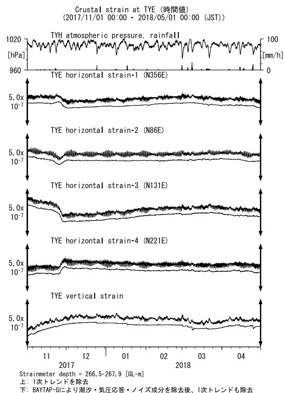
第 6 図 TYE における歪観測結果 (2017 年 11 月～2018 年 4 月) Fig. 6 Observed strains at the TYE observation site from November 2017 to April 2018.
