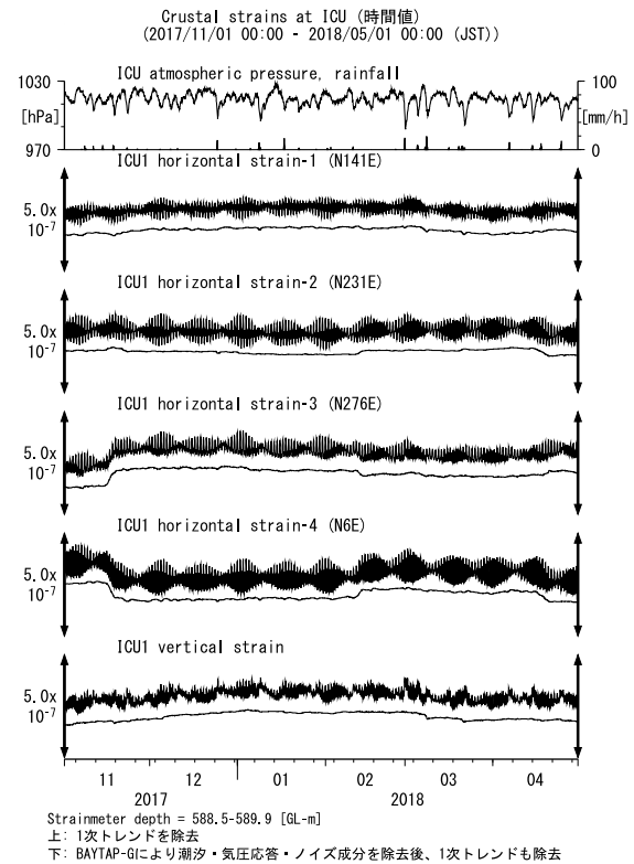
第15図 ICUにおける歪観測結果 (2017年11月～2018年4月) Fig. 15 Observed strains at the ICU observation site from November 2017 to April 2018.
