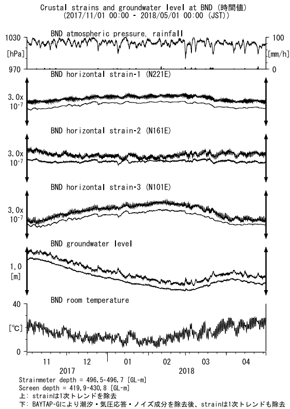
第 22 図 BND における歪・地下水位観測結果 (2017 年 11 月～2018 年 4 月)
