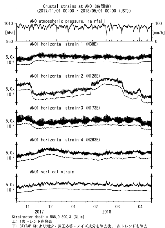
第 9 図 ANO における歪観測結果 (2017 年 11 月～2018 年 4 月) Fig. 9 Observed strains at the ANO observation site from November 2017 to April 2018.
