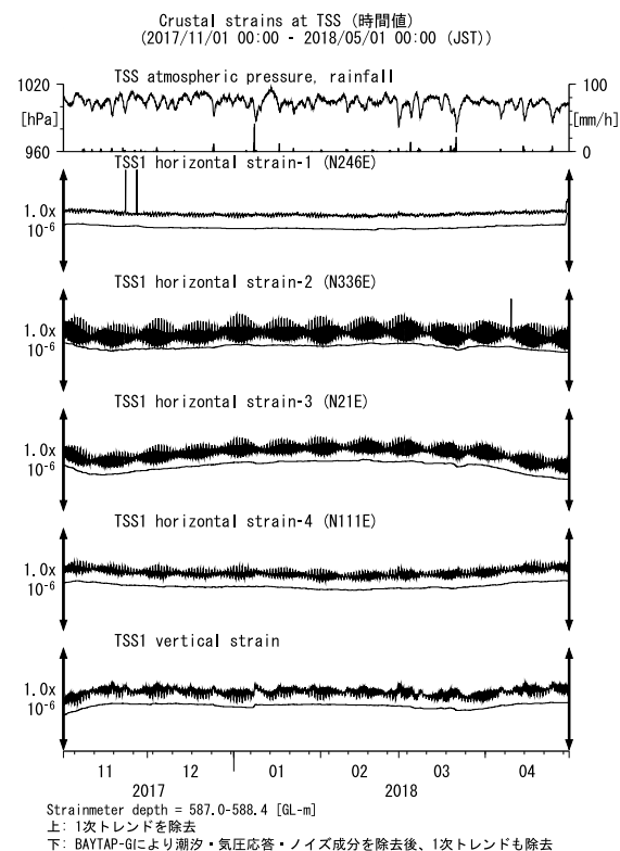
第31図 TSSにおける歪観測結果 (2017年11月～2018年4月)
