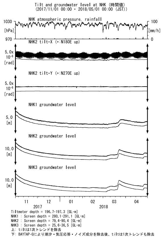
第 38 図 NHK における傾斜・地下水位観測結果 (2017 年 11 月～2018 年 4 月)
