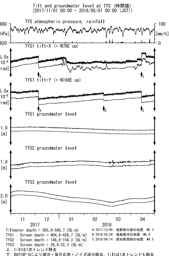
第3図 TYSにおける傾斜・地下水位観測結果 (2017年11月～2018年4月) Fig. 3 Observed tilts and groundwater levels at the TYS observation site from November 2017 to April 2018.
