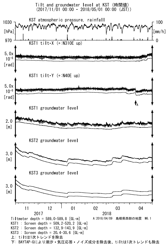
第 20 図 KST における傾斜・地下水位観測結果 (2017 年 11 月～2018 年 4 月)
