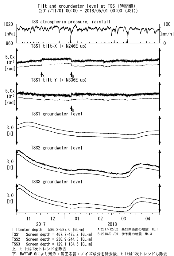
第32図 TSSにおける傾斜・地下水位観測結果 (2017年11月～2018年4月)
