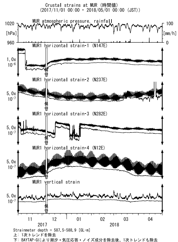
第 25 図 MUR における歪観測結果 (2017 年 11 月～2018 年 4 月)
