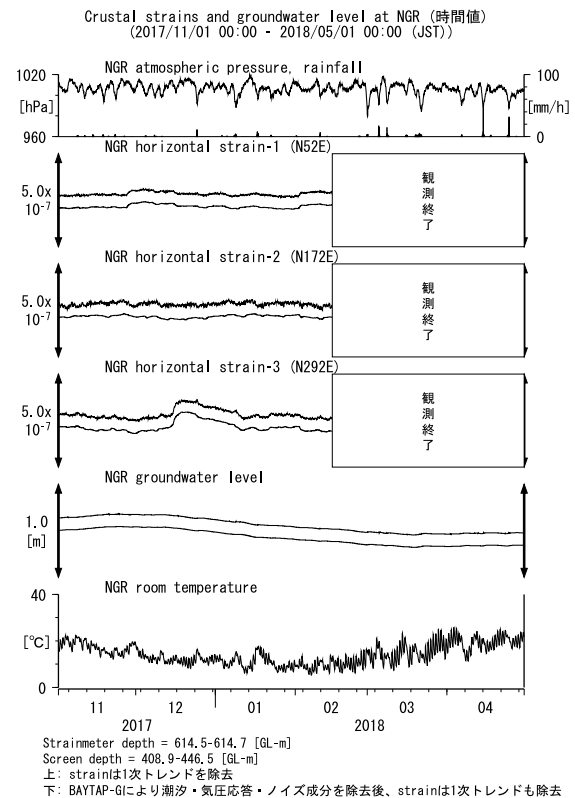
第 21 図 NGR における歪・地下水位観測結果 (2017 年 11 月～2018 年 4 月)
