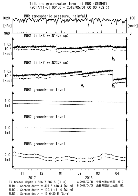
第 26 図 MUR における傾斜・地下水位観測結果 (2017 年 11 月～2018 年 4 月) Fig. 26 Observed tilts and groundwater levels at the MUR observation site from November 2017 to April 2018.
