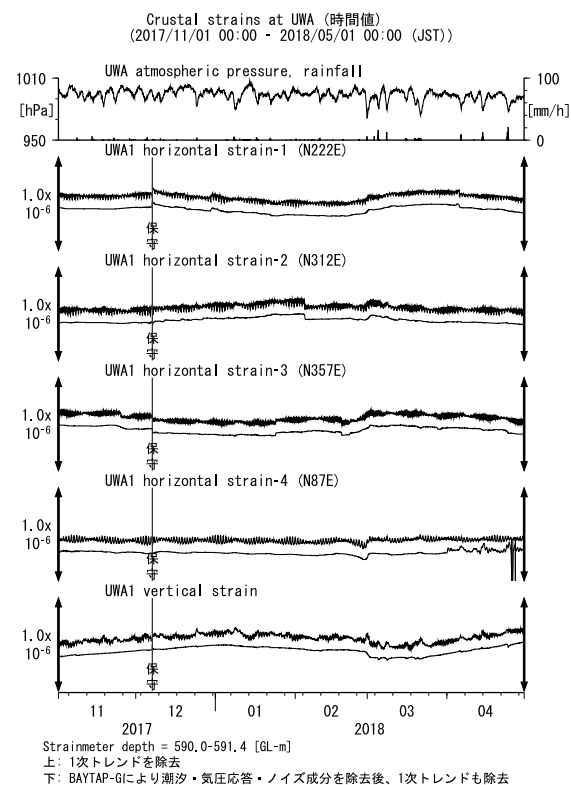
第33図 UWAにおける歪観測結果 (2017年11月～2018年4月)
