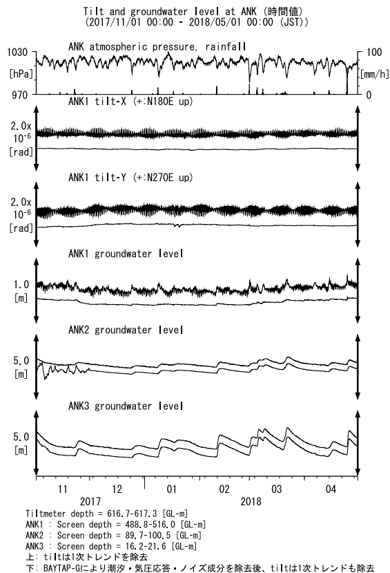
第 24 図 ANK における傾斜・地下水位観測結果 (2017 年 11 月～2018 年 4 月)
