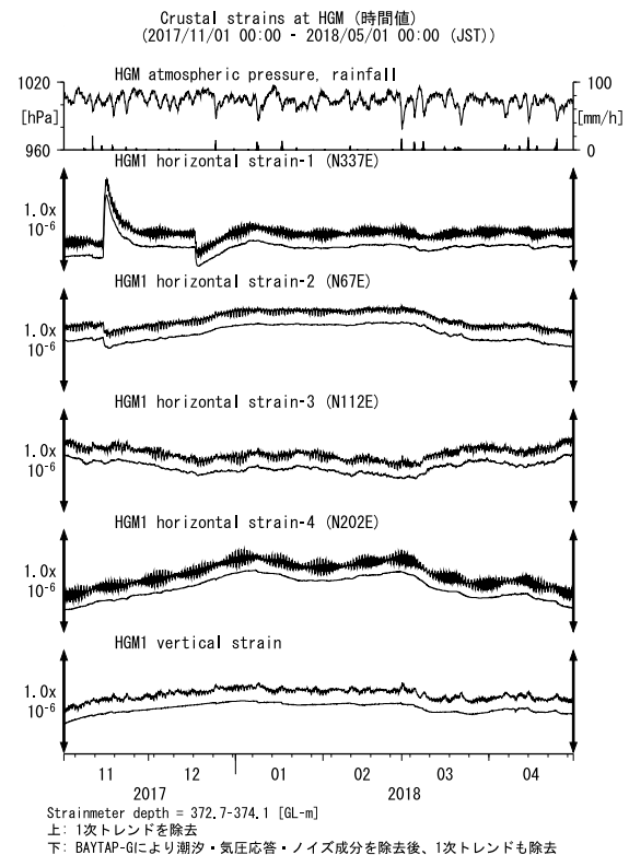
第17図 HGMにおける歪観測結果 (2017年11月～2018年4月) Fig. 17 Observed strains at the HGM observation site from November 2017 to April 2018.
