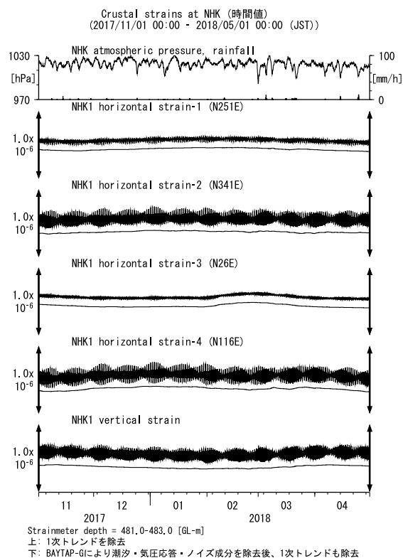
第37図 NHKにおける歪観測結果 (2017年11月～2018年4月) Fig. 37 Observed strains at the NHK observation site from November 2017 to April 2018.
