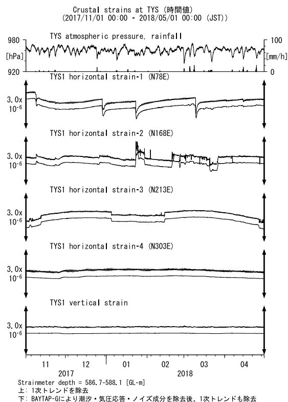
第2図 TYSにおける歪観測結果 (2017年11月～2018年4月) Fig. 2 Observed strains at the TYS observation site from November 2017 to April 2018.
