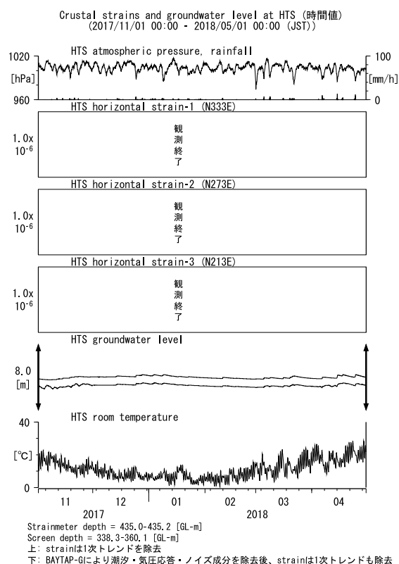
第 8 図 HTS における歪・地下水位観測結果 (2017 年 11 月～2018 年 4 月) Fig. 8 Observed strains and groundwater level at the HTS observation site from November 2017 to April 2018.
