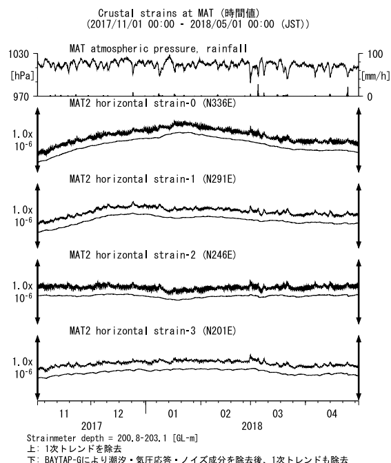
第35図 MATにおける歪観測結果 (2017年11月～2018年4月) Fig. 35 Observed strains at the MAT observation site from November 2017 to April 2018.
