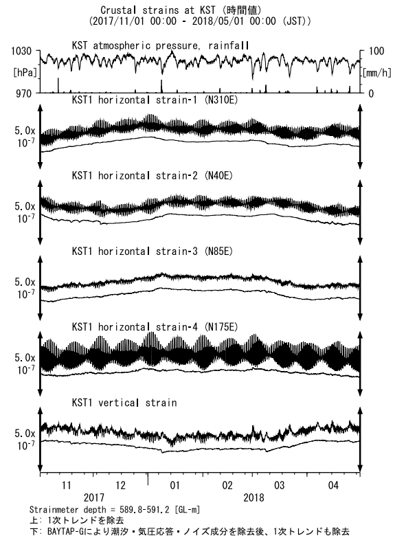
第 19 図 KST における歪観測結果 (2017 年 11 月～2018 年 4 月)
