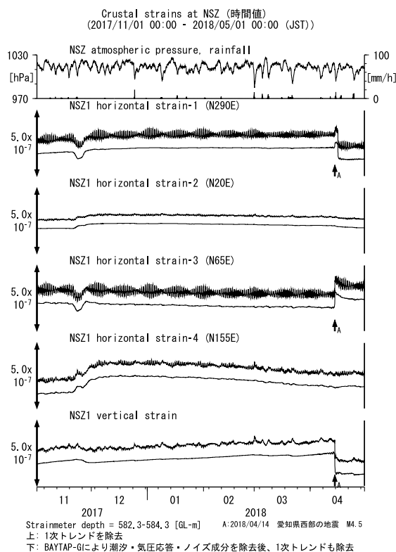
第4図 NSZにおける歪観測結果 (2017年11月～2018年4月) Fig. 4 Observed strains at the NSZ observation site from November 2017 to April 2018.
