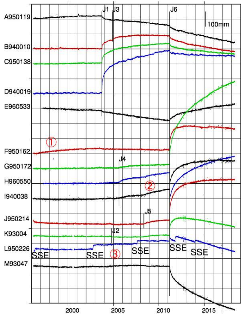
第2a図 プレート沈み込み方向の位置変化（東日本；1996年から2018年10月）沈み込みと逆方向が上向き。J1:2003年十勝沖地震(M8.0), J2:2004年新潟県中越地震(M6.8), J3:2004年11月29日釧路沖の地震(M7.1), J4:2005年8月16日宮城県沖の地震(M7.2), J5:2008年5月8日茨城県沖の地震(M7.0), J6:2011年東北地方太平洋沖地震(M9.0), J7:2015年2月17日三陸沖の地震(M6.9).
