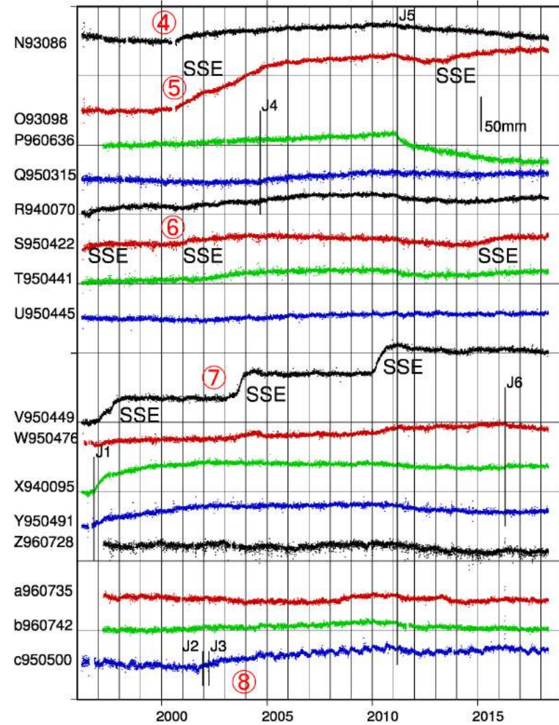
第2b図 プレート沈み込み方向の位置変化（西日本；1996年から2018年10月）沈み込みと逆方向が上向き。J1:1996年10月19日日向灘の地震(M6.9), J2:2001年12月18日与那国島近海(M7.3), J3:2002年3月31日台湾付近の地震(M7.2), J4:2004年9月5日三重県南東沖の地震(M7.4), J5:2011年東北地方太平洋沖地震(M9.0), J6:2016年熊本地震(M7.3).
