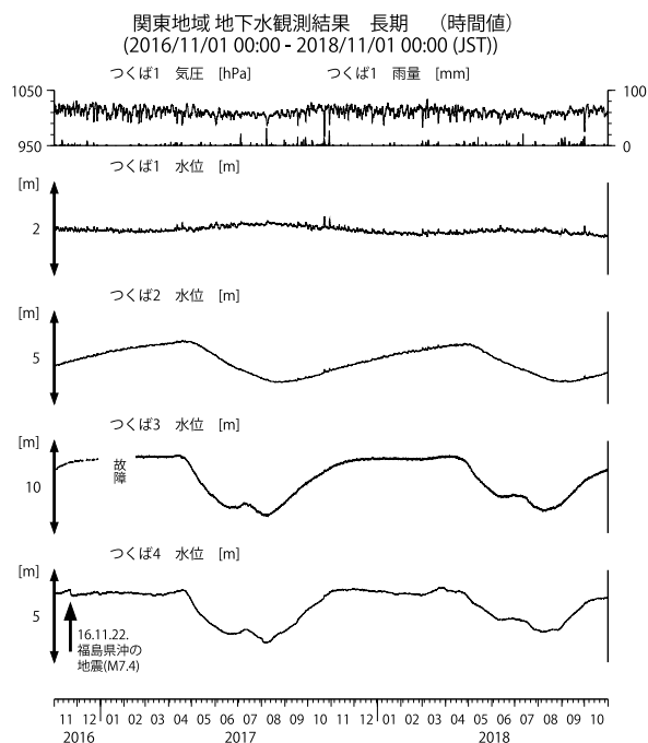
第20図 関東地域の地下水等の観測結果(2016年11月～2018年10月)
