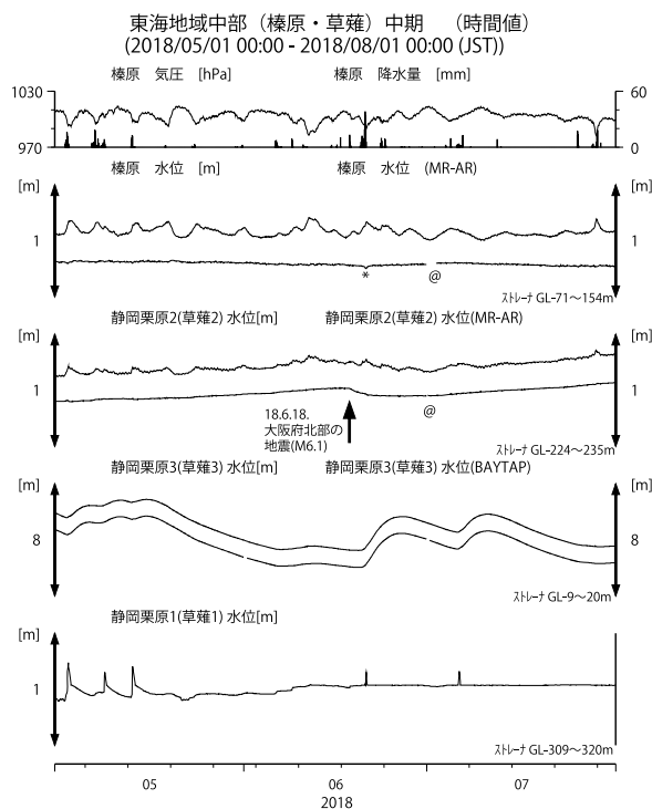
第3図 東海地域中部の地下水等の観測結果(2018年5月～2018年7月) Fig. 3 Observed groundwater levels and others in the central Tokai district from May 2018 to Jul. 2018.
