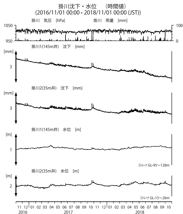
第22図 掛川における沈下等の観測結果(2016年11月~2018年10月) Fig. 22 Observed subsidence data and others at the Kakegawa observation well from Nov. 2016 to Oct. 2018.
