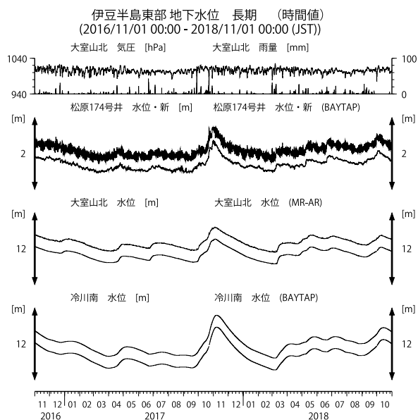
第19図 伊豆半島東部の地下水等の観測結果(2016年11月～2018年10月)
