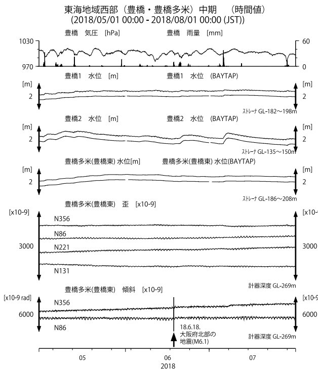
第7図 東海地域西部(豊橋・豊橋多米)の地下水等の観測結果(2018年5月～2018年7月) Fig. 7 Observed groundwater levels and others at the Toyohashi and Toyohashi-tame observation sites in the western Tokai district from May 2018 to Jul. 2018.
