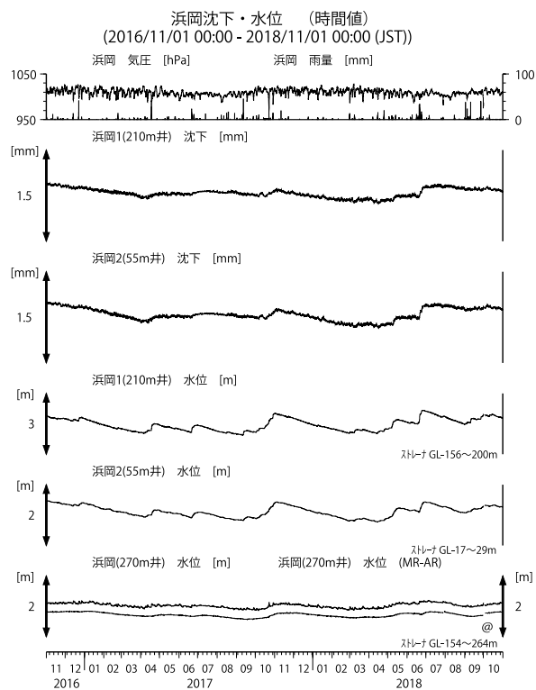
第21図 浜岡における沈下等の観測結果(2016年11月~2018年10月) Fig. 21 Observed subsidence data and others at the Hamaoka observation well from Nov. 2016 to Oct. 2018.
