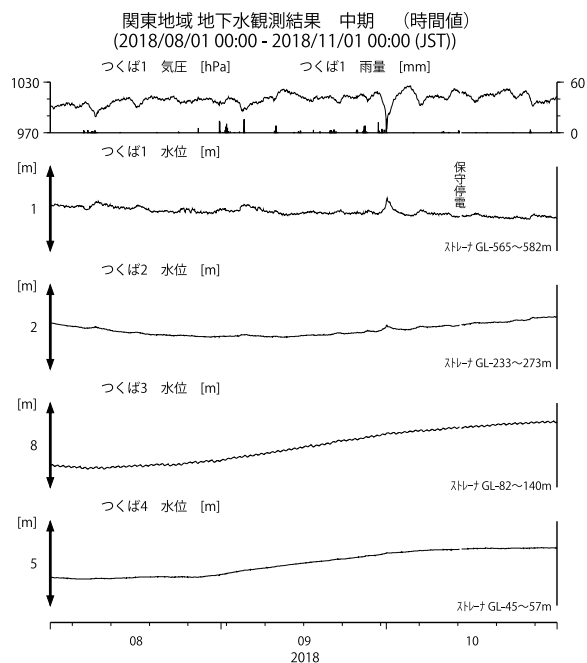
第14図 関東地域の地下水等の観測結果(2018年8月～2018年10月) Fig. 14 Observed groundwater levels and others in the Kanto district from Aug. 2018 to Oct. 2018.
