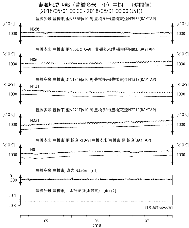
第9図 東海地域西部(豊橋多米)の歪等の観測結果(2018年5月～2018年7月) Fig. 9 Observed strain and others at the Toyohashi-tame observation site in the western Tokai district from May 2018 to Jul. 2018.
