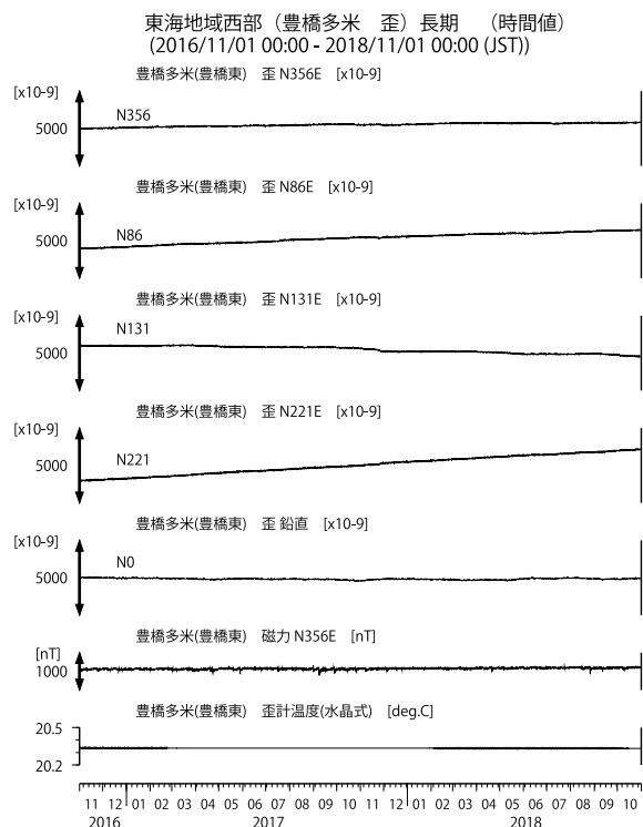
第18図 東海地域西部(豊橋多米)の歪等の観測結果(2016年11月～2018年10月)
