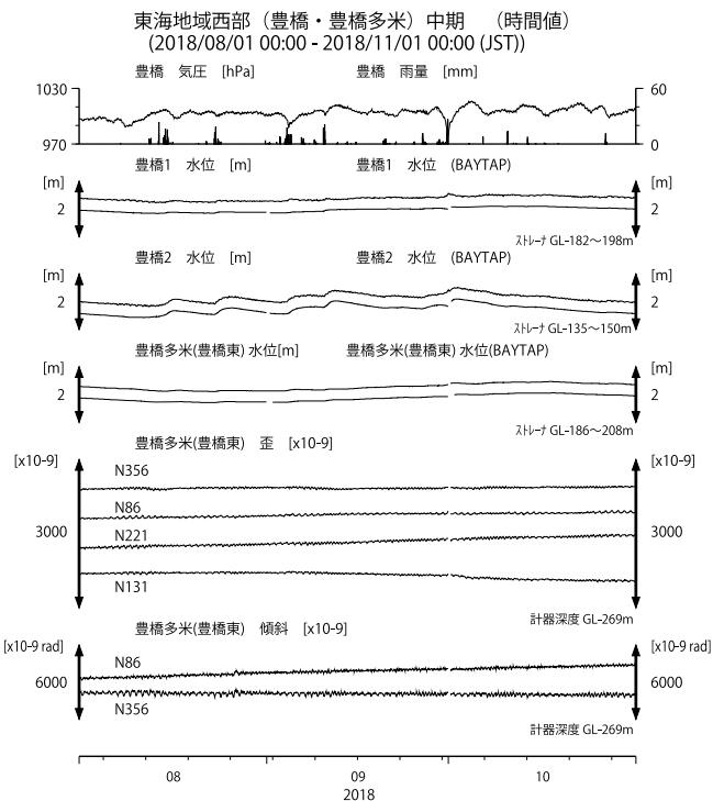
第8図 東海地域西部(豊橋・豊橋多米)の地下水等の観測結果(2018年8月～2018年10月) Fig. 8 Observed groundwater levels and others at the Toyohashi and Toyohashi-tame observation sites in the western Tokai district from Aug. 2018 to Oct. 2018.
