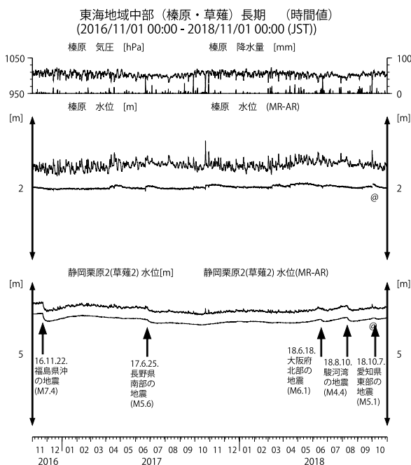
第15図 東海地域中部の地下水等の観測結果(2016年11月～2018年10月) Fig. 15 Observed groundwater levels and others in the central Tokai district from Nov. 2016 to Oct. 2018.
