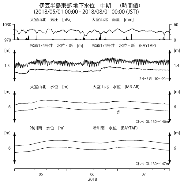
第11図 伊豆半島東部の地下水等の観測結果(2018年5月～2018年7月) Fig. 11 Observed groundwater levels and others in the eastern Izu peninsula district from May 2018 to Jul. 2018.
