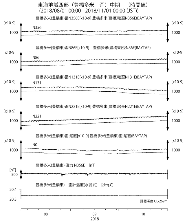
第10図 東海地域西部(豊橋多米)の歪等の観測結果(2018年8月～2018年10月) Fig. 10 Observed strain and others at the Toyohashi-tame observation site in the western Tokai district from Aug. 2018 to Oct. 2018.
