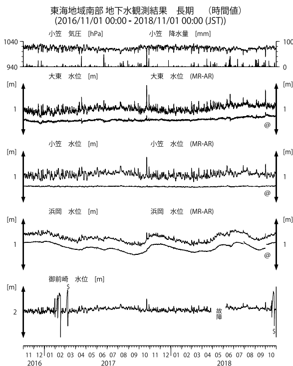
第16図 東海地域南部の地下水等の観測結果(2016年11月～2018年10月) Fig. 16 Observed groundwater levels and others in the southern Tokai district from Nov. 2016 to Oct. 2018.
