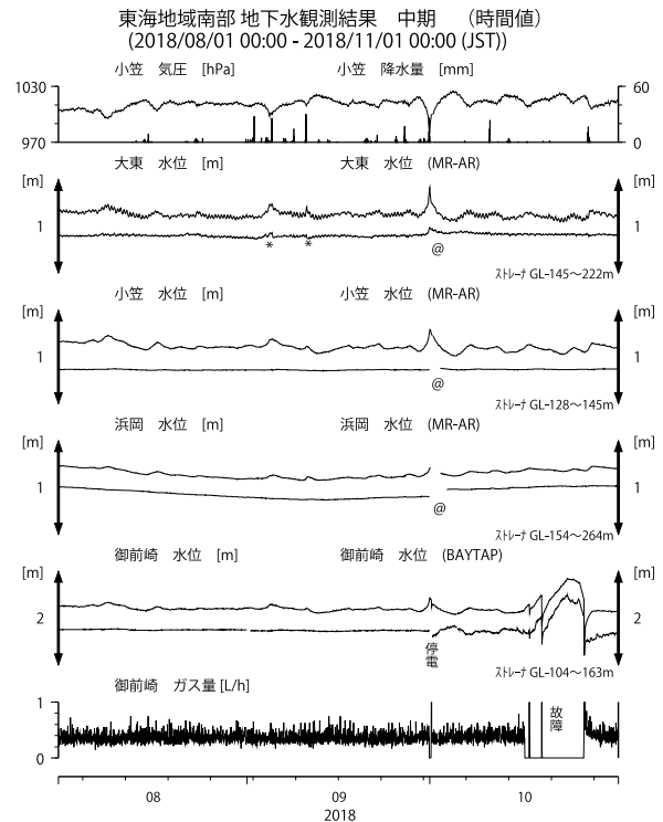
第6図 東海地域南部の地下水等の観測結果(2018年8月～2018年10月) Fig. 6 Observed groundwater levels and others in the southern Tokai district from Aug. 2018 to Oct. 2018.
