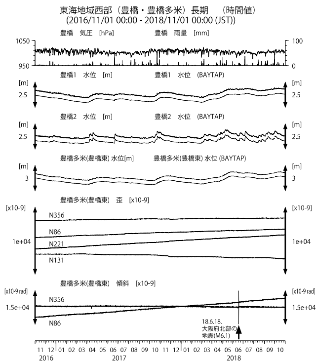
第17図 東海地域西部(豊橋・豊橋多米)の地下水等の観測結果(2016年11月～2018年10月)
