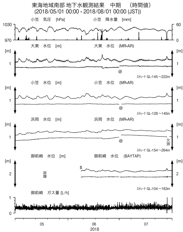
第5図 東海地域南部の地下水等の観測結果(2018年5月～2018年7月) Fig. 5 Observed groundwater levels and others in the southern Tokai district from May 2018 to Jul. 2018.
