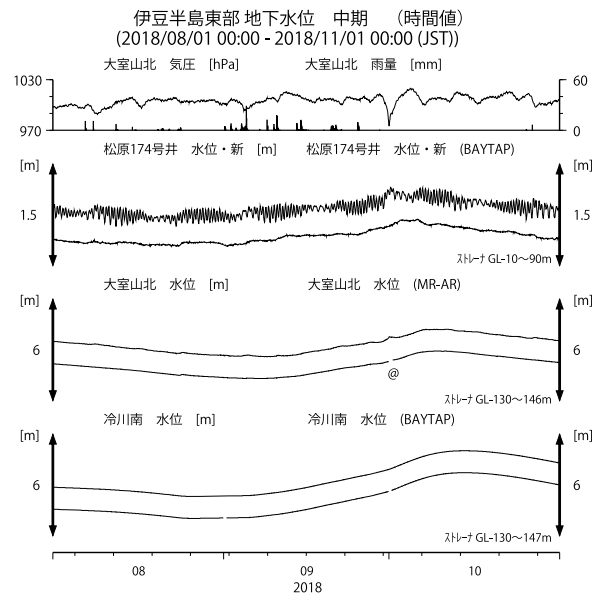
第12図 伊豆半島東部の地下水等の観測結果(2018年8月～2018年10月) Fig. 12 Observed groundwater levels and others in the eastern Izu peninsula district from Aug. 2018 to Oct. 2018.
