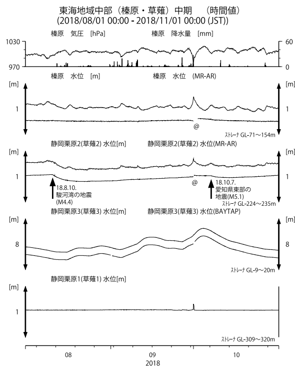
第4図 東海地域中部の地下水等の観測結果(2018年8月～2018年10月) Fig. 4 Observed groundwater levels and others in the central Tokai district from Aug. 2018 to Oct. 2018.
