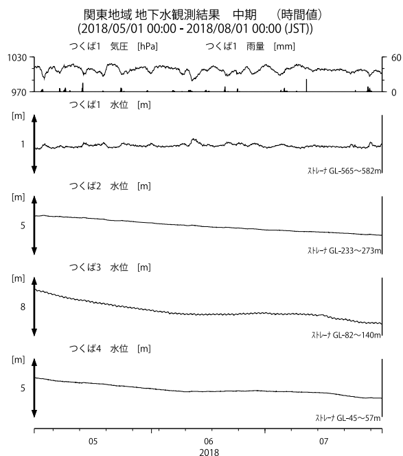
第13図 関東地域の地下水等の観測結果(2018年5月～2018年7月) Fig. 13 Observed groundwater levels and others in the Kanto district from May 2018 to Jul. 2018.
