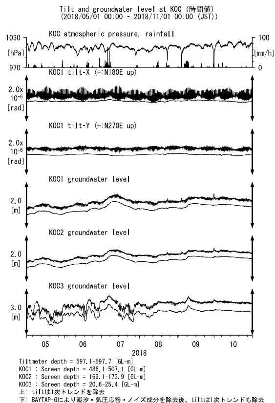
第 26 図 KOC における傾斜・地下水位観測結果 (2018 年 5 月～2018 年 10 月)
