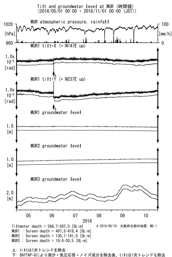
第 24 図 MUR における傾斜・地下水位観測結果 (2018 年 5 月～2018 年 10 月)
