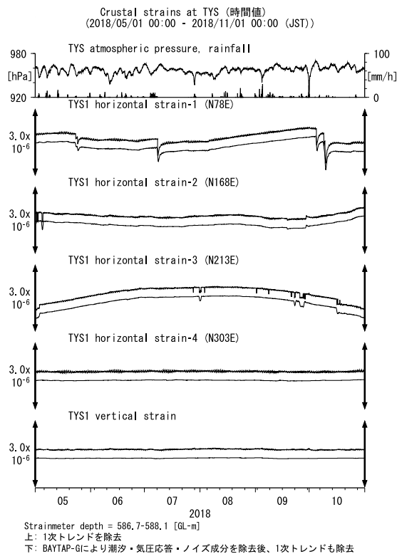
第2図 TYSにおける歪観測結果 (2018年5月～2018年10月) Fig. 2 Observed strains at the TYS observation site from May 2018 to October 2018.
