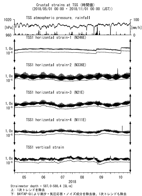
第 29 図 TSS における歪観測結果 (2018 年 5 月～2018 年 10 月)
