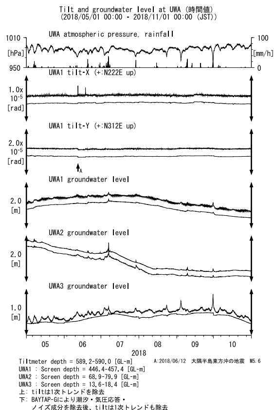
第32図 UWAにおける傾斜・地下水位観測結果 (2018年5月～2018年10月)
