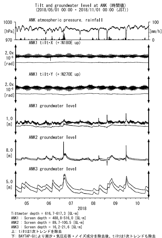
第 22 図 ANK における傾斜・地下水位観測結果 (2018 年 5 月～2018 年 10 月)
