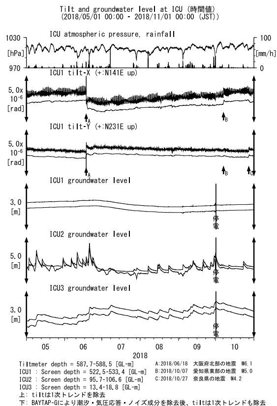
第 15 図 ICU における傾斜・地下水位観測結果 (2018 年 5 月～2018 年 10 月) Fig. 15 Observed tilts and groundwater levels at the ICU observation site from May 2018 to October 2018.
