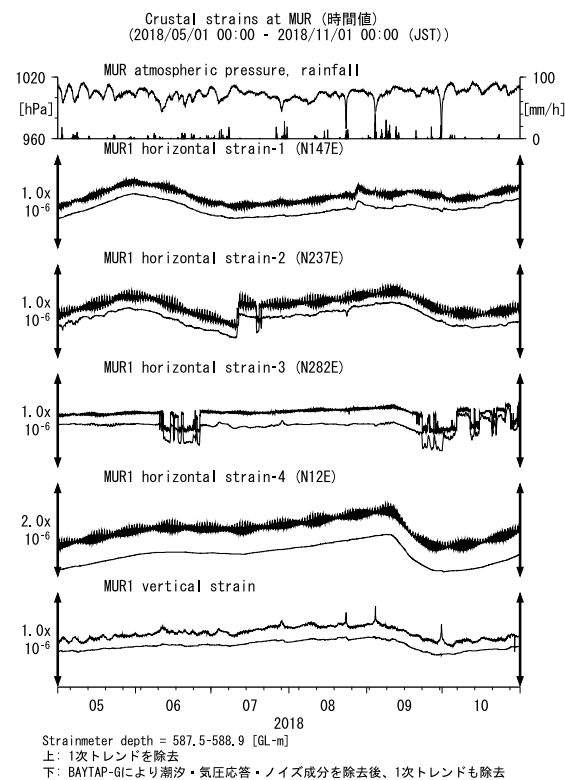
第 23 図 MUR における歪観測結果 (2018 年 5 月～2018 年 10 月)
