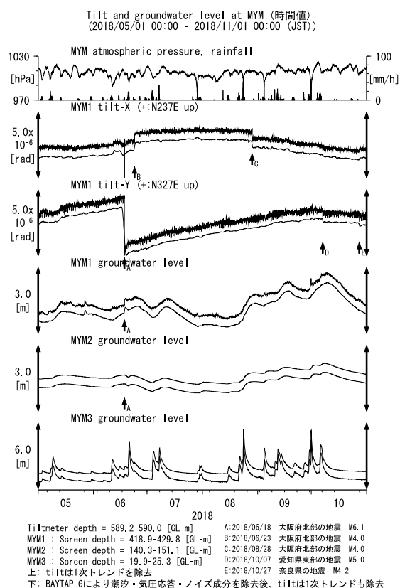
第 13 図 MYM における傾斜・地下水位観測結果 (2018 年 5 月～2018 年 10 月) Fig. 13 Observed tilts and groundwater levels at the MYM observation site from May 2018 to October 2018.
