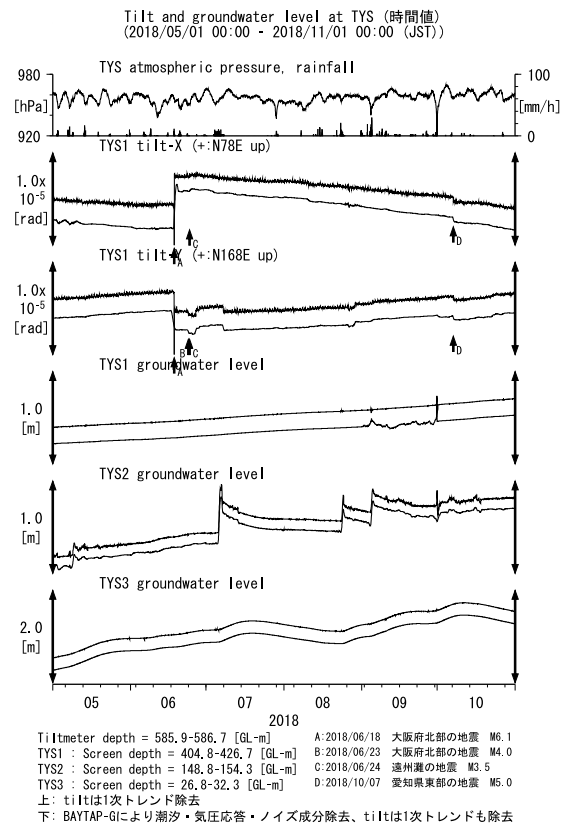
第3図 TYSにおける傾斜・地下水位観測結果 (2018年5月～2018年10月) Fig. 3 Observed tilts and groundwater levels at the TYS observation site from May 2018 to October 2018.
