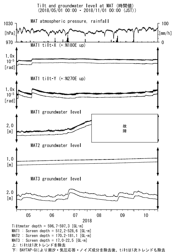
第 34 図 MAT における傾斜・地下水位観測結果 (2018 年 5 月～2018 年 10 月)
