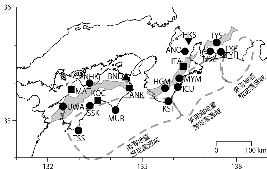
第1図 地下水等総合観測点の分布図 (●, ■, ▲, ▼). 観測点の一覧は第1表に示す. ●はデジタル方式の石井式歪計・傾斜計を併設している新規観測点, ■はGladwin式歪計・ミツトヨ式傾斜計を併設している新規観測点, ▲はアナログ方式の石井式歪計を併設している既存の観測点, ▼は既存の地下水観測点. 灰色の領域は短期的SSE及び深部低周波微動が定常的に発生していると考えられる地域.
