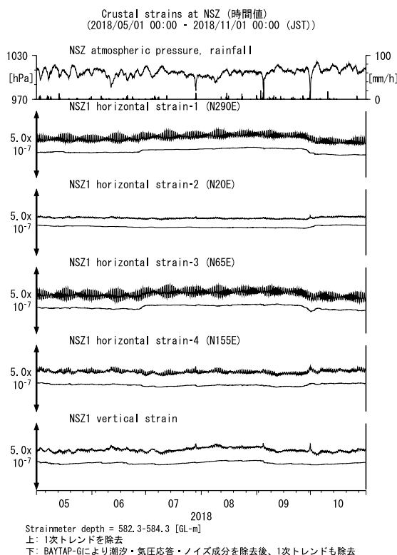
第4図 NSZにおける歪観測結果 (2018年5月～2018年10月) Fig. 4 Observed strains at the NSZ observation site from May 2018 to October 2018.
