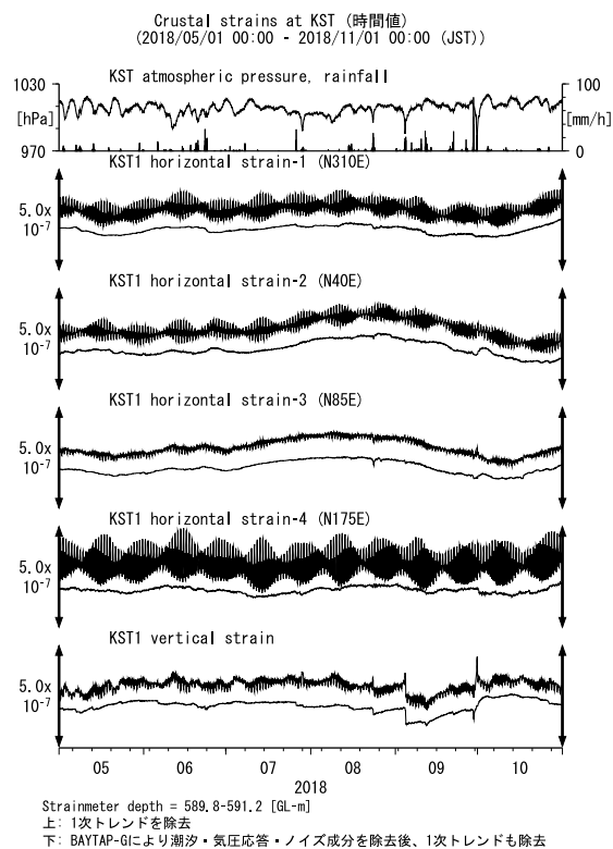
第18図 KSTにおける歪観測結果 (2018年5月~2018年10月) Fig. 18 Observed strains at the KST observation site from May 2018 to October 2018.
