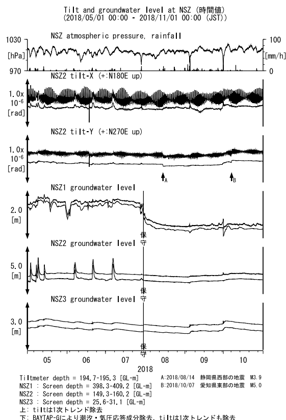
第5図 NSZにおける傾斜・地下水位観測結果 (2018年5月～2018年10月) Fig. 5 Observed tilts and groundwater levels at the NSZ observation site from May 2018 to October 2018.
