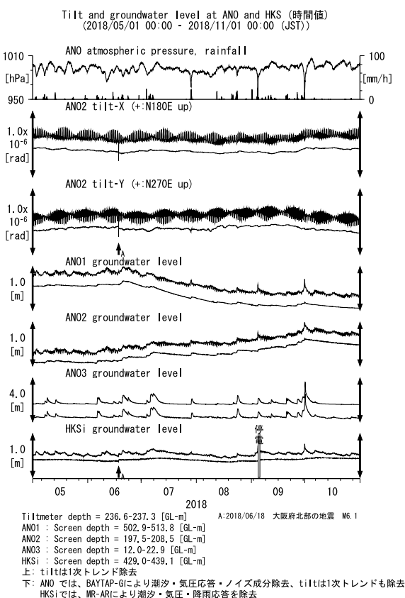
第9図 ANOおよびHKSにおける傾斜・地下水位観測結果 (2018年5月～2018年10月) Fig. 9 Observed tilts and groundwater levels at the ANO and the HKS observation site from May 2018 to October 2018.
