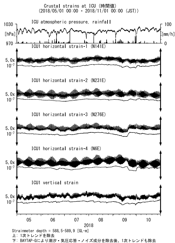
第 14 図 ICU における歪観測結果 (2018 年 5 月～2018 年 10 月) Fig. 14 Observed strains at the ICU observation site from May 2018 to October 2018.
