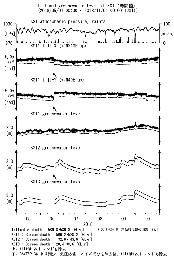
第19図 KSTにおける傾斜・地下水位観測結果 (2018年5月~2018年10月) Fig. 19 Observed tilts and groundwater levels at the KST observation site from May 2018 to October 2018.
