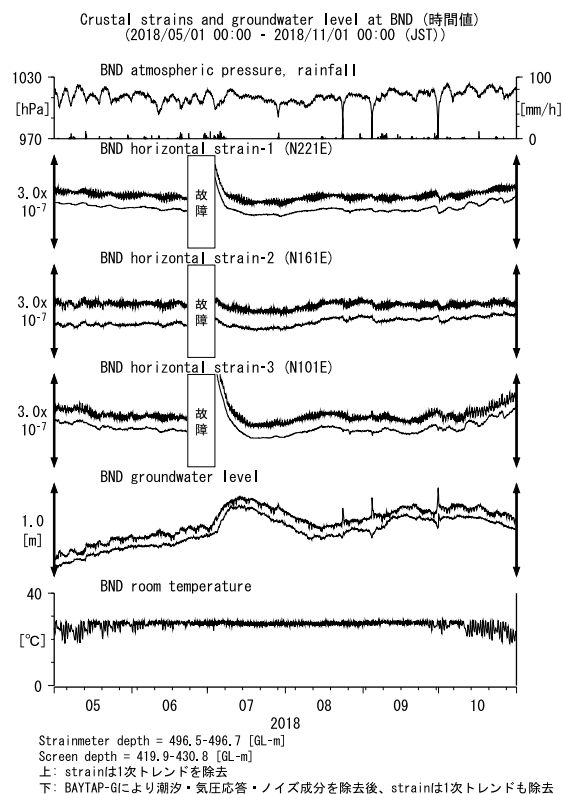
第20図 BNDにおける歪・地下水位観測結果 (2018年5月~2018年10月) Fig. 20 Observed strains and groundwater level at the BND observation site from May 2018 to October 2018.
