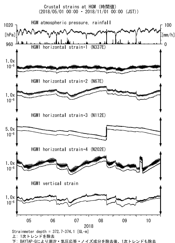
第 16 図 HGM における歪観測結果 (2018 年 5 月～2018 年 10 月) Fig. 16 Observed strains at the HGM observation site from May 2018 to October 2018.
