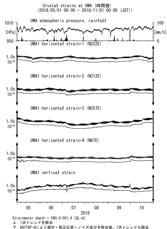
第31図 UWAにおける歪観測結果 (2018年5月～2018年10月) Fig. 31 Observed strains at the UWA observation site from May 2018 to October 2018.
