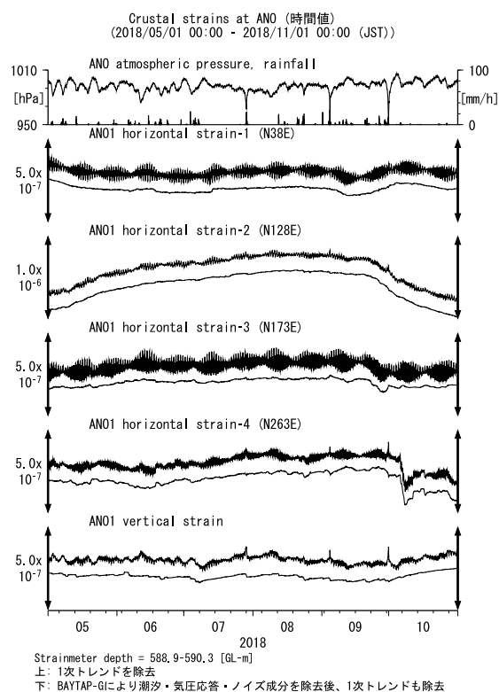
第8図 ANOにおける歪観測結果 (2018年5月～2018年10月) Fig. 8 Observed strains at the ANO observation site from May 2018 to October 2018.
