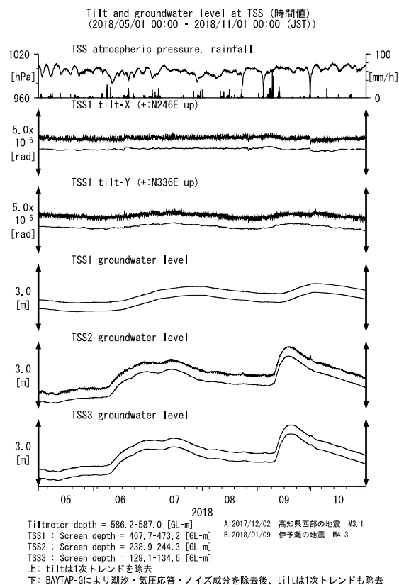
第30図 TSSにおける傾斜・地下水位観測結果 (2018年5月～2018年10月)
