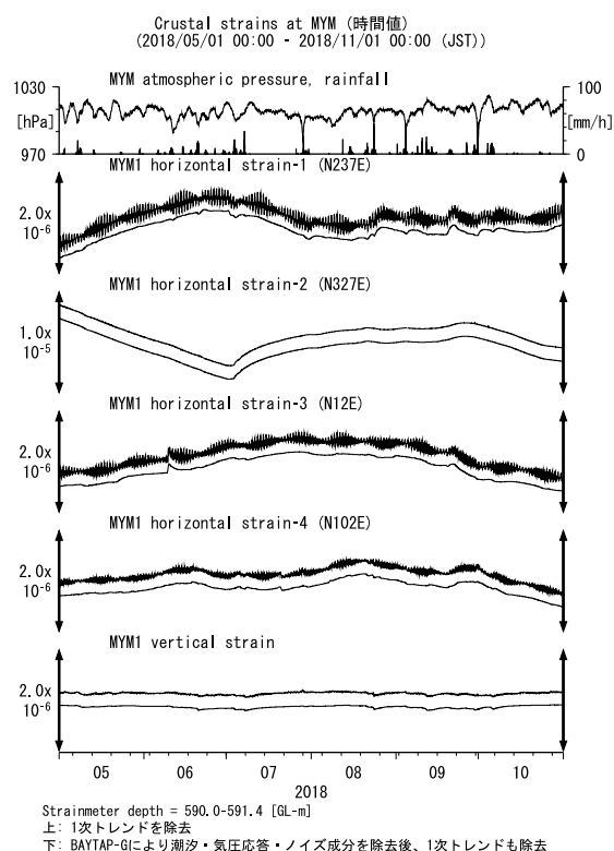
第 12 図 MYM における歪観測結果 (2018 年 5 月～2018 年 10 月) Fig. 12 Observed strains at the MYM observation site from May 2018 to October 2018.
