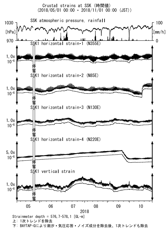
第 27 図 SSK における歪観測結果 (2018 年 5 月～2018 年 10 月)
