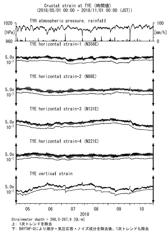
第6図 TYEにおける歪観測結果 (2018年5月～2018年10月) Fig. 6 Observed strains at the TYE observation site from May 2018 to October 2018.
