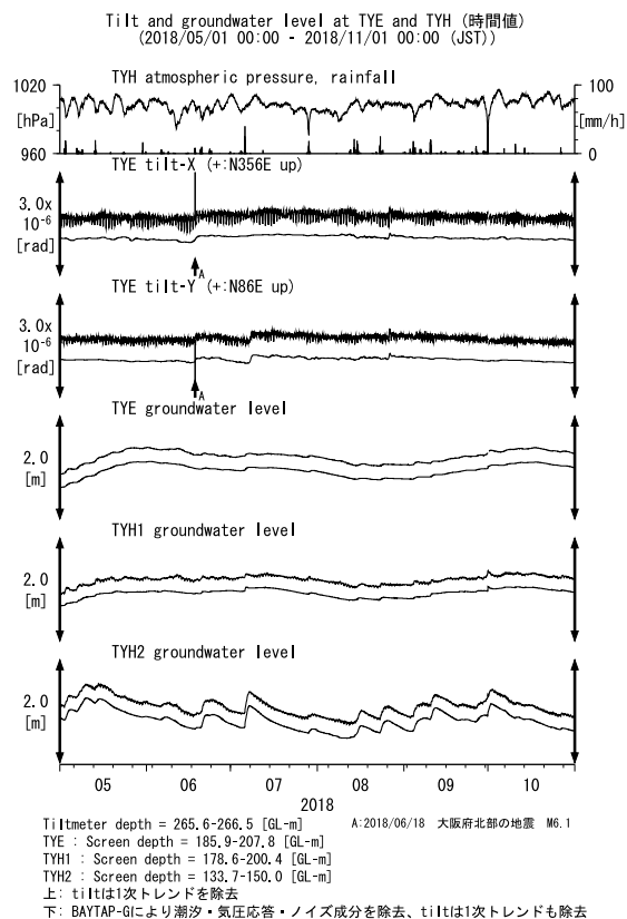
第7図 TYEおよびTYHにおける傾斜・地下水位観測結果 (2018年5月～2018年10月) Fig. 7 Observed tilts and groundwater levels at the TYE and the TYH observation site from May 2018 to October 2018.
