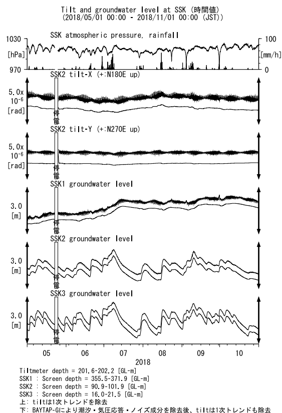
第 28 図 SSK における傾斜・地下水位観測結果 (2018 年 5 月～2018 年 10 月)
