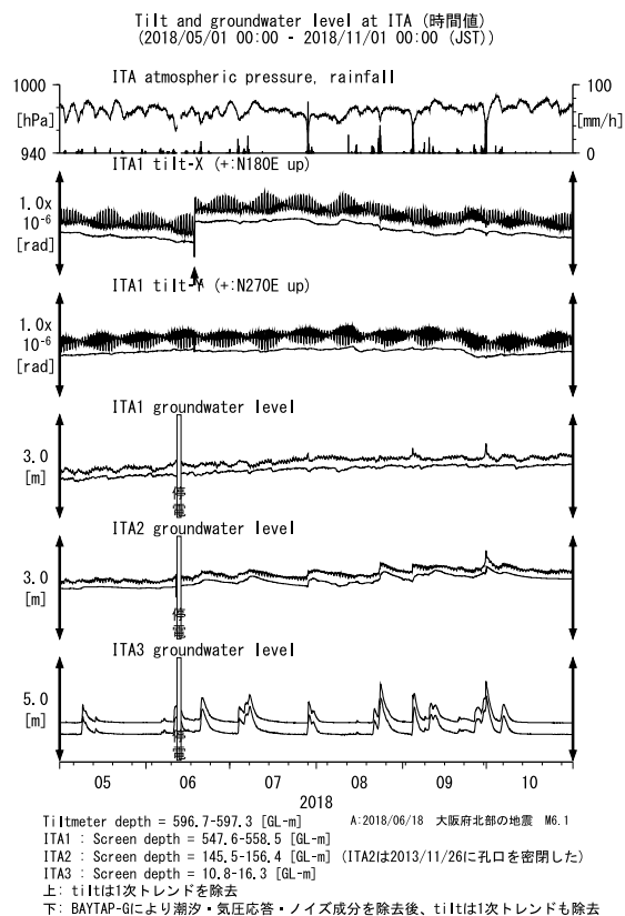
第 11 図 ITA における傾斜・地下水位観測結果 (2018 年 5 月～2018 年 10 月) Fig. 11 Observed tilts and groundwater levels at the ITA observation site from May 2018 to October 2018.
