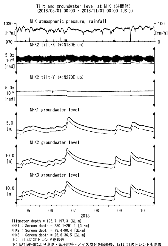
第 36 図 NHK における傾斜・地下水位観測結果 (2018 年 5 月～2018 年 10 月)
