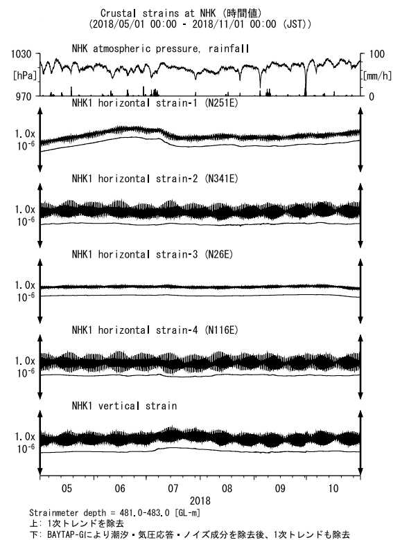
第 35 図 NHK における歪観測結果 (2018 年 5 月～2018 年 10 月)
