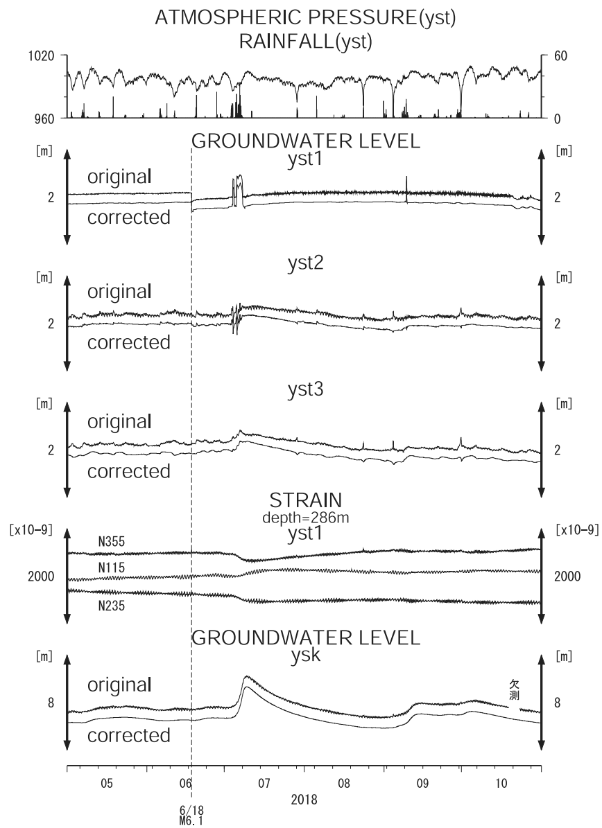
第2図 yst1, yst2, yst3, ysk の2018年5月～2018年10月の観測結果. Fig. 2 Observation results at yst1, yst2, yst3 and ysk from May 2018 to October 2018.
