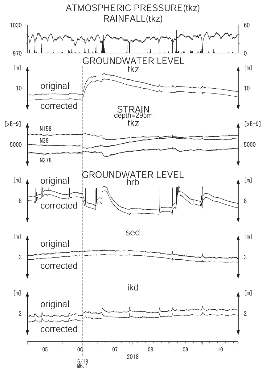
第3図 tkz, hrb, sed, ikd の2018年5月～2018年10月の観測結果. Fig. 3 Observation results at tkz, hrb, sed and ikd from May 2018 to October 2018.
