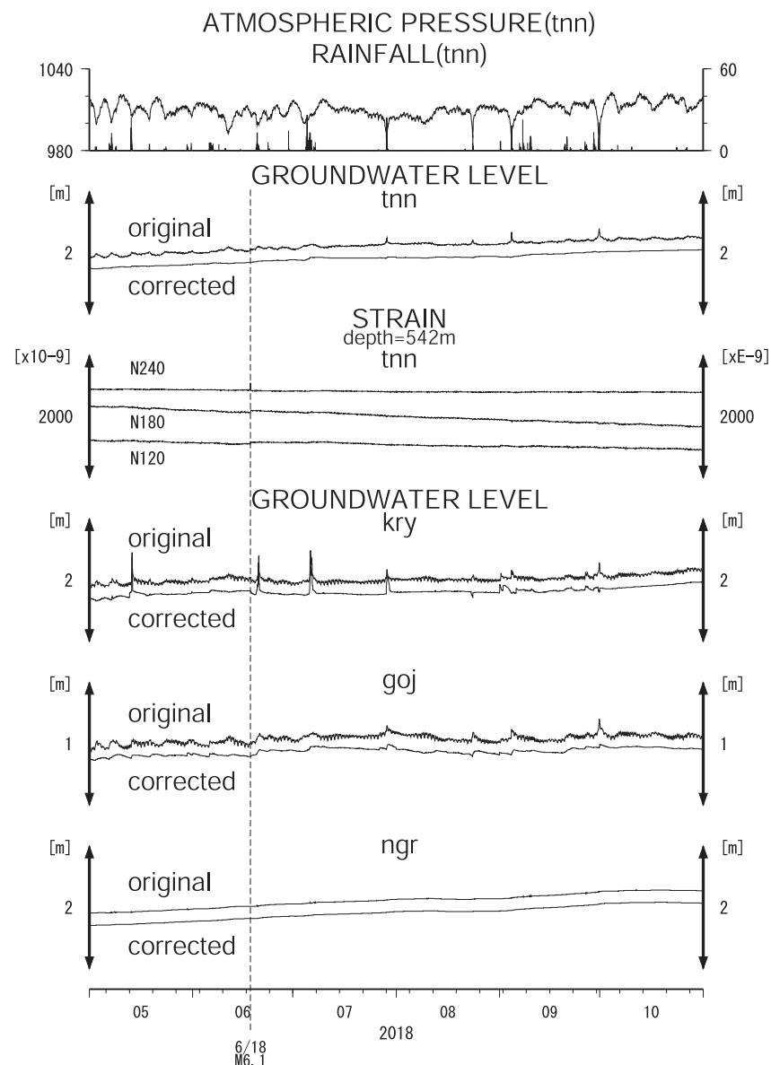
第4図 tnn, kry, goj の2018年5月～2018年10月の観測結果。 Fig. 4 Observation results at tnn, kry and goj from May 2018 to October 2018.
