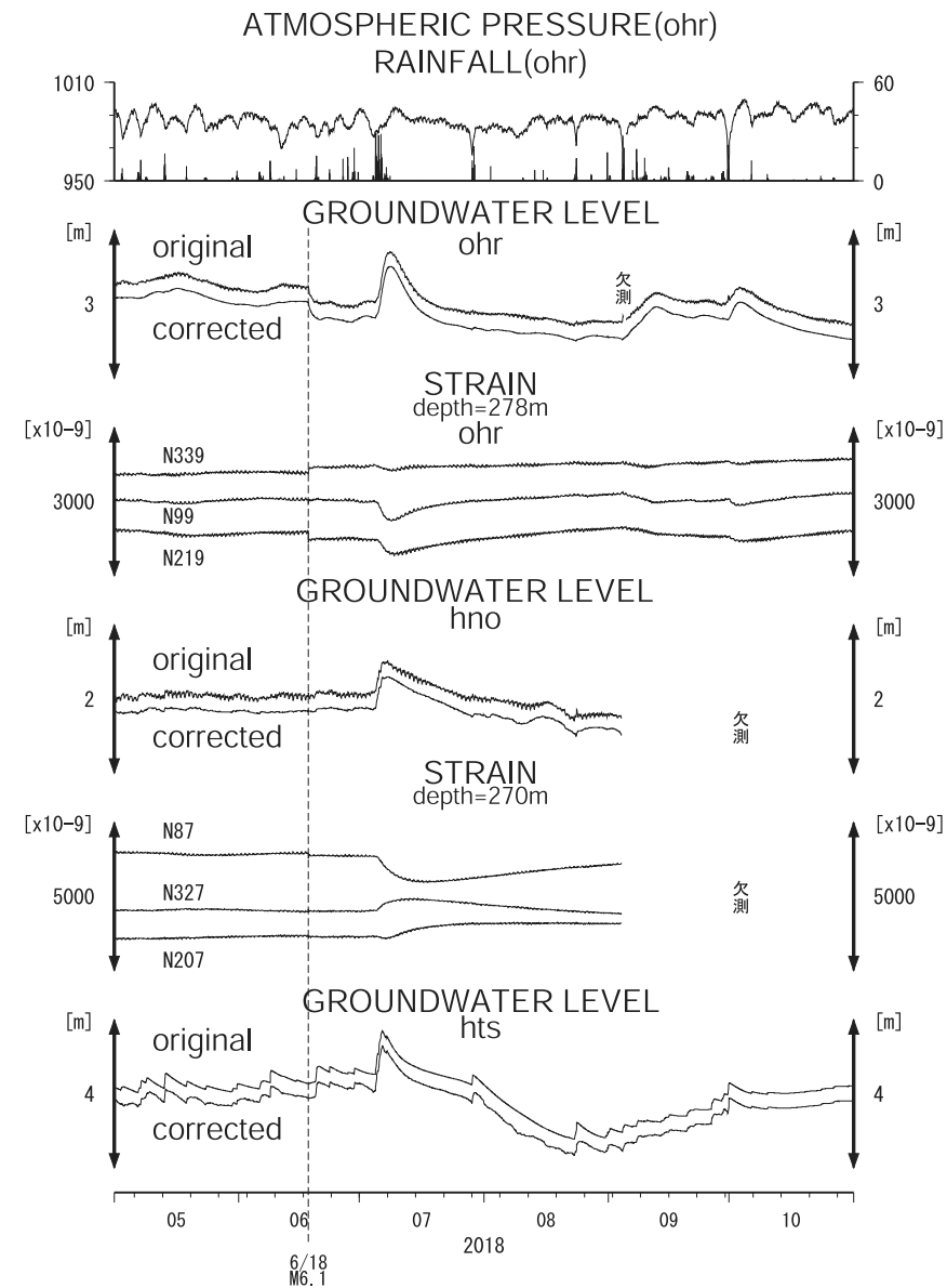
第5図 ohr, hno, hts-i の地下水水位・地殻歪の2018年5月～2018年10月の観測結果。 Fig. 5 Observation results at ohr, hno and hts-i from May 2018 to October 2018.
