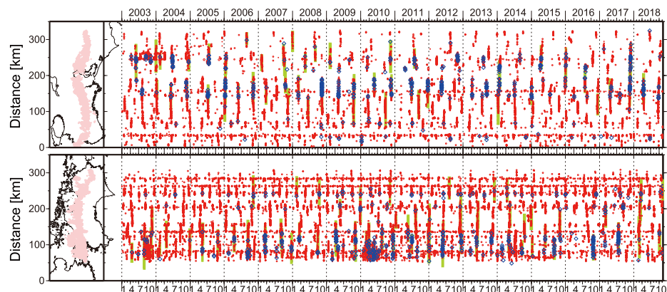
第 3 図 西南日本で発生した深部低周波微動（赤丸）及び深部超低周波地震（青菱形）の 2003 年から約 16 年間の時空間分布. 黄緑色太線は、傾斜変動から検出された短期的スロースリップイベントを示す.
