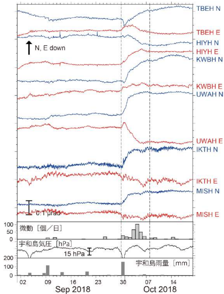
第2図 2018年9月1日から10月19日までの傾斜時系列。観測点位置は第3図に示した。記録は上方向への変化が北・東下りの傾斜変動を表す。気圧応答・潮汐成分をBAYTAP-G4)により除去し、直線トレンドを補正した後の記録を示した。9月30日～10月7日の傾斜変化量をSSEによるものと仮定した。四国西部での微動活動度・気象庁宇和島観測点での気圧変化および雨量をあわせて表示した。
