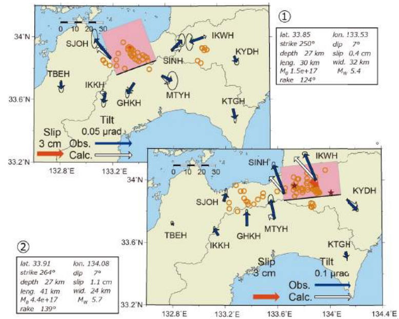
第5図 2018年10月～11月四国中東部のSSEの断層モデル。図の見方は第3図と同じ。 Fig. 5 Same as Fig. 3 but for the October-November 2018 short-term SSE in the central and eastern Shikoku region.
