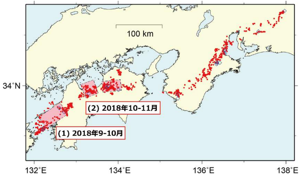
第1図 2018年5月1日～2018年11月7日の期間に検知された短期的SSE (ピンク矩形). 同期間に発生した深部低周波微動 (赤点) 及び VLFЕ の震央 (青菱形) を重ねて表示した.
