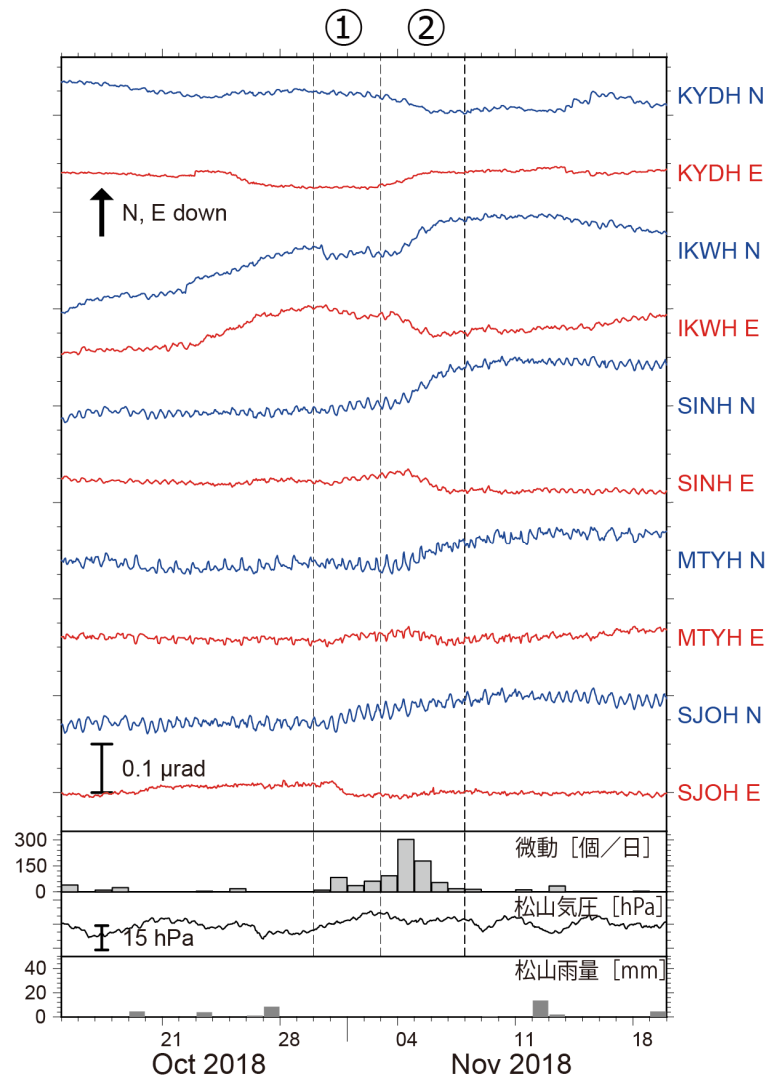
第4図 2018年10月15日から11月19日までの傾斜時系列。図の見方は第2図と同様。観測点位置は第5図に示した。期間①②の傾斜変化量をSSEによるものと仮定した。四国中東部における微動活動度・気象庁松山観測点での気圧変化および雨量をあわせて表示した。 Fig. 4 Same as Fig. 2 but for the records observed around Shikoku from October 15, 2018 to November 19, 2018. The tilt changes for the time windows indicated by the broken lines are assumed to be caused by an SSE. The atmospheric pressure and the precipitation were observed at the JMA Matsuyama meteorological observatory. The station locations and the tilt changes during the time windows indicated by broken lines are shown in Fig. 5.
