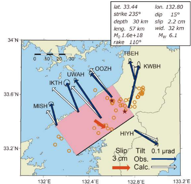
第3図 2018年10月～11月四国西部の短期的SSEの断層モデル。図2の破線で示された期間に観測された傾斜変化ベクトル(青矢印)・このデータから推定されたSSEの断層モデル(赤矩形・矢印)・モデルから計算される傾斜変化ベクトル(白抜き矢印)を示す。同じ期間の微動と深部超低周波地震の震央を橙円で示した。
