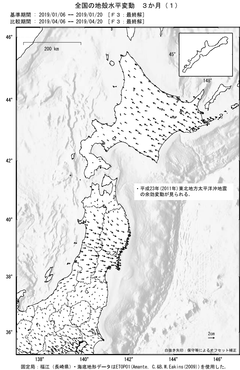
第4図 GNSS連続観測から求めた2019年1月～2019年4月の水平変動 Fig. 4 Horizontal displacements at GNSS sites during January 2019 – April 2019. (☆, Reference station is Fukue)
