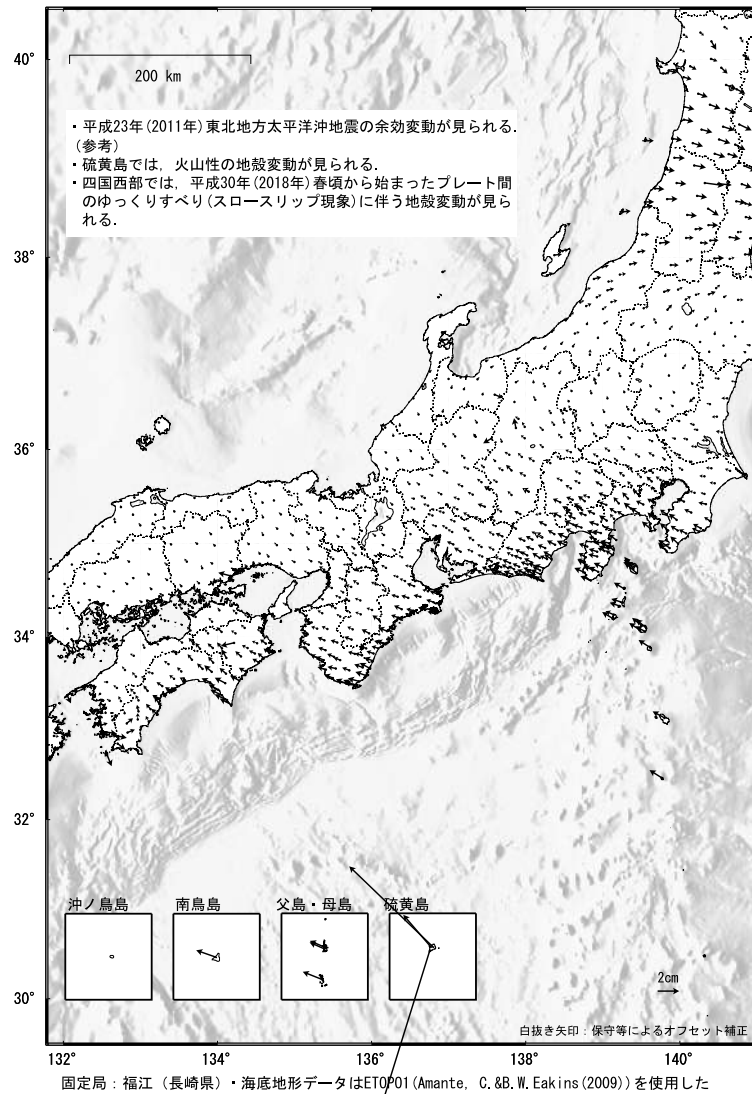
第5図 GNSS連続観測から求めた2019年1月～2019年4月の水平変動 Fig. 5 Horizontal displacements at GNSS sites during January 2019 – April 2019. (☆, Reference station is Fukue)
