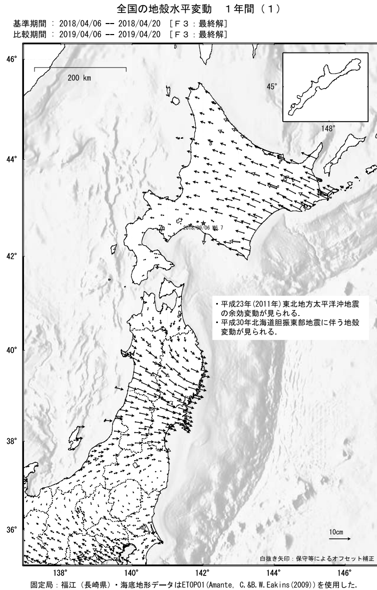
第1図 GNSS連続観測から求めた2018年4月～2019年4月の水平変動 Fig. 1 Annual horizontal displacement velocities at permanent GNSS sites during April 2018 – April 2019. (☆, Reference station is Fukue)
