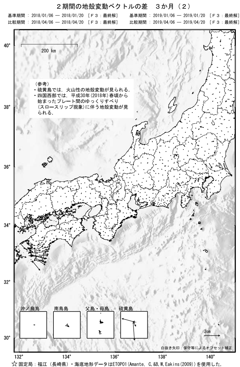
第 8 図 GNSS 水平変動の差 (3 ヶ月間)
