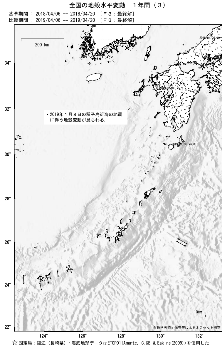
第3図 GNSS連続観測から求めた2018年4月～2019年4月の水平変動 Fig. 3 Annual horizontal displacement velocities at permanent GNSS sites during April 2018 – April 2019. (☆, Reference station is Fukue)
