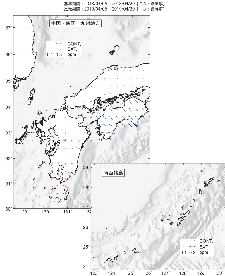
第12図 GNSS連続観測データから推定した中国・四国・九州及び南西諸島地方の水平歪 (2018年4月～2019年4月)
