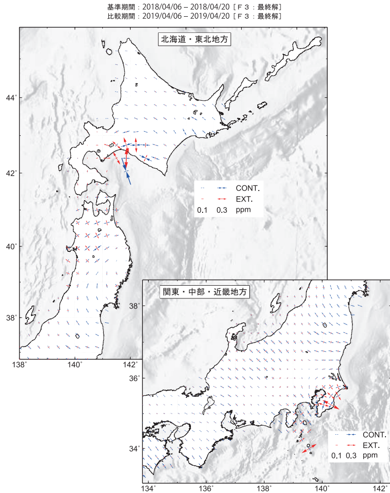
第11図 GNSS連続観測データから推定した北海道・東北および関東・中部・近畿地方の水平歪 (2018年4月～2019年4月)
