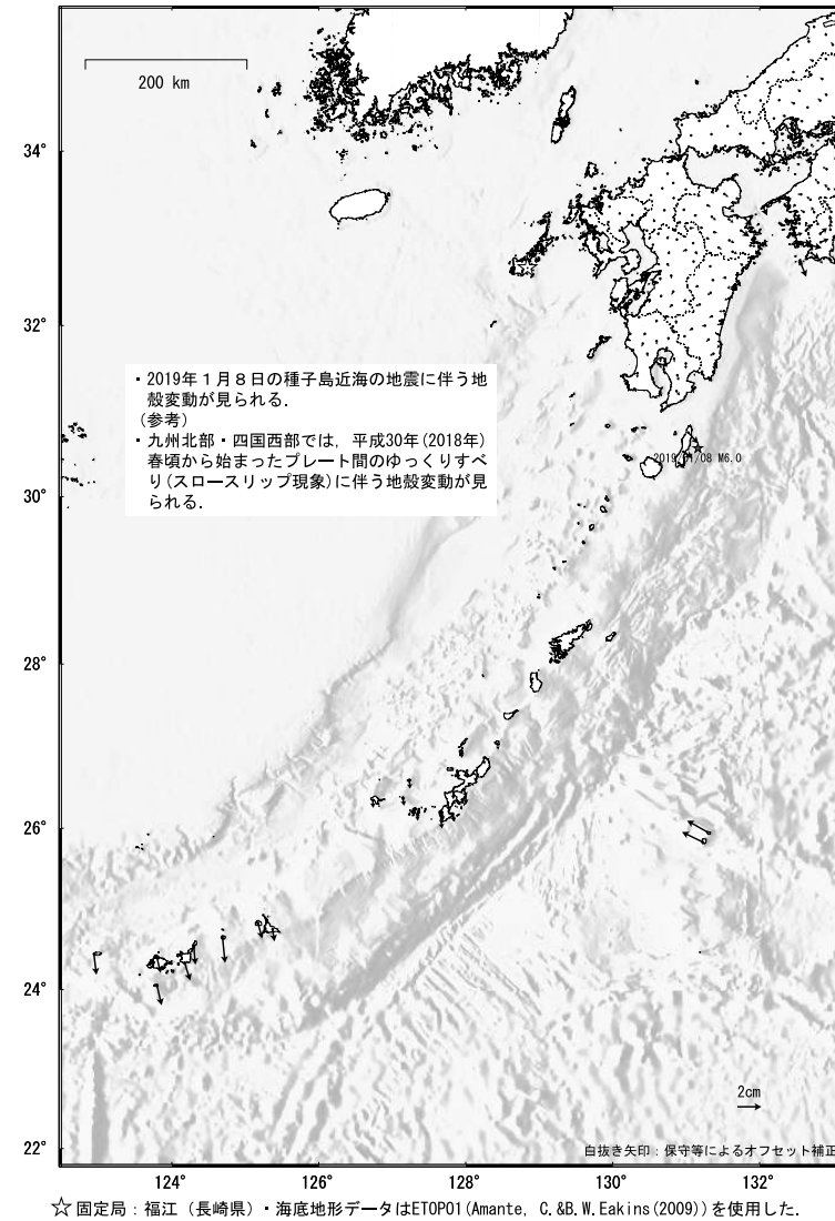
第6図 GNSS連続観測から求めた2019年1月～2019年4月の水平変動 Fig. 6 Horizontal displacements at GNSS sites during January 2019 – April 2019. (☆, Reference station is Fukue)
