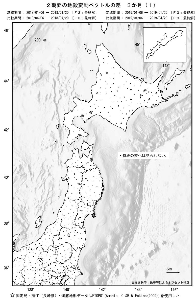
第 7 図 GNSS 水平変動の差 (3 ヶ月間)
