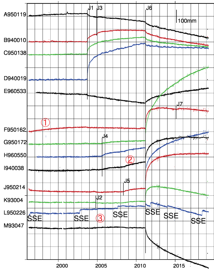
第2a図 プレート沈み込み方向の位置変化（東日本；1996年から2019年4月） 沈み込みと逆方向が上向き。地点番号は、第1図の観測点記号に GEONET 観測点番号を付加したもの。J1:2003年十勝沖地震(M8.0), J2:2004年新潟県中越地震(M6.8), J3:2004年11月29日釧路沖の地震(M7.1), J4:2005年8月16日宮城県沖の地震(M7.2), J5:2008年5月8日茨城県沖の地震(M7.0), J6:2011年東北地方太平洋沖地震(M9.0), J7:2015年2月17日三陸沖の地震(M6.9).
