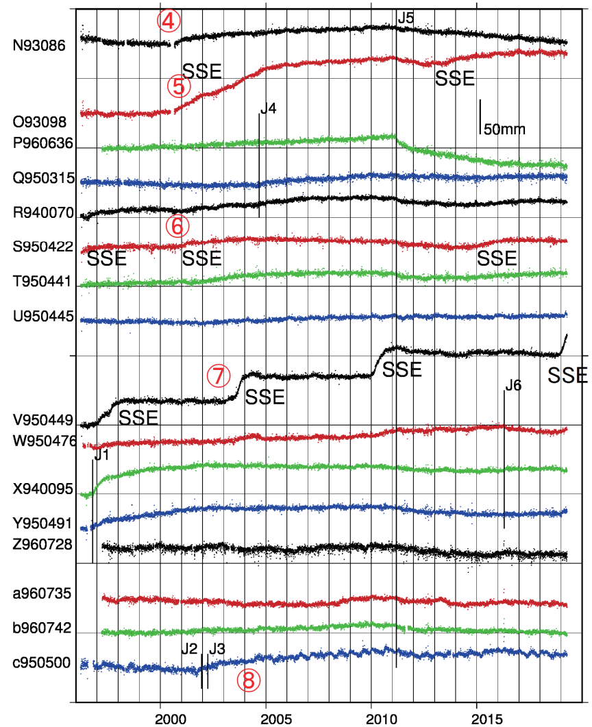
第2b図 プレート沈み込み方向の位置変化（西日本；1996年から2019年4月） 沈み込みと逆方向が上向き。地点番号は、第1図の観測点記号に GEONET 観測点番号を付加したもの。J1:1996年10月19日日向灘の地震(M6.9), J2:2001年12月18日与那国島近海(M7.3), J3:2002年3月31日台湾付近の地震(M7.2), J4:2004年9月5日三重県南東沖の地震(M7.4), J5:2011年東北地方太平洋沖地震(M9.0), J6:2016年熊本地震(M7.3).
