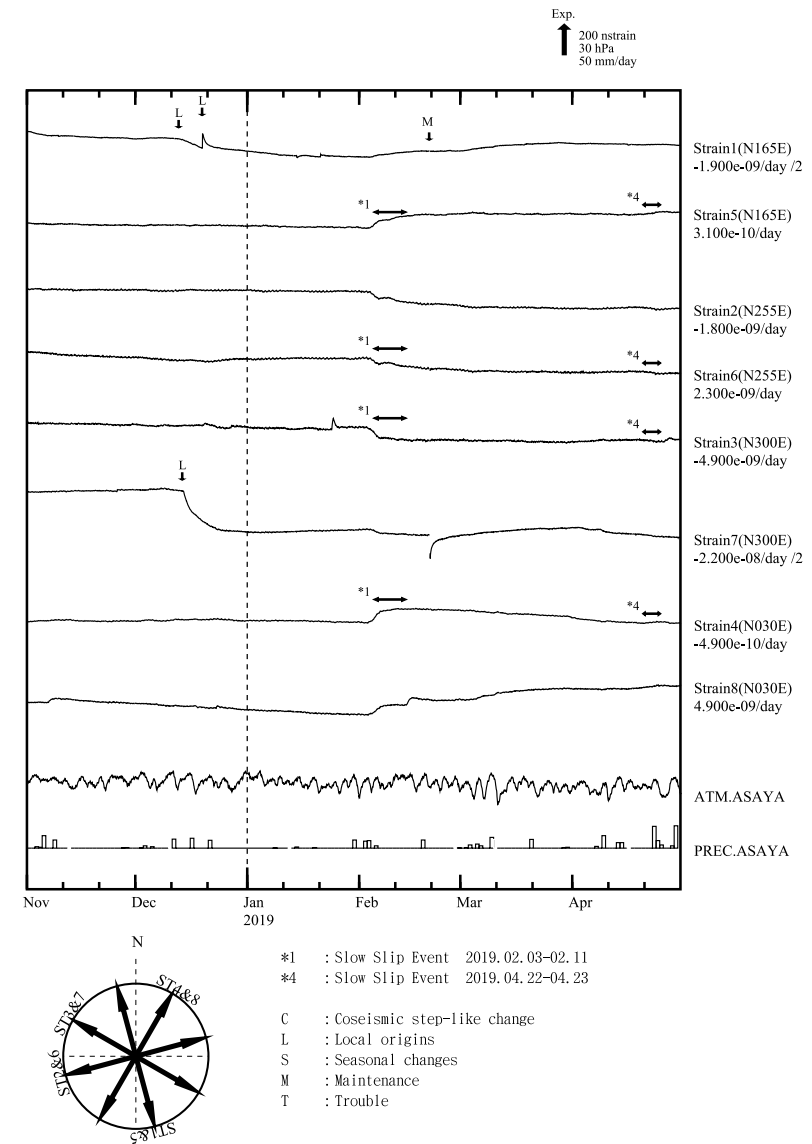
第4図(f)～(k) 左：2012年1月以後の多成分ひずみ計変化（日平均値）。主ひずみ・最大せん断ひずみ・面積ひずみは各方向成分から計算されている。 右：2018年11月～2019年4月の多成分ひずみ計変化（時間値：気圧・潮汐・地磁気補正した値）。各図下部に気圧変化と降水量を示す。
