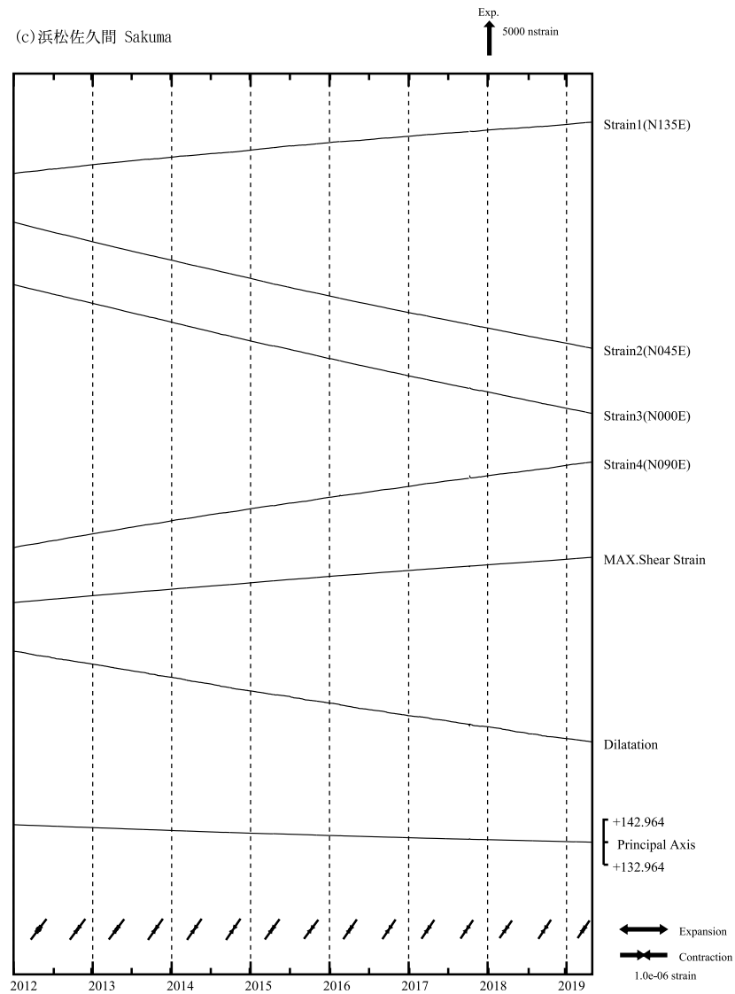
第4図(a)～(e) 左：2012年1月以後の多成分ひずみ計変化（日平均値）。主ひずみ・最大せん断ひずみ・面積ひずみは各方向成分から計算されている。 右：2018年11月～2019年4月の多成分ひずみ計変化（時間値：気圧・潮汐・地磁気・降水補正した値）。各図下部に気圧変化と降水量を示す。
