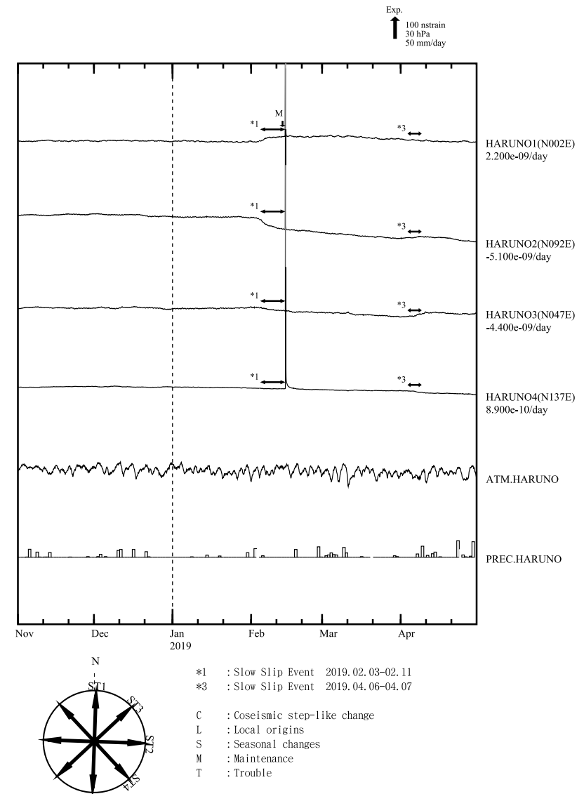
第4図(a)～(c) 左：2012年1月以後の多成分ひずみ計変化（日平均値）。主ひずみ・最大せん断ひずみ・面積ひずみは各方向成分から計算されている。 右：2018年11月～2019年4月の多成分ひずみ計変化（時間値：気圧・潮汐・地磁気・降水補正した値）。各図下部に気圧変化と降水量を示す。
