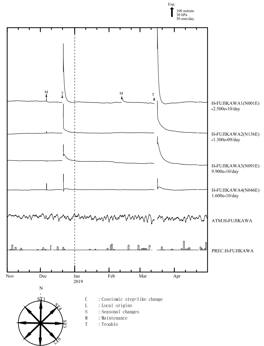
第4図(a)～(c) 左：2012年1月以後の多成分ひずみ計変化（日平均値）。主ひずみ・最大せん断ひずみ・面積ひずみは各方向成分から計算されている。 右：2018年11月～2019年4月の多成分ひずみ計変化（時間値：気圧・潮汐・地磁気・降水補正した値）。各図下部に気圧変化と降水量を示す。
