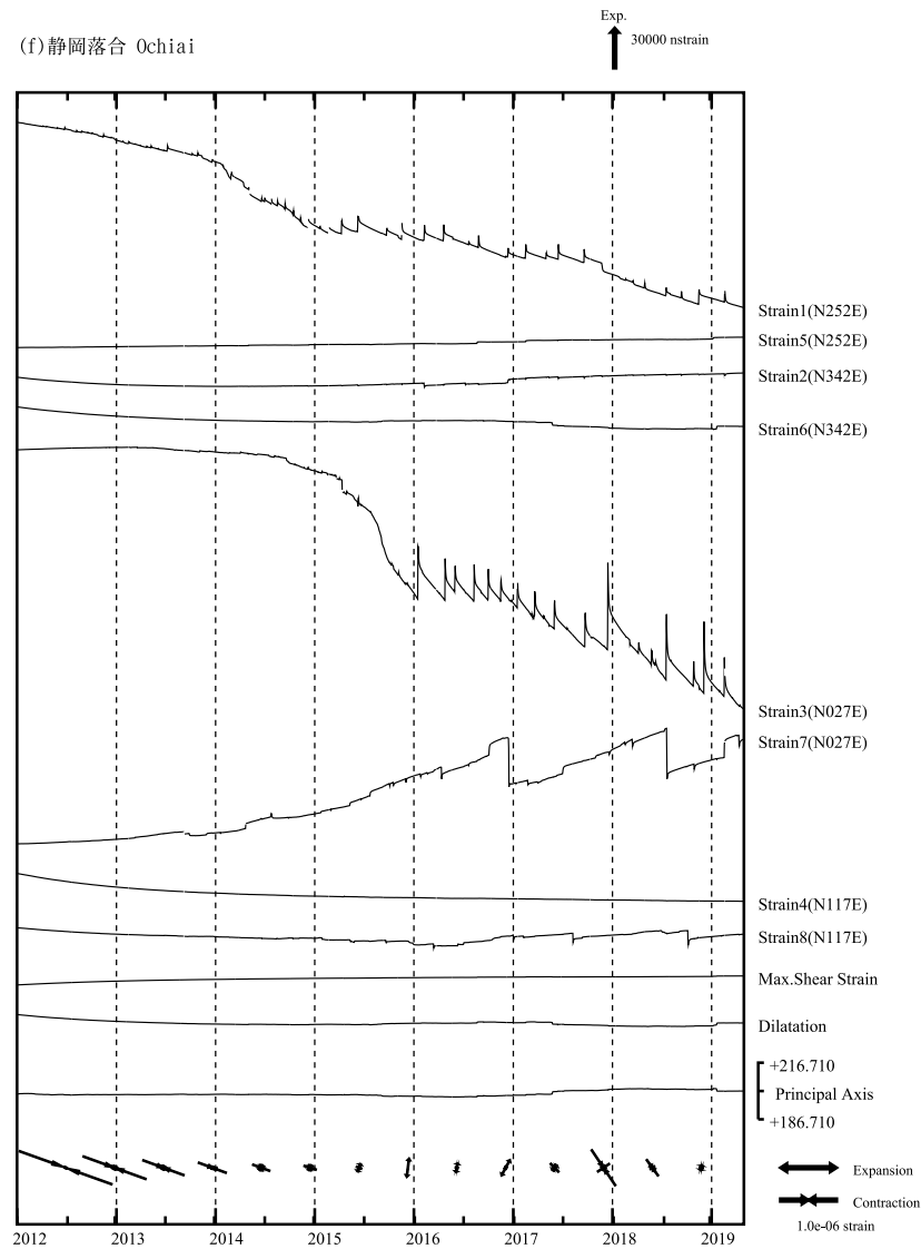
第4図(f)~(k) 左：2012年1月以後の多成分ひずみ計変化（日平均値）。主ひずみ・最大せん断ひずみ・面積ひずみは各方向成分から計算されている。 右：2018年11月～2019年4月の多成分ひずみ計変化（時間値：気圧・潮汐・地磁気補正した値）。各図下部に気圧変化と降水量を示す。
