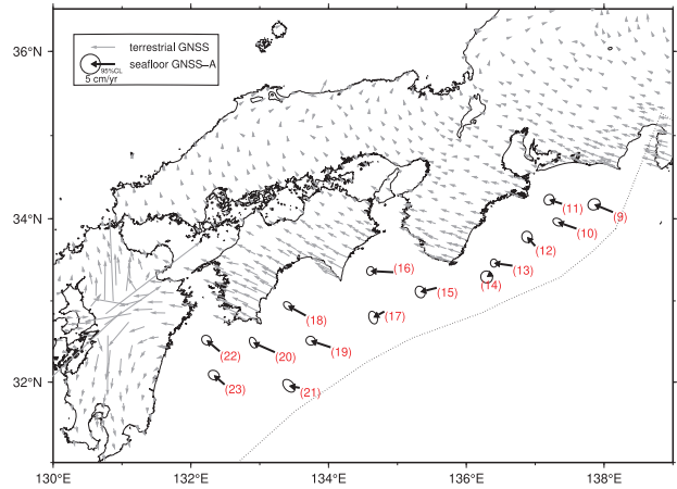
第 1 図 南海トラフ沿いの海底の水平地殻変動（直近約 4 年間の移動速度）【アムールプレート固定】
