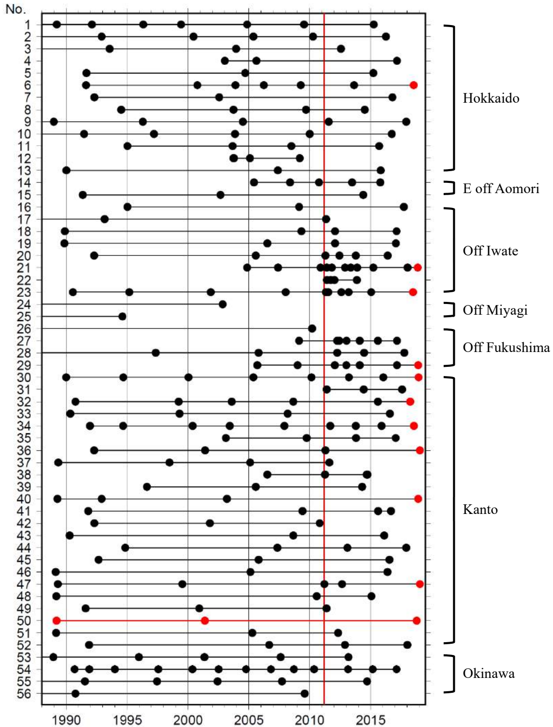
第 1 図 中規模相似地震活動経過図（～2019 年 1 月末）
