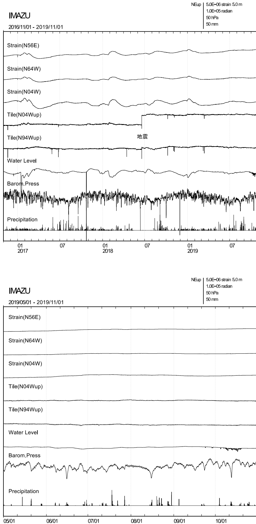
第2図 今津観測点における(上)2016年11月～2019年10月、(下)2019年5月～2019年10月のひずみ・傾斜変化(時間値)。毎年冬のひずみ・水位変化は、観測点付近の融雪のための地下水汲み上げに伴うもの。
