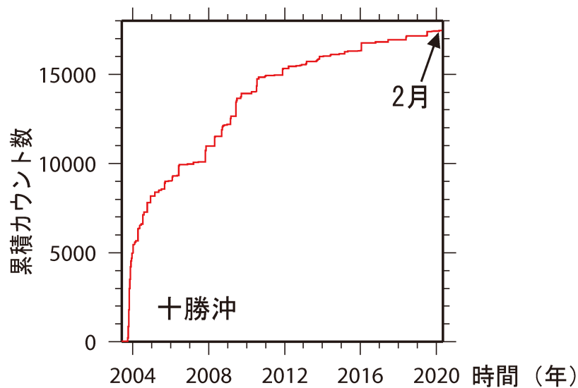
第 3 図 十勝沖における検出イベント累積カウンタ数の時間変化。
