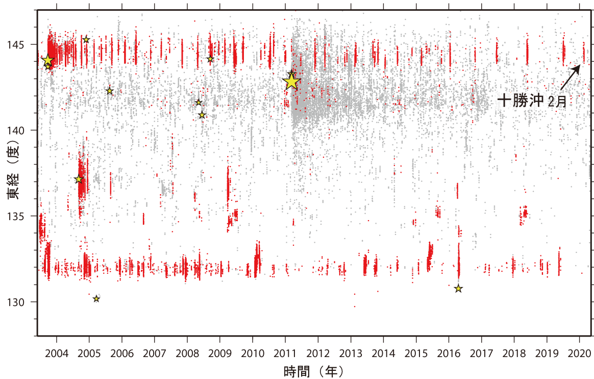
第 2 図 2003 年 6 月 1 日から 2020 年 4 月 30 日までの期間に検出されたイベントの時空間分布。検出されたイベントを防災科研 Hi-net 手動または自動検測震源と照合し、対応する地震が見出されたイベントを灰色丸印で、それ以外を赤色丸印で示す。
