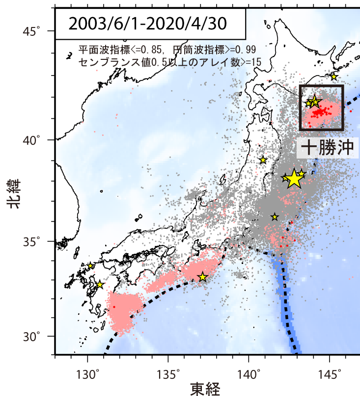
第 1 図 検出されたイベントの震央分布 (2003 年 6 月 1 日から 2020 年 4 月 30 日)。検出イベントを防災科研 Hi-net の手動または自動検測震源と照合し、対応する地震が見出されたイベントを灰色で、それ以外を桃色 (2019 年 10 月 31 日以前)、および赤色 (11 月 1 日以降) の点でそれぞれ示す。これらは主として周期 10 秒以上に卓越する超低周波地震を表すが、東北地方太平洋沖地震の発生以降は、除去しきれない通常の地震を多数含む。期間内に発生した M7 以上の地震の震央を黄色星印で併せて示す (ただし、2011 年 3 月 11 日以降の東日本は東北地方太平洋沖地震の本震のみ図示)。
