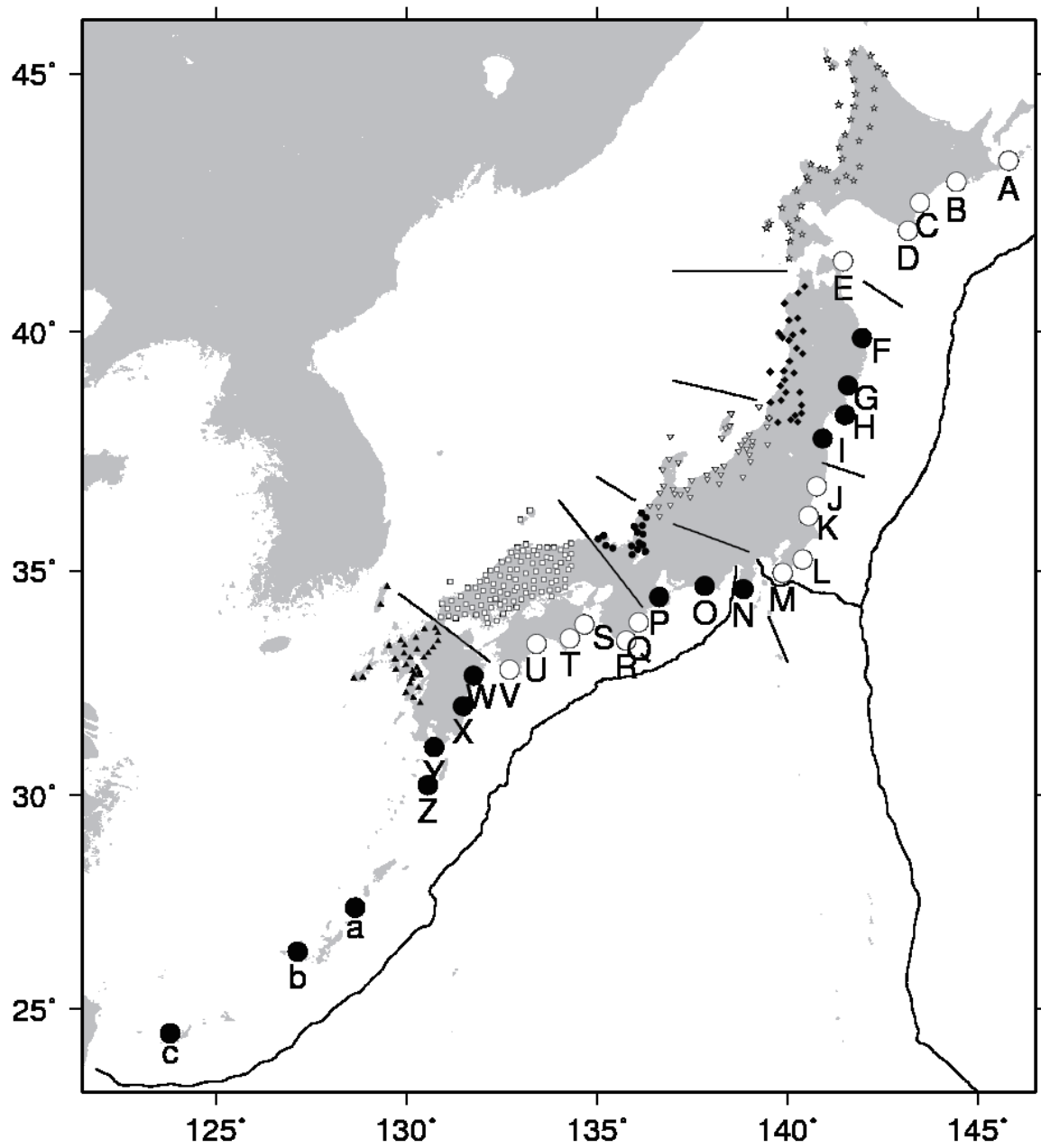
第 1 図 調査対象観測点 (A-Z, a-c) と領域固定に用いた観測点 Fig. 1 Observation points (A-Z, a-c) and points used for region fixing.
