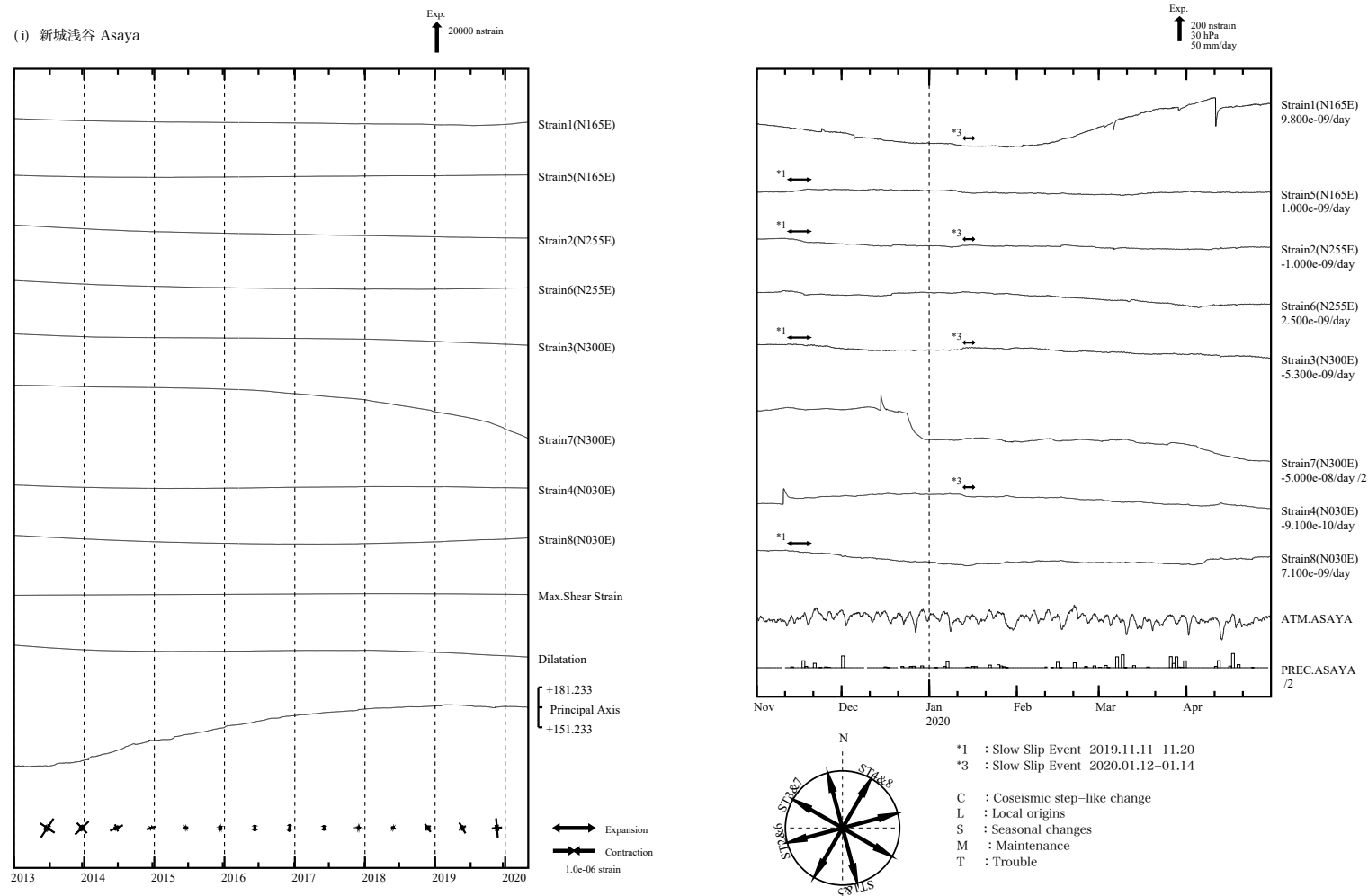
第 4 図 (e) ~ (j) 左 : 2013 年 1 月以後の多成分ひずみ計変化 (日平均値)。主ひずみ・最大せん断ひずみ・面積ひずみは各方向成分から計算されている。 右 : 2019 年 11 月 ~ 2020 年 4 月の多成分ひずみ計変化 (時間値 : 気圧・潮汐・地磁気補正した値)。各図下部に気圧変化と降水量を示す。
