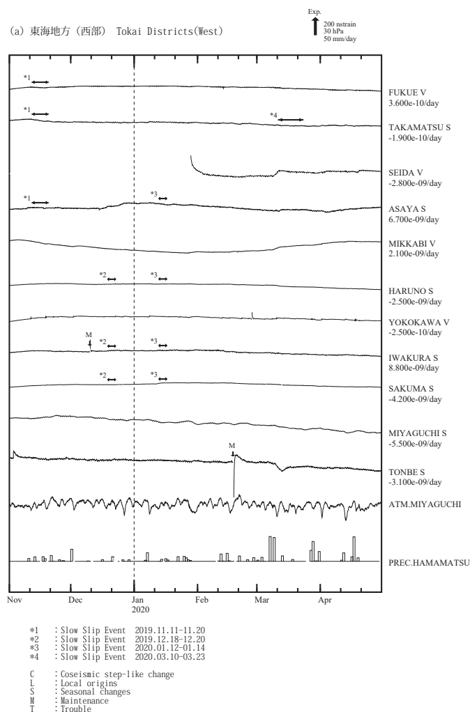
第 3 図 (a) ~ (d) 2019 年 11 月 ~ 2020 年 4 月の東海・伊豆・南関東地域における区域別体積ひずみ (V) 及び面積ひずみ (S) の変化 (時間値: 気圧・潮汐・降水補正した値). 各図下部に区域を代表する気圧変化と降水量を示す. 地点名の下に D strain/day 及び /M はそれぞれ 1 日あたりのトレンド変化量を D として補正していること及び縮尺を 1/M 倍にして表示していることを示している.
