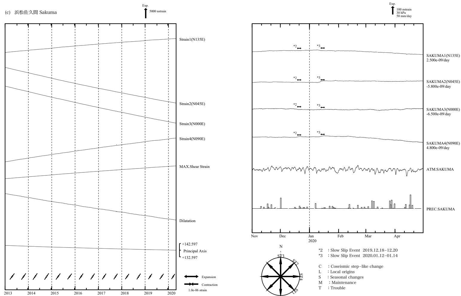
第 4 図 (a) ~ (d) 左 : 2013 年 1 月以後の多成分ひずみ計変化 (日平均値)。主ひずみ・最大せん断ひずみ・面積ひずみは各方向成分から計算されている。
