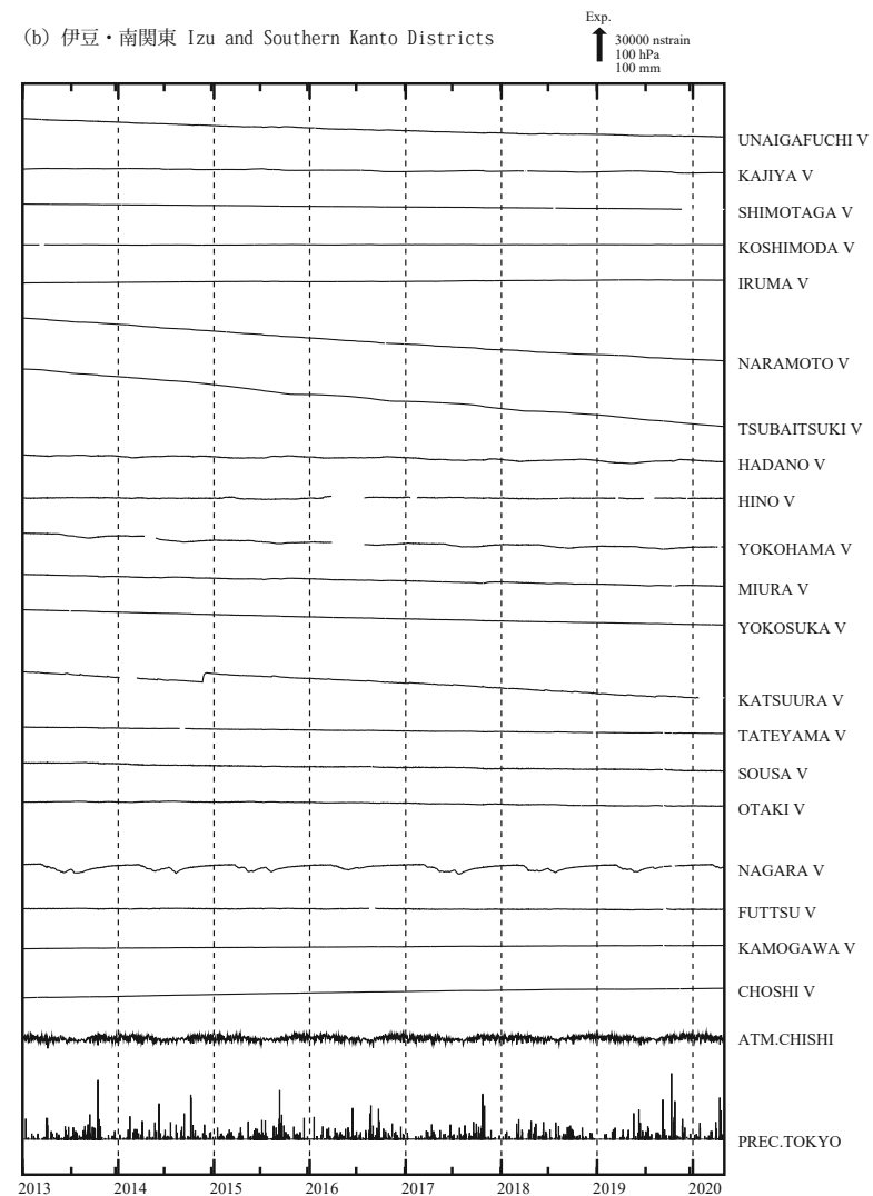
第 2 図 (a), (b) 2013 年 1 月以後の東海・伊豆・南関東地域における区域別体積ひずみ (V) 及び面積ひずみ (S) の変化 (日平均値). 各図下部に区域を代表する気圧変化と降水量を示す.
