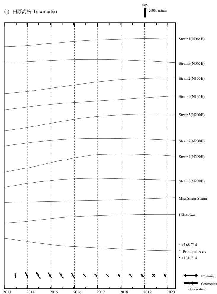
第 4 図 (c) ~ (j) 左 : 2013 年 1 月以後の多成分ひずみ計変化 (日平均値). 主ひずみ・最大せん断ひずみ・面積ひずみは各方向成分から計算されている. 右 : 2019 年 11 月 ~ 2020 年 4 月の多成分ひずみ計変化 (時間値 : 気圧・潮汐・地磁気補正した値). 各図下部に気圧変化と降水量を示す.
