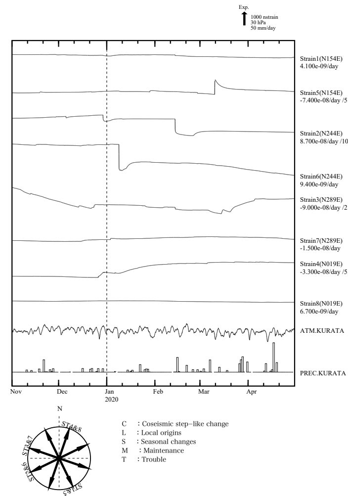
第 4 図 (c) ~ (j) 左 : 2013 年 1 月以後の多成分ひずみ計変化 (日平均値). 主ひずみ・最大せん断ひずみ・面積ひずみは各方向成分から計算されている. 右 : 2019 年 11 月 ~ 2020 年 4 月の多成分ひずみ計変化 (時間値 : 気圧・潮汐・地磁気補正した値). 各図下部に気圧変化と降水量を示す.
