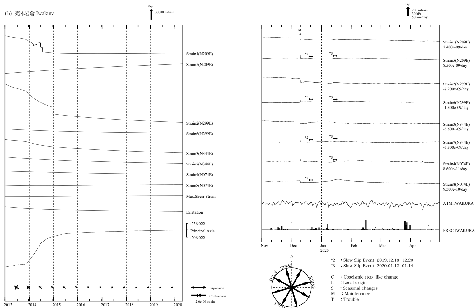
第4図(c)～(j) 左：2013年1月以後の多成分ひずみ計変化（日平均値）。主ひずみ・最大せん断ひずみ・面積ひずみは各方向成分から計算されている。 右：2019年11月～2020年4月の多成分ひずみ計変化（時間値：気圧・潮汐・地磁気補正した値）。各図下部に気圧変化と降水量を示す。
