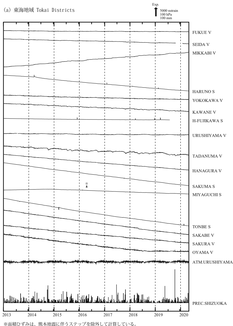
第 2 図 (a), (b) 2013 年 1 月以後の東海・伊豆・南関東地域における区域別体積ひずみ (V) 及び面積ひずみ (S) の変化 (日平均値). 各図下部に区域を代表する気圧変化と降水量を示す.
