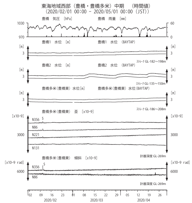
第 8 図 東海地域西部 (豊橋・豊橋多米) の地下水等の観測結果 (2020 年 2 月～2020 年 4 月)
