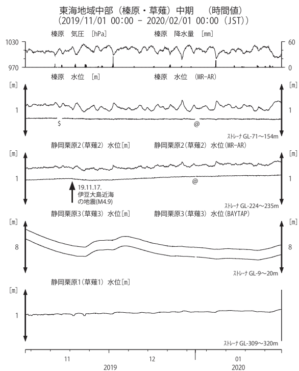
第 3 図 東海地域中部の地下水等の観測結果 (2019 年 11 月～2020 年 1 月)
