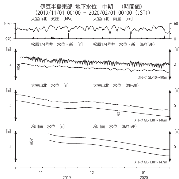
第 11 図 伊豆半島東部の地下水等の観測結果（2019 年 11 月～2020 年 1 月）
