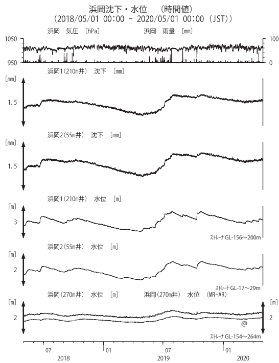
第 21 図 浜岡における沈下等の観測結果（2018 年 5 月～2020 年 4 月）
