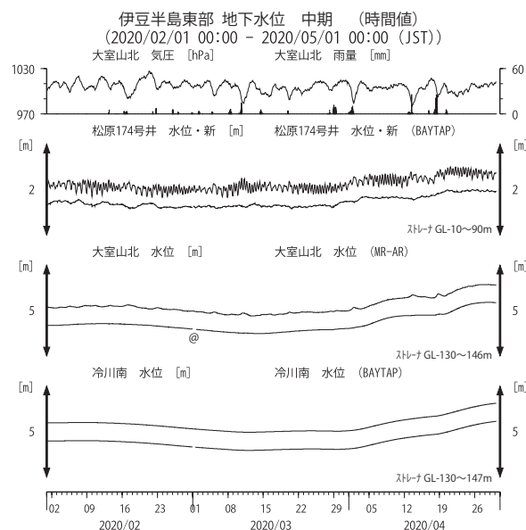
第 12 図 伊豆半島東部の地下水等の観測結果（2020 年 2 月～2020 年 4 月）
