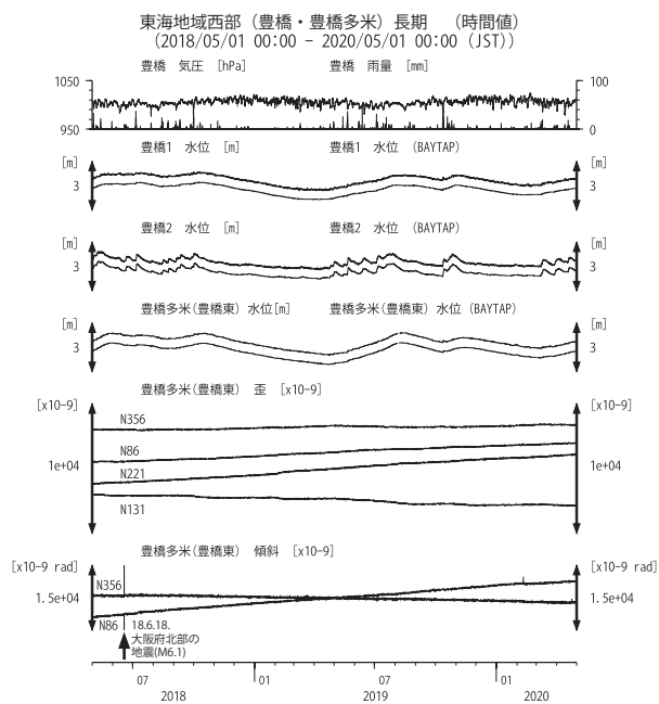
第 17 図 東海地域西部（豊橋・豊橋多米）の地下水等の観測結果（2018 年 5 月～2020 年 4 月）
