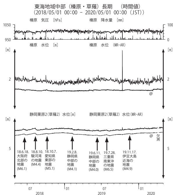
第 15 図 東海地域中部の地下水等の観測結果 (2018 年 5 月～2020 年 4 月)
