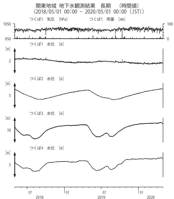
第 20 図 関東地域の地下水等の観測結果（2018 年 5 月～2020 年 4 月）
