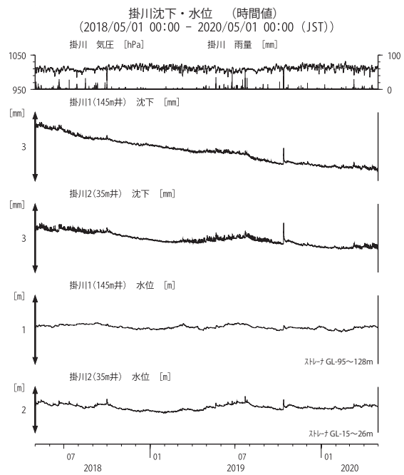
第 22 図 掛川における沈下等の観測結果（2018 年 5 月～2020 年 4 月）
