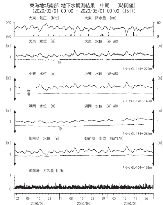
第 6 図 東海地域南部の地下水等の観測結果 (2020 年 2 月～2020 年 4 月)
