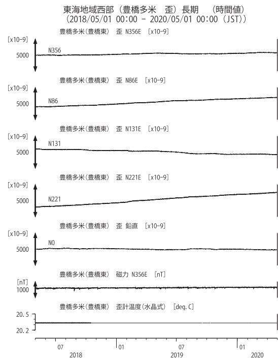
第 18 図 東海地域西部（豊橋多米）の歪等の観測結果（2018 年 5 月～2020 年 4 月）
