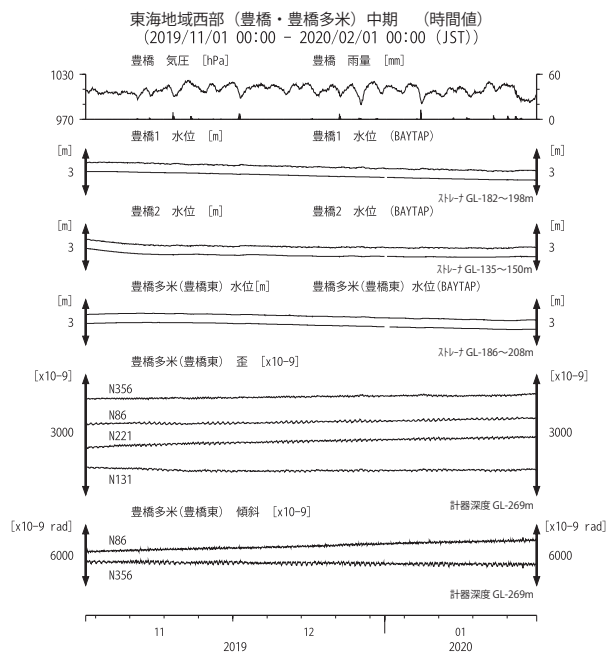
第 7 図 東海地域西部 (豊橋・豊橋多米) の地下水等の観測結果 (2019 年 11 月～2020 年 1 月)
