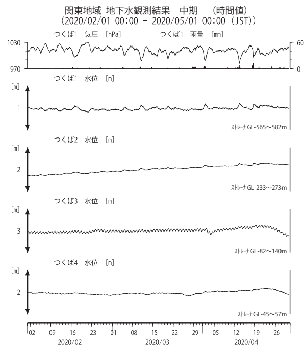
第 14 図 関東地域の地下水等の観測結果 (2020 年 2 月～2020 年 4 月)
