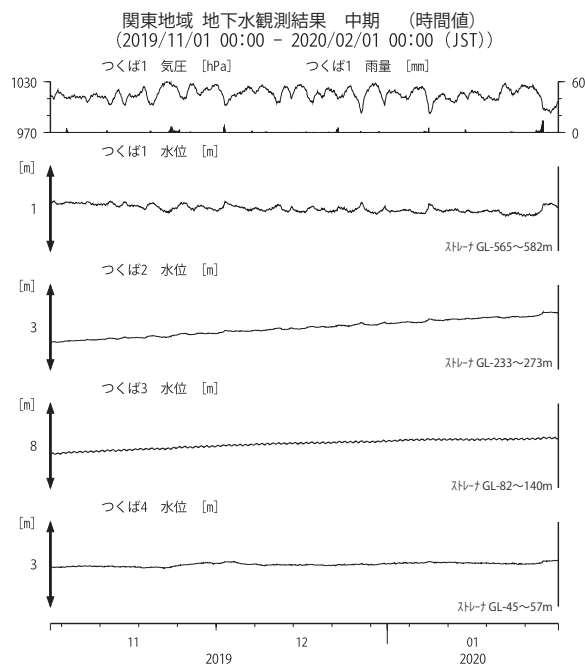
第 13 図 関東地域の地下水等の観測結果 (2019 年 11 月～2020 年 1 月)
