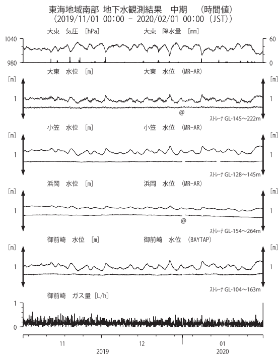
第 5 図 東海地域南部の地下水等の観測結果 (2019 年 11 月～2020 年 1 月)
