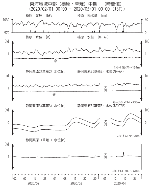
第 4 図 東海地域中部の地下水等の観測結果 (2020 年 2 月～2020 年 4 月)
