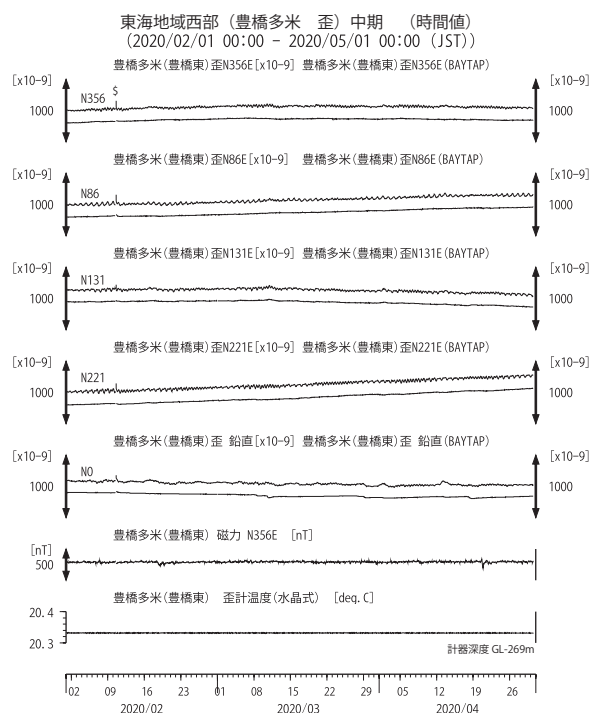
第10図 東海地域西部（豊橋多米）の歪等の観測結果 (2020年2月～2020年4月)
