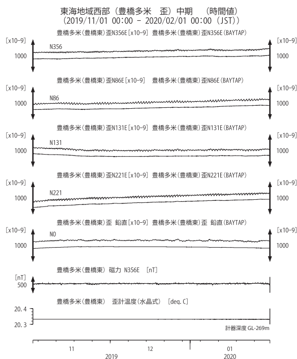
第9図 東海地域西部（豊橋多米）の歪等の観測結果 (2019年11月～2020年1月)
