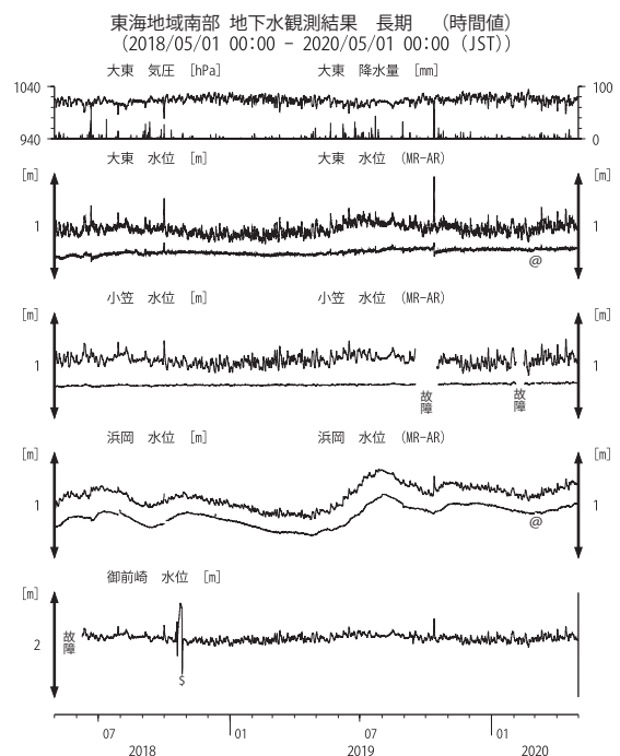
第 16 図 東海地域南部の地下水等の観測結果 (2018 年 5 月～2020 年 4 月)
