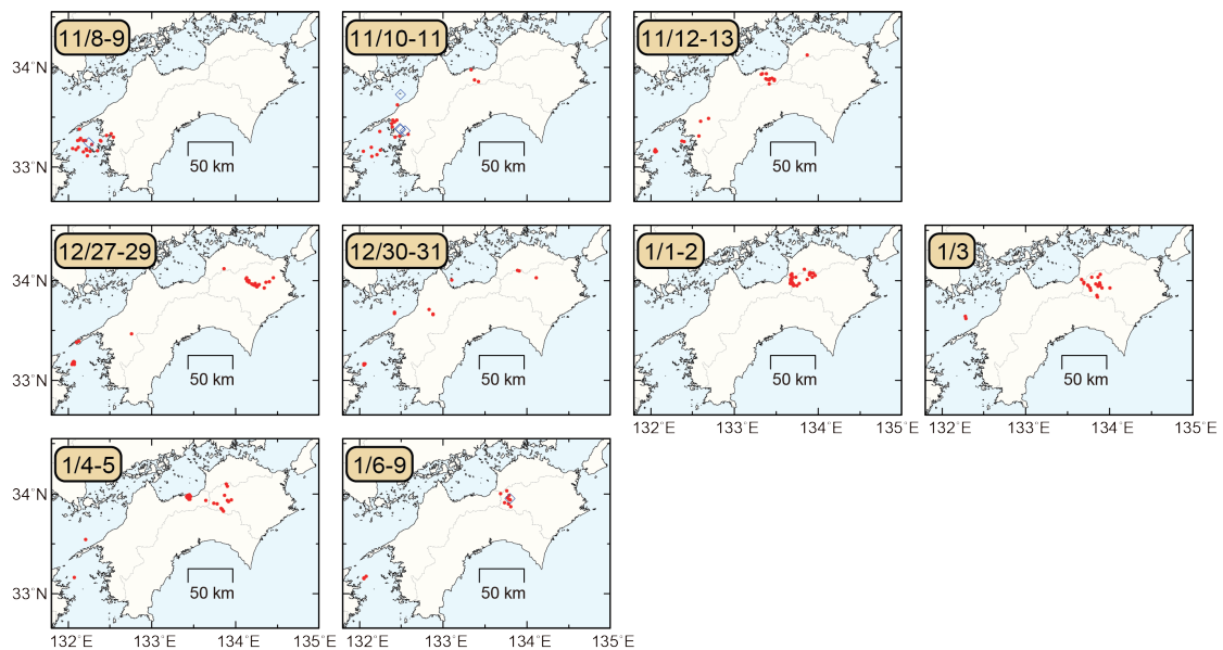
第 5 図 2019 年 11 月から 2020 年 1 月までの期間に四国地域で発生した、主な深部低周波微動及び超低周波地震の活動における震央分布スナップショット。赤丸が当該期間の微動、青菱形が超低周波地震を表す。
