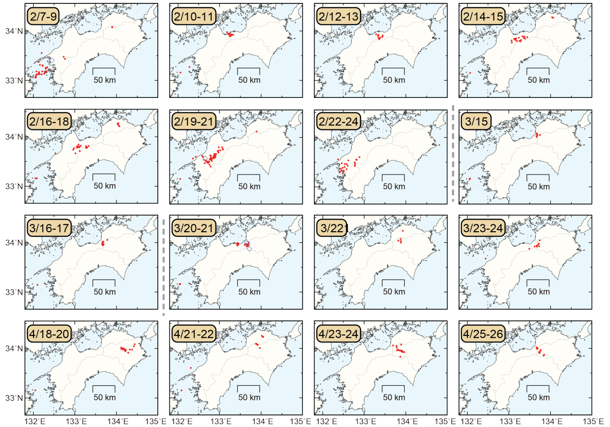
第 6 図 2020 年 2 月から 2020 年 4 月までの期間に四国地域で発生した、主な深部低周波微動及び超低周波地震の活動における震央分布スナップショット。赤丸が当該期間の微動、青菱形が超低周波地震を表す。
