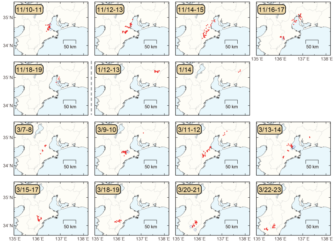
第 4 図 2019 年 11 月から 2020 年 3 月までの期間に東海・紀伊半島地域で発生した、主な深部低周波微動及び深部超低周波地震の活動における震央分布スナップショット。赤丸が当該期間の微動、青菱形が超低周波地震を表す。
